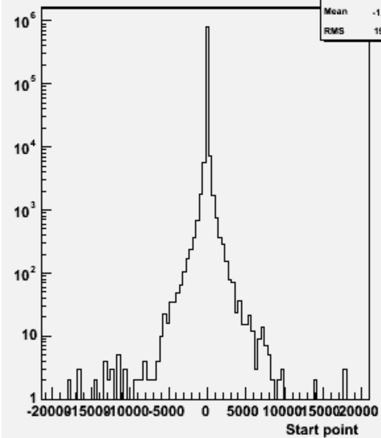
Start point Z : w101160 ssude2n2_o
