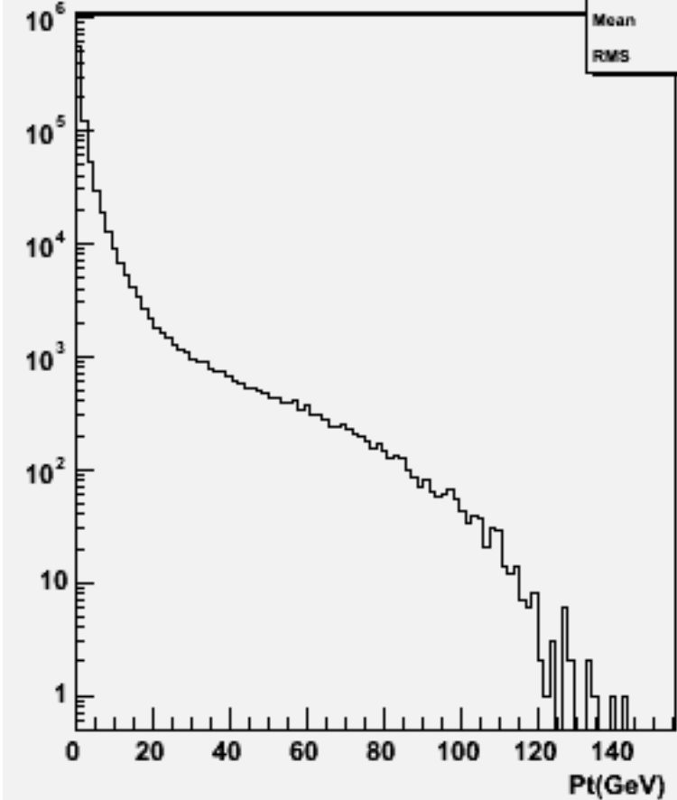
Particle Pt : w101160 ssude2n2_o
