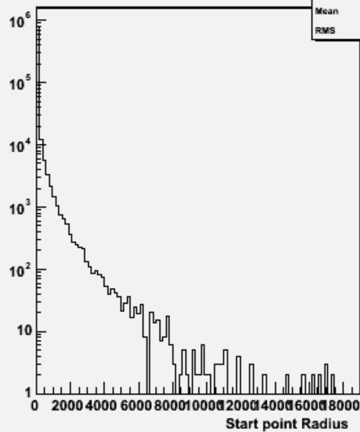
Start point R : w101160 ssude2n2_o
