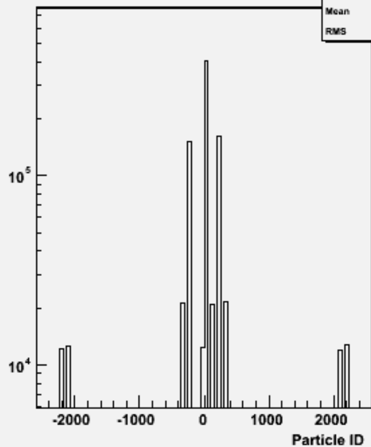
Particle ID : w101160 ssude2n2_o
