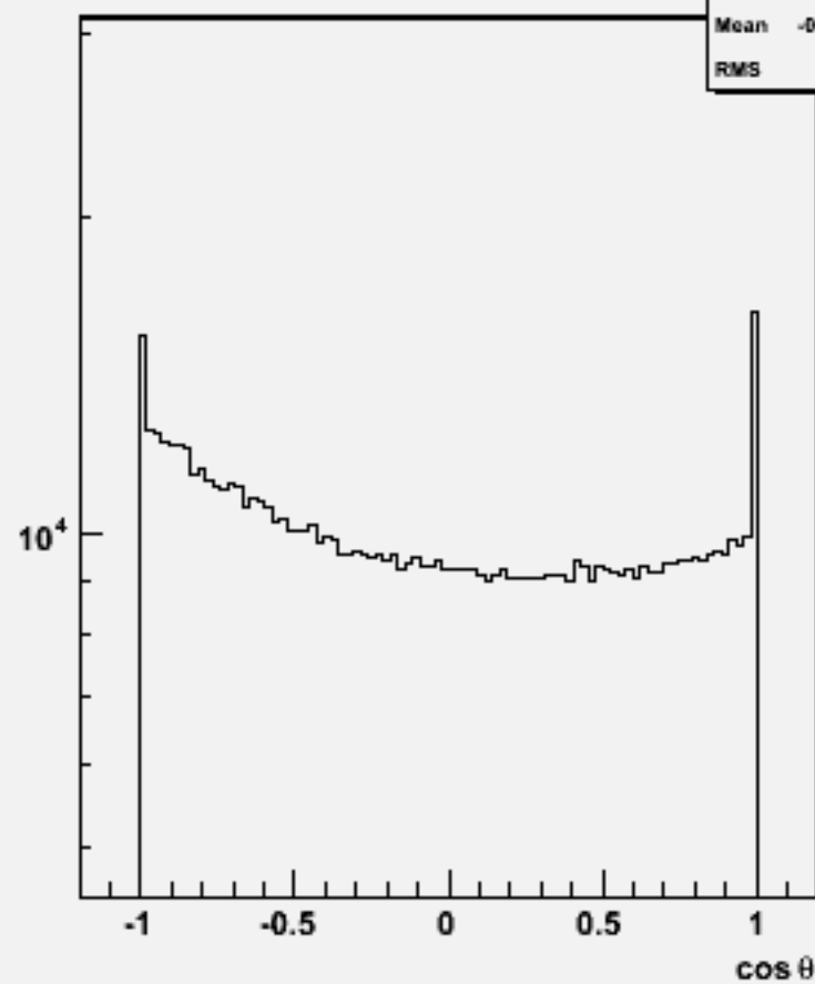
Particle cos \theta : w101160 ssude2n2_o
