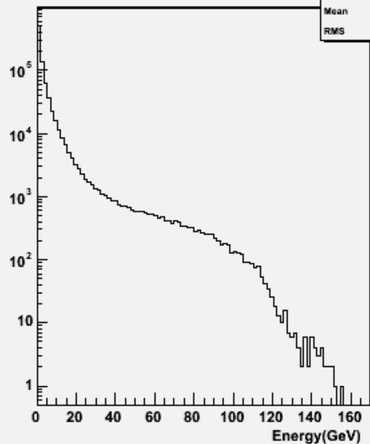
Particle Energy : w101160 ssude2n2_o
