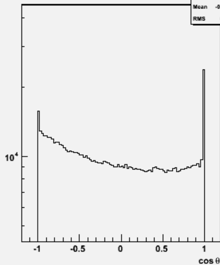
Particle cos \theta : w101156 ssude1n1_o
