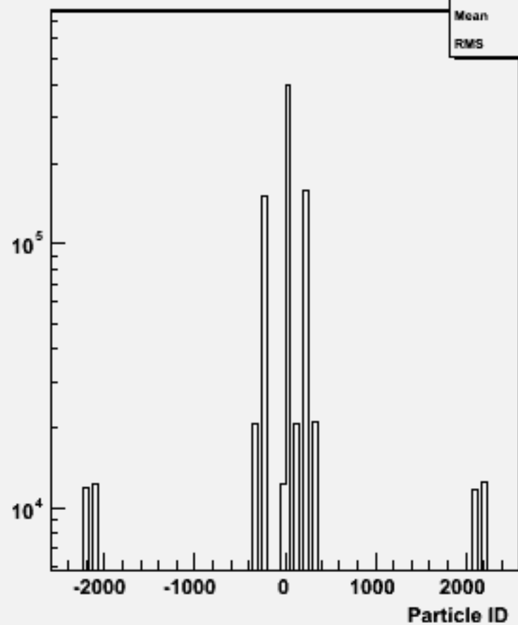
Particle ID : w101156 ssude1n1_o
