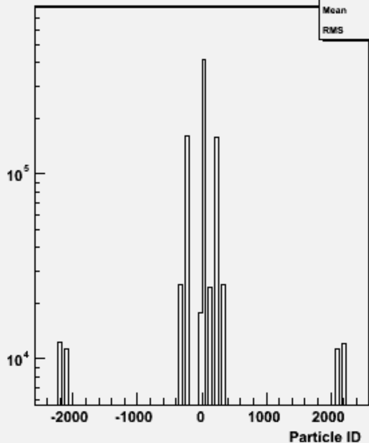
Particle ID : w101152 ssn3e3sc_o
