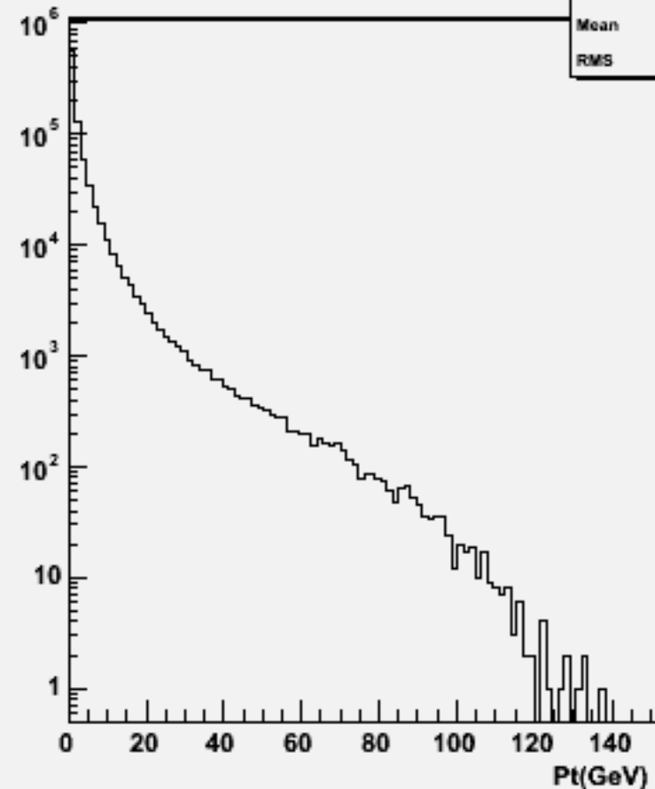
Particle Pt : w101152 ssn3e3sc_o
