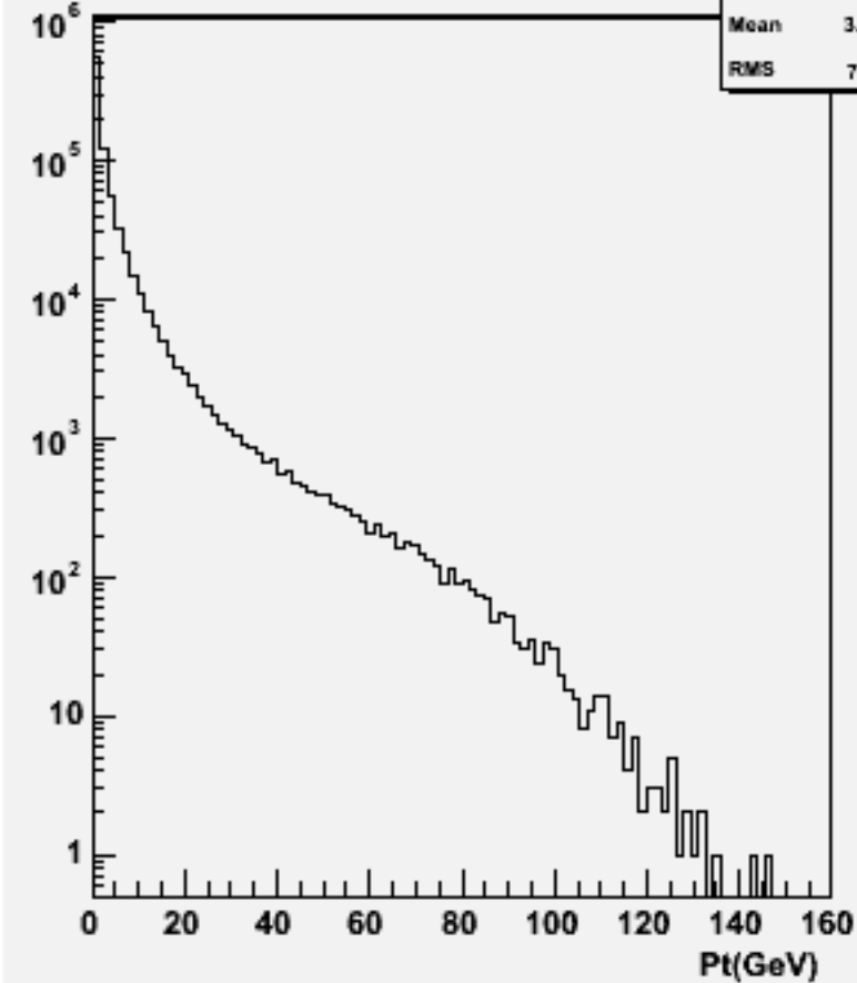
Particle Pt : w101149 ssn3e3du_o
