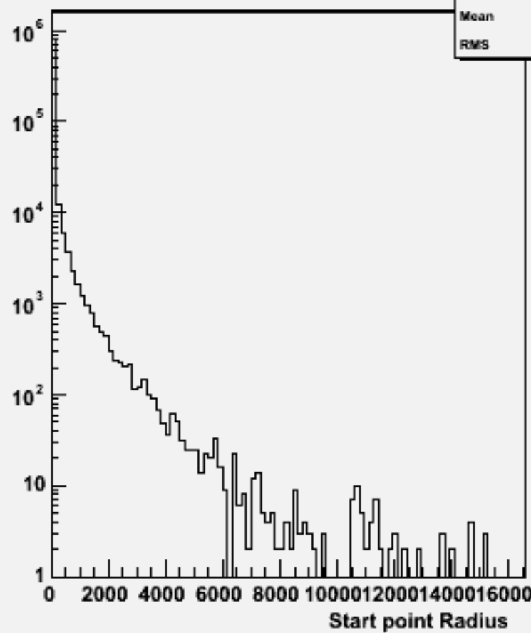
Start point R : w101149 ssn3e3du_o
