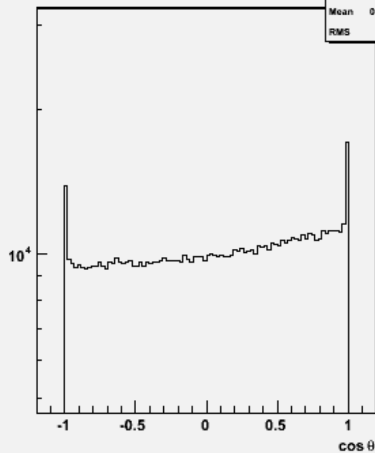
Particle cos \theta : w101149 ssn3e3du_o
