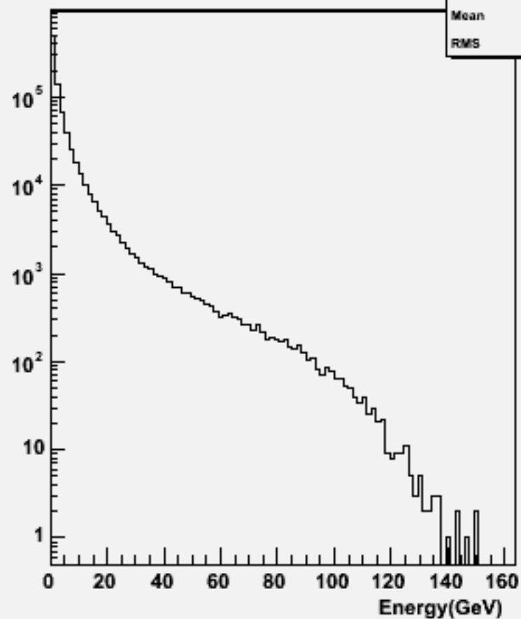
Particle Energy : w101149 ssn3e3du_o
