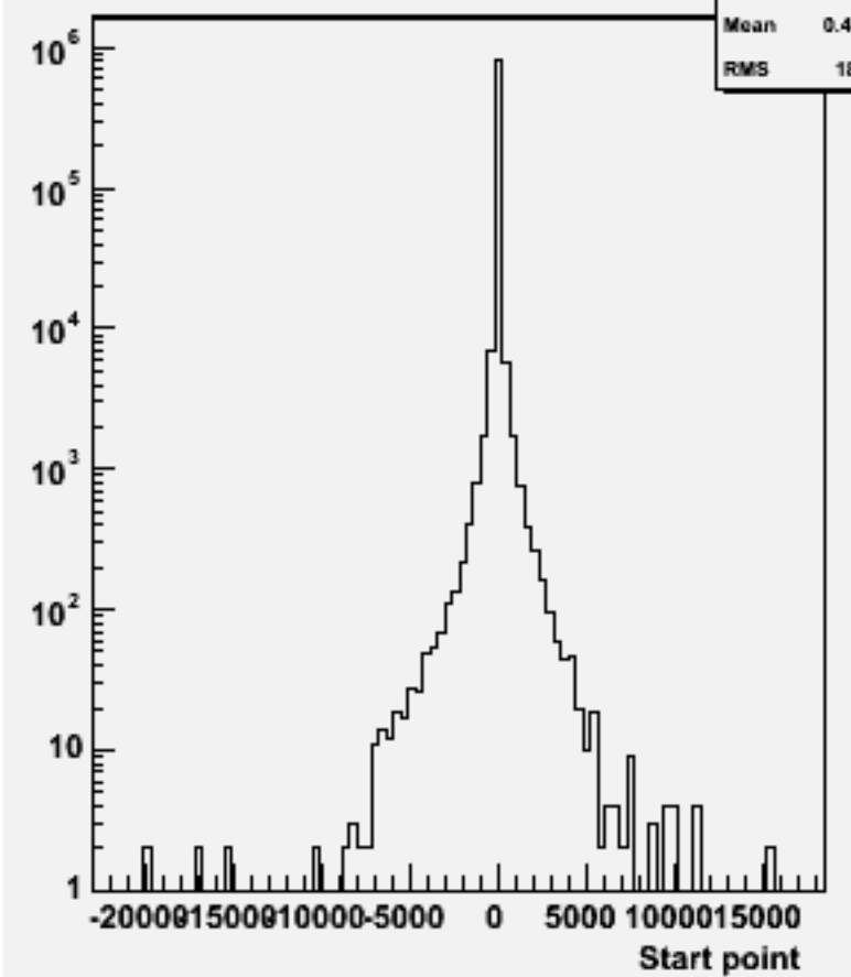
Start point Z : w101149 ssn3e3du_o
