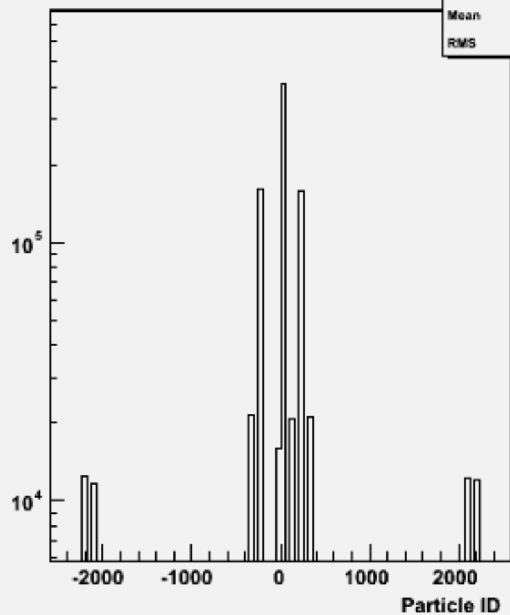
Particle ID : w101149 ssn3e3du_o
