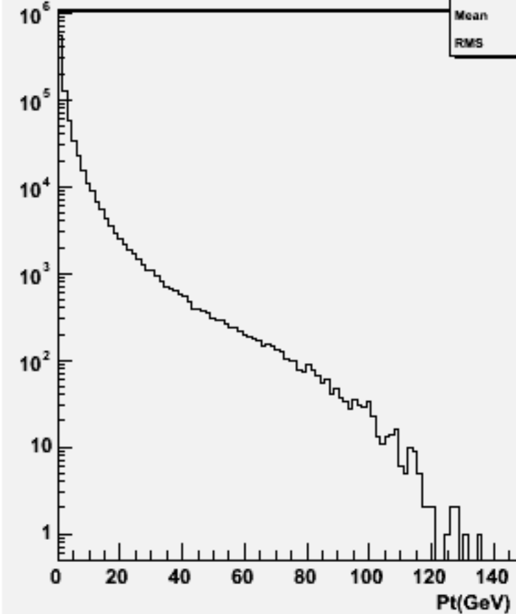
Particle Pt : w101148 ssn3e3du_o
