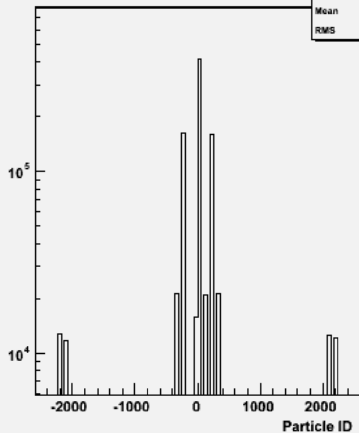
Particle ID : w101148 ssn3e3du_o
