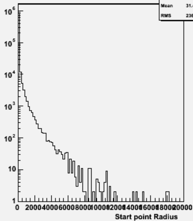
Start point R : w101148 ssn3e3du_o
