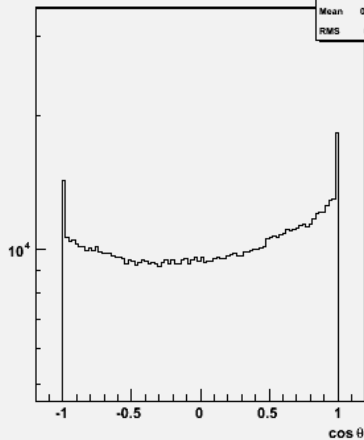
Particle cos \theta : w101148 ssn3e3du_o
