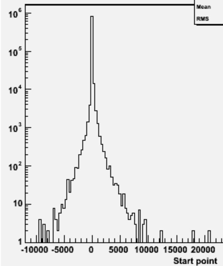
Start point Z : w101148 ssn3e3du_o
