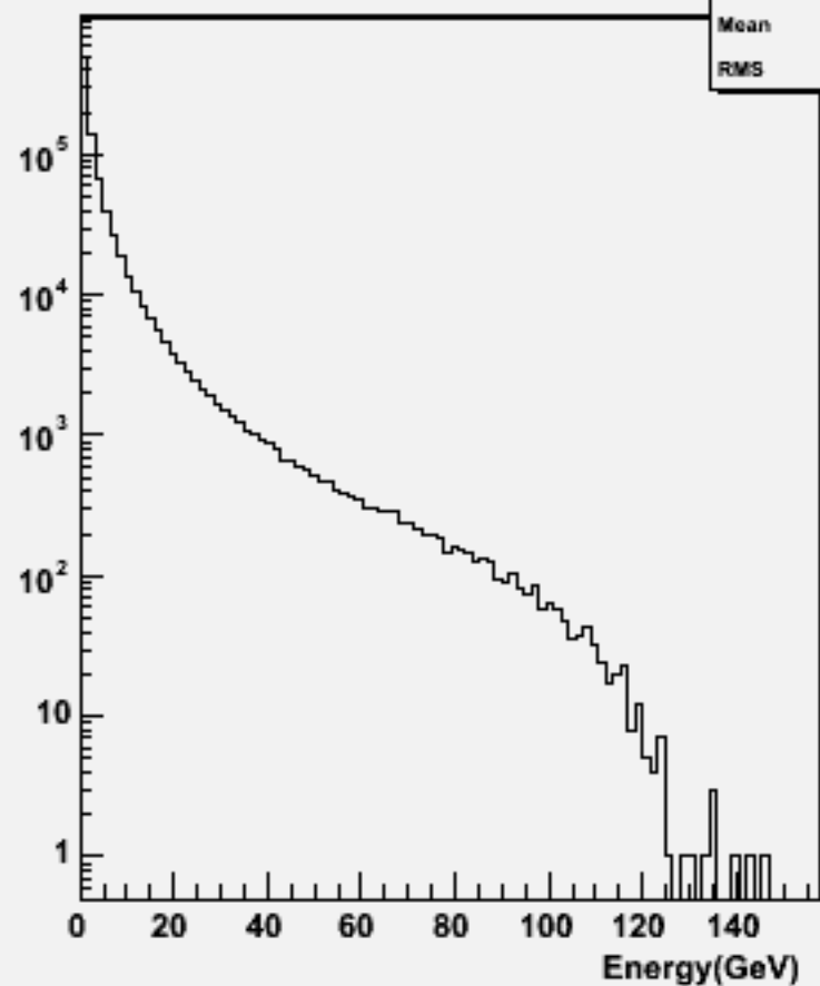
Particle Energy : w101148 ssn3e3du_o
