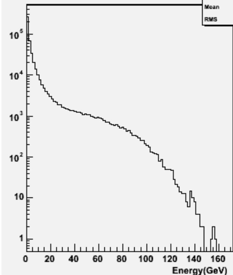
Start point R : w101141 ssn3e3e2n2_o
