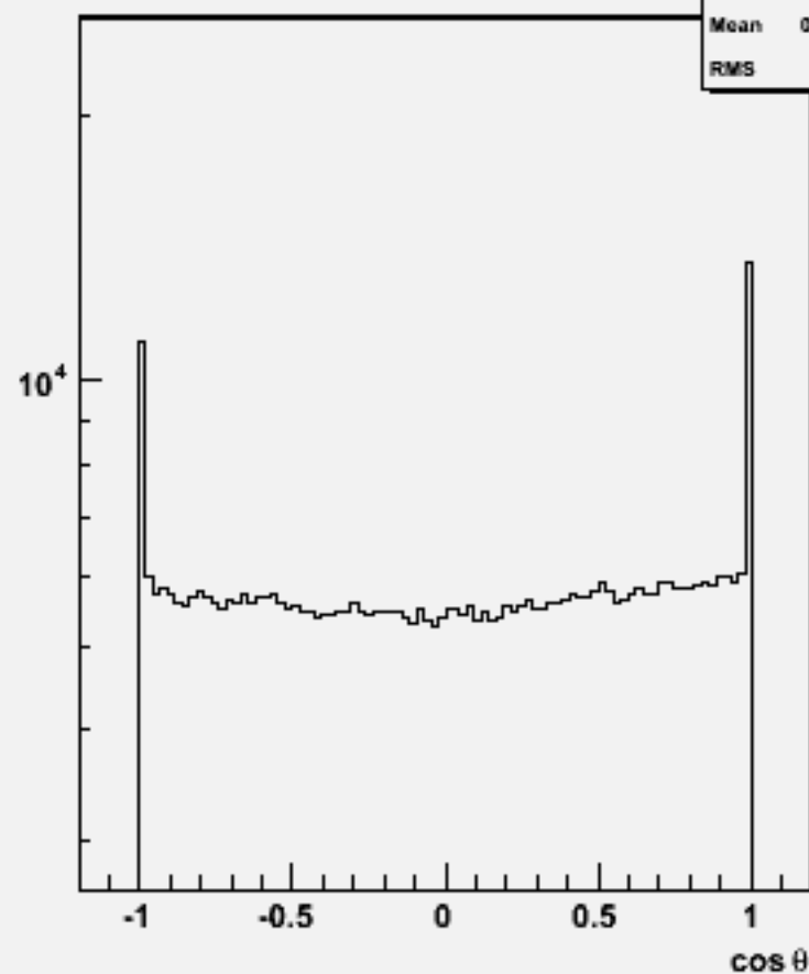
Particle cosθ : w101141 ssn3e3e2n2_o
