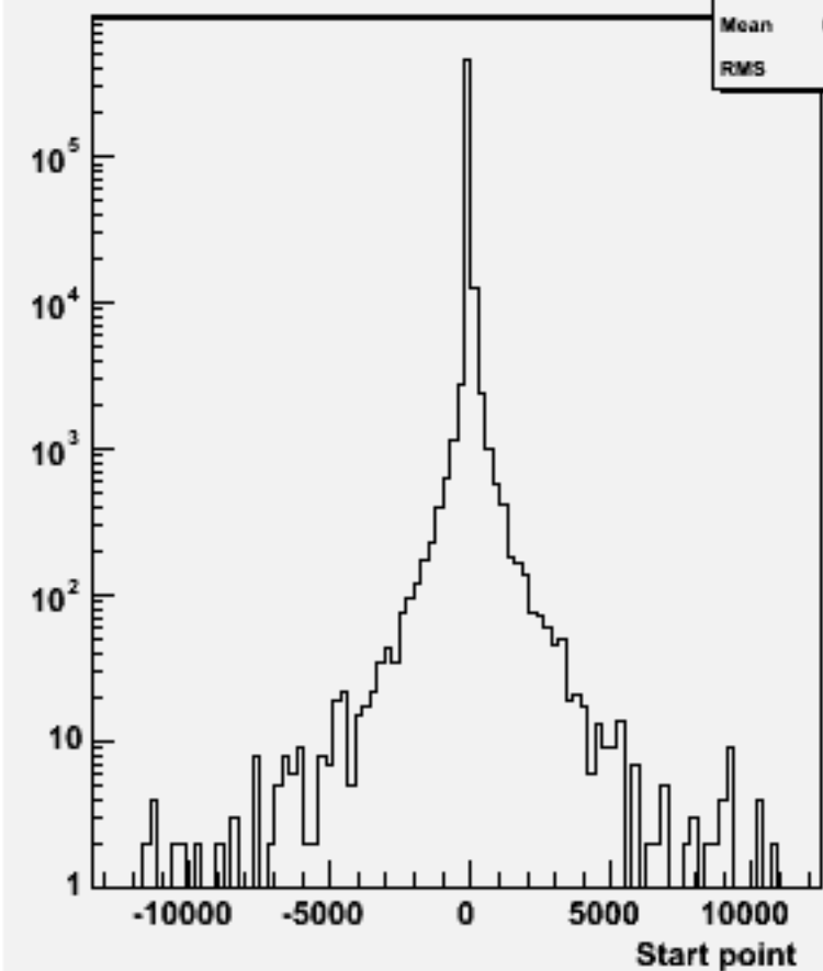
Start point Z : w101141 ssn3e3e2n2_o
