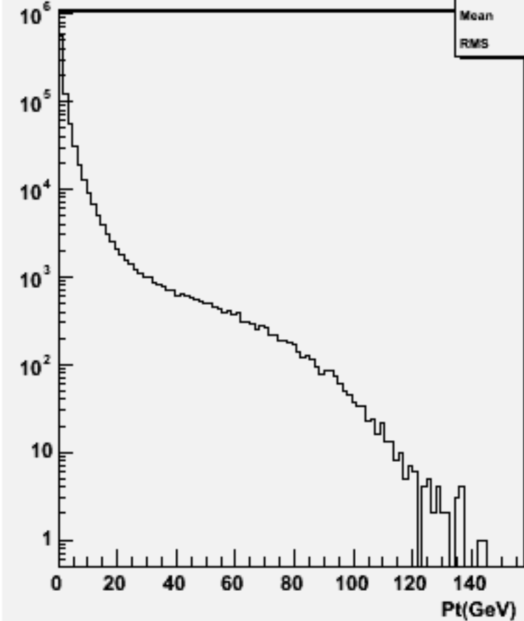
Particle Pt : w101133 ssn2e2sc_o
