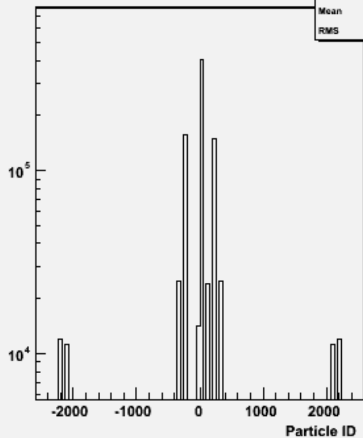
Particle ID : w101133 ssn2e2sc_o
