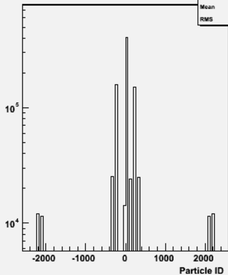
Particle ID : w101132 ssn2e2sc_o
