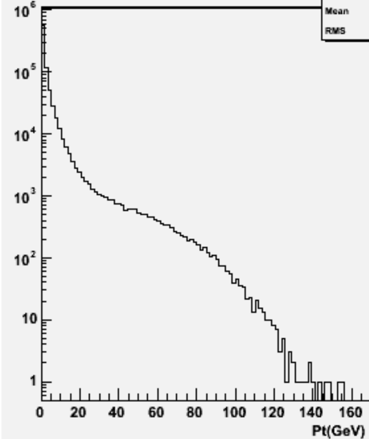
Particle Pt : w101129 ssn2e2du_o
