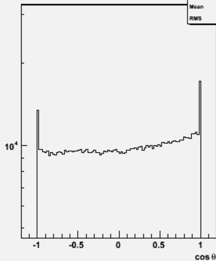
Particle cos \theta : w101129 ssn2e2du_o
