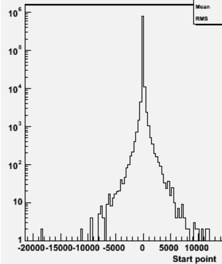
Start point Z : w101129 ssn2e2du_o
