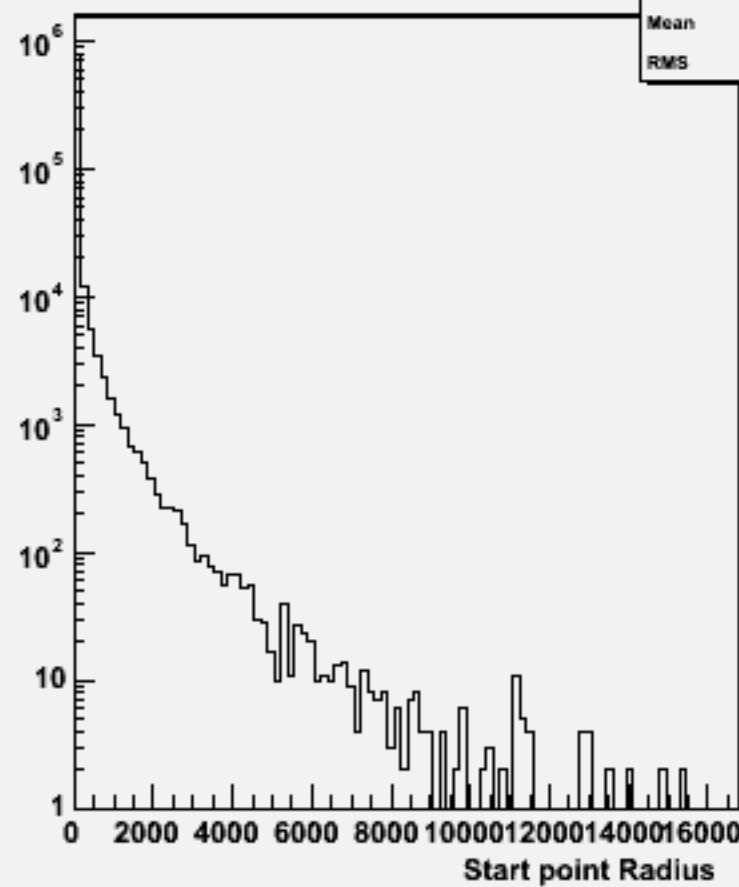
Start point R : w101129 ssn2e2du_o
