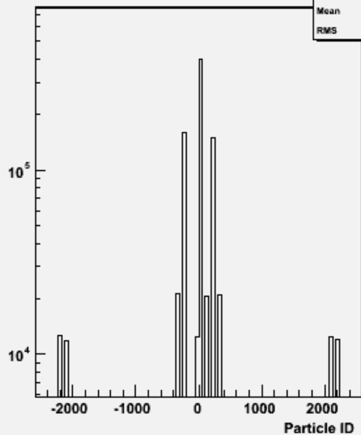
Particle ID : w101129 ssn2e2du_o
