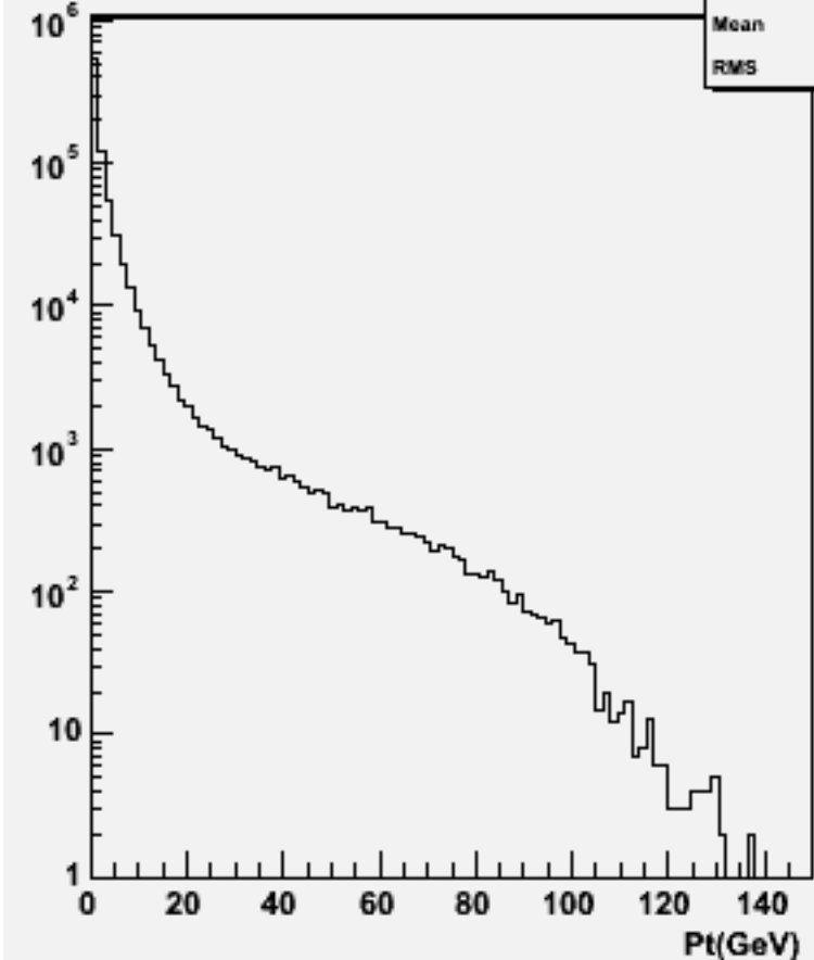
Particle Pt : w101128 ssn2e2du_o
