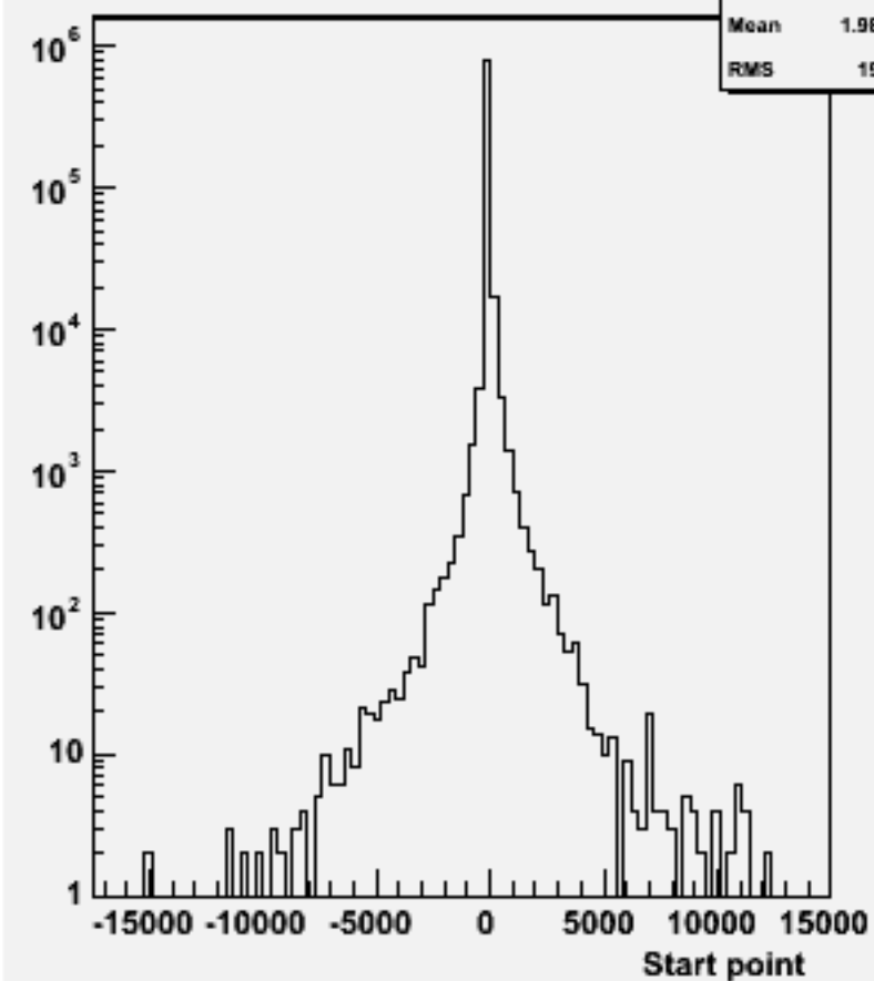
Start point Z : w101128 ssn2e2du_o
