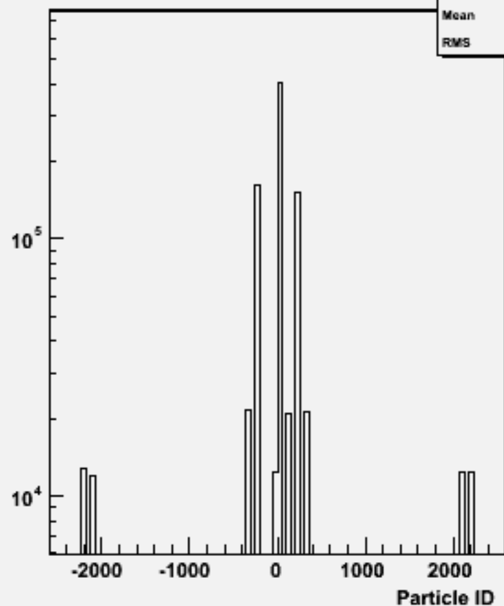
Particle ID : w101128 ssn2e2du_o
