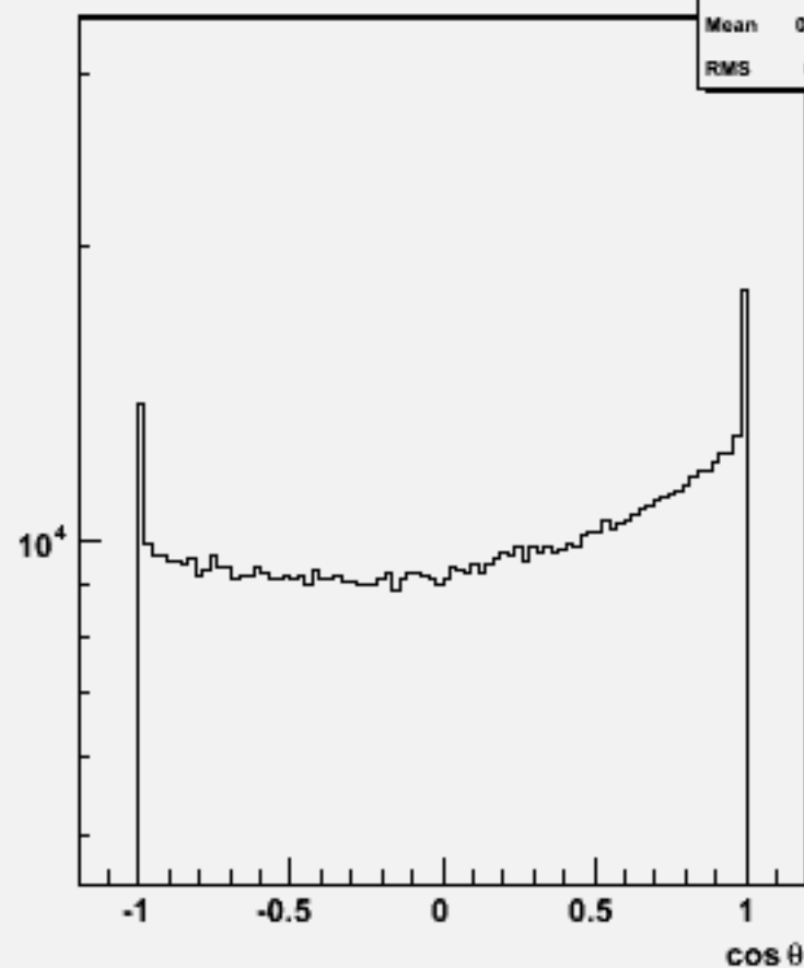
Particle cos \theta : w101128 ssn2e2du_o
