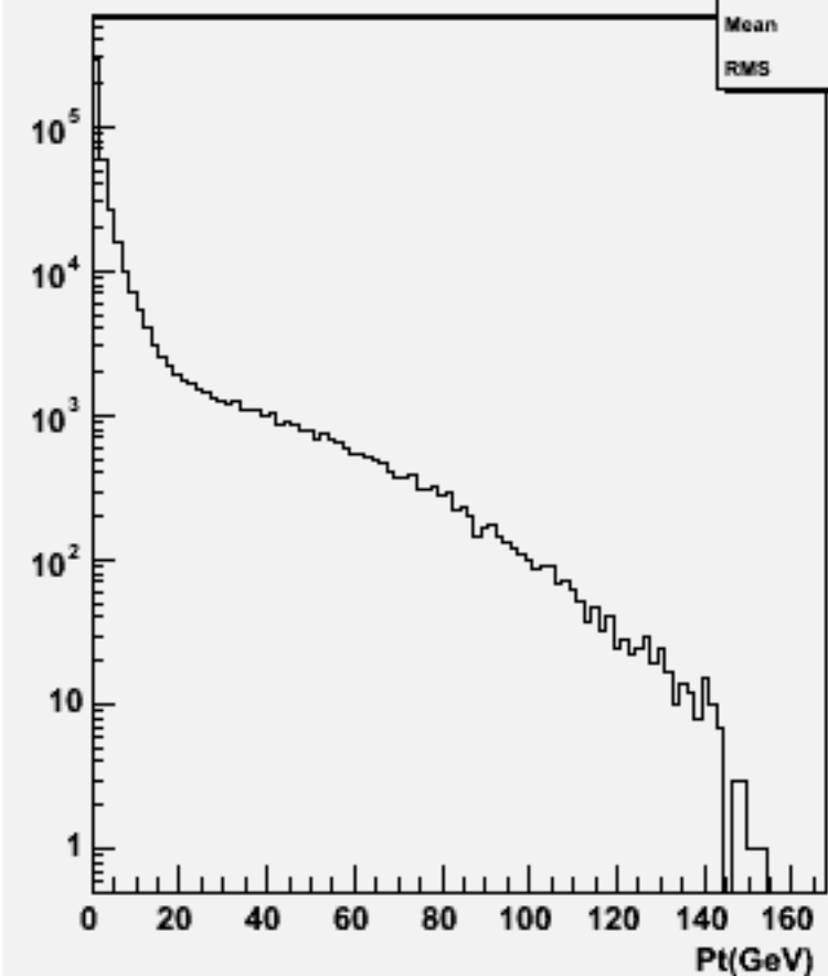
Particle Pt : w101121 ssn2e2e2n2_o
