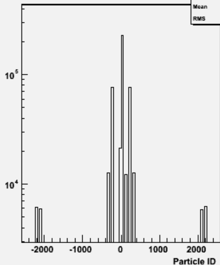
Particle ID : w101121 ssn2e2e2n2_o
