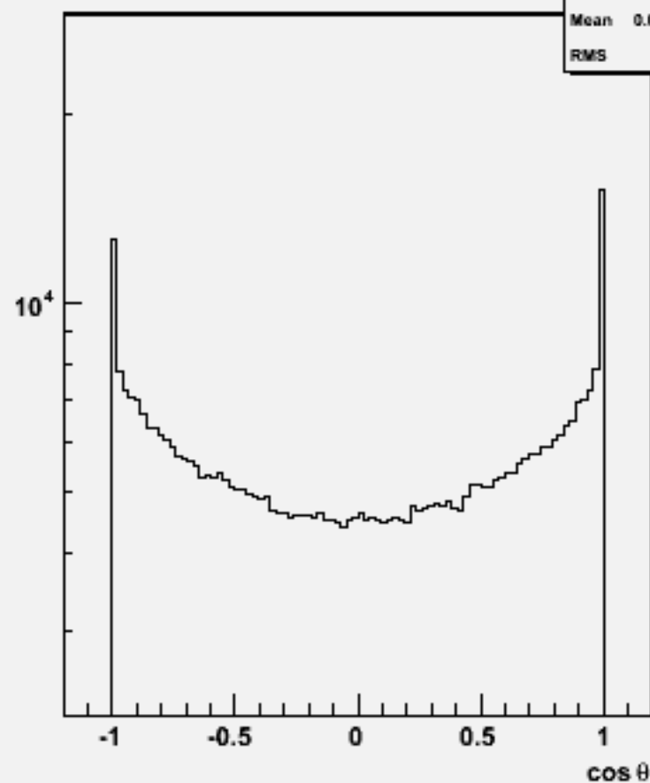
Particle cosθ : w101121 ssn2e2e2n2_o
