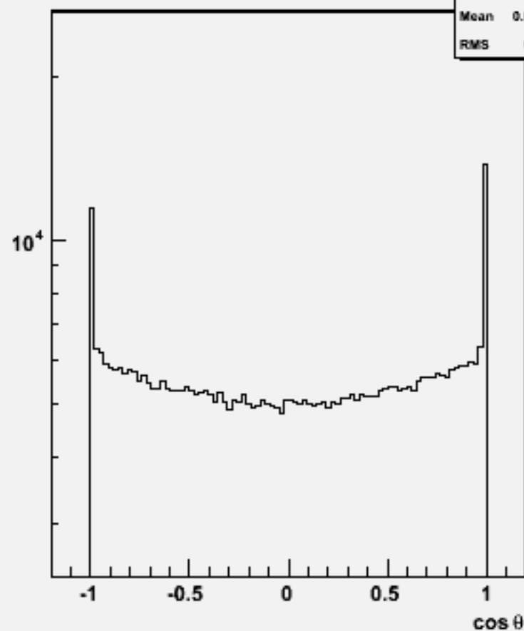
Particle \cos\theta : w101120 ssn2e2e2n2_o
