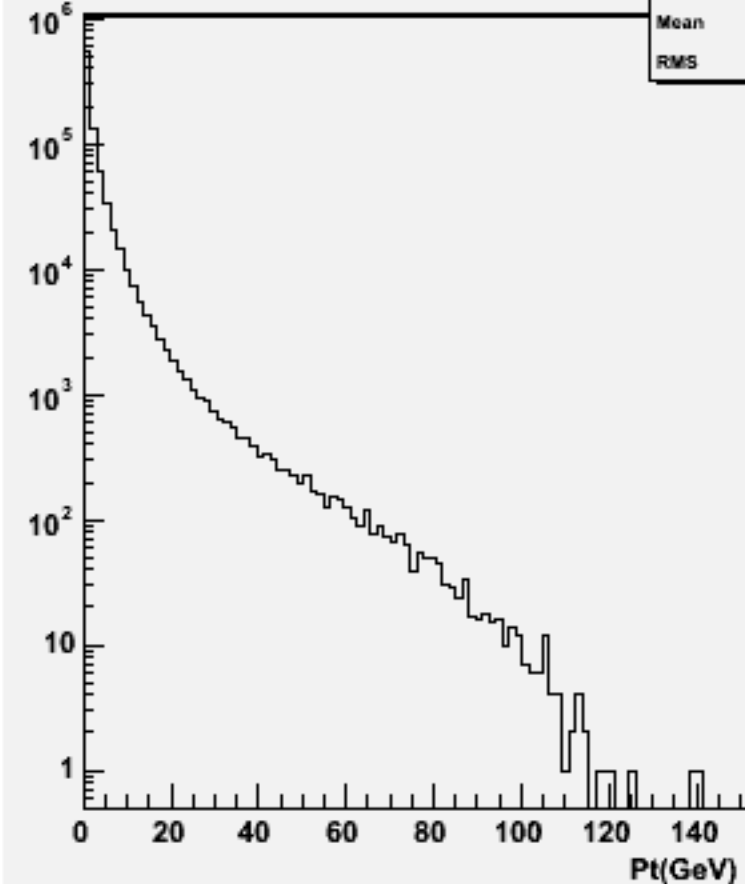
Particle Pt : w101112 ssn1e1sc_o
