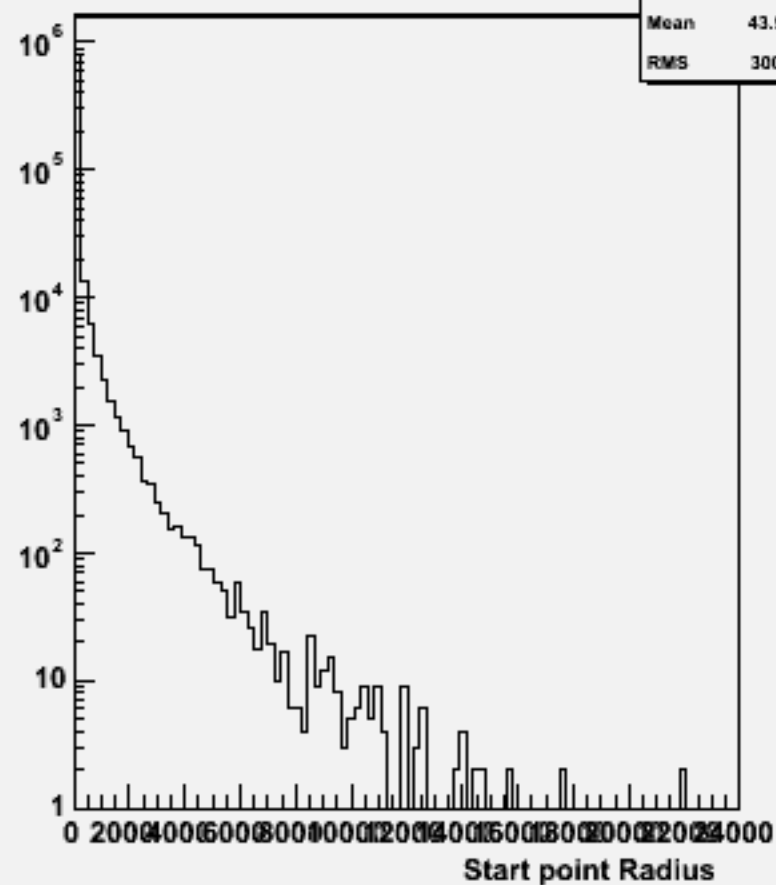
Start point R : w101112 ssn1e1sc_o
