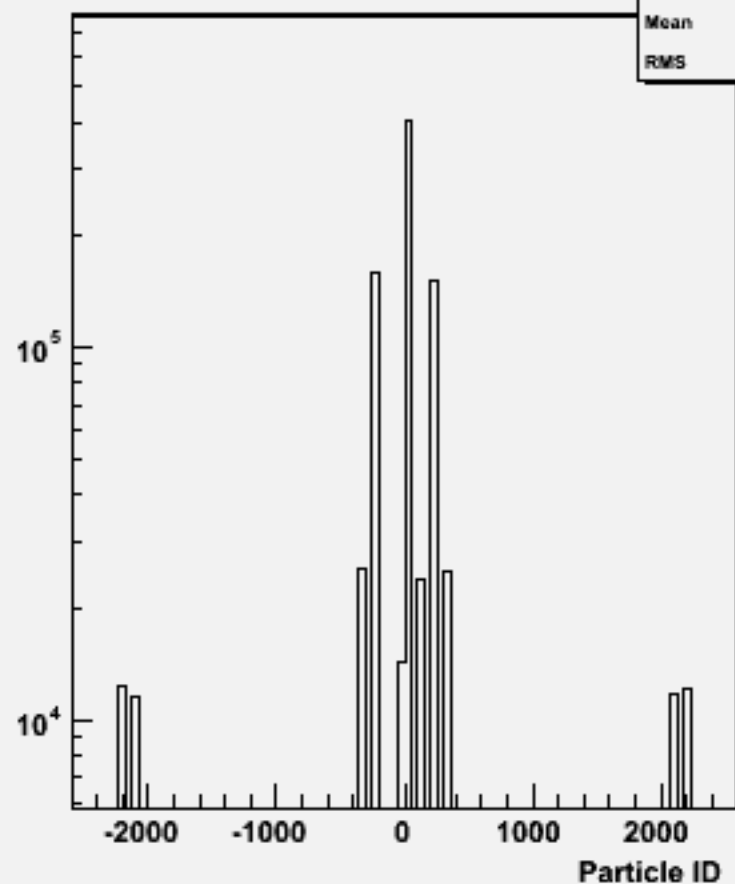
Particle ID : w101112 ssn1e1sc_o
