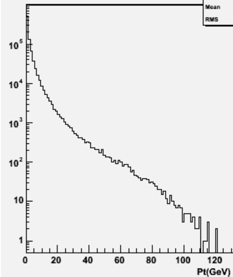
Particle Pt : w101111 ssn1e1sc_o
