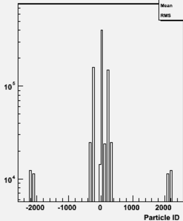
Particle ID : w101111 ssn1e1sc_o
