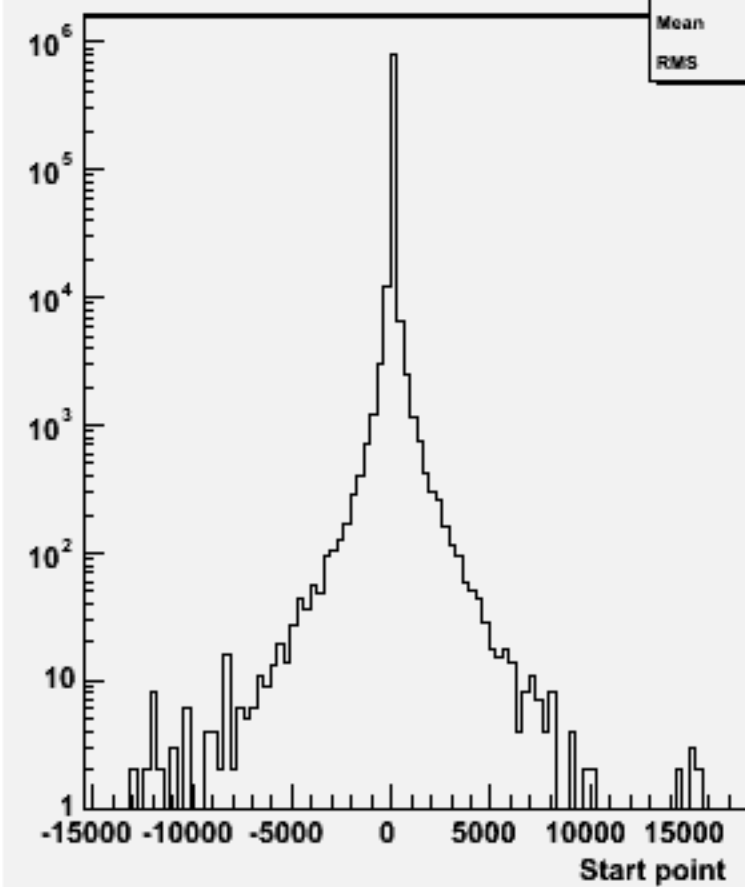
Start point Z : w101111 ssn1e1sc_o
