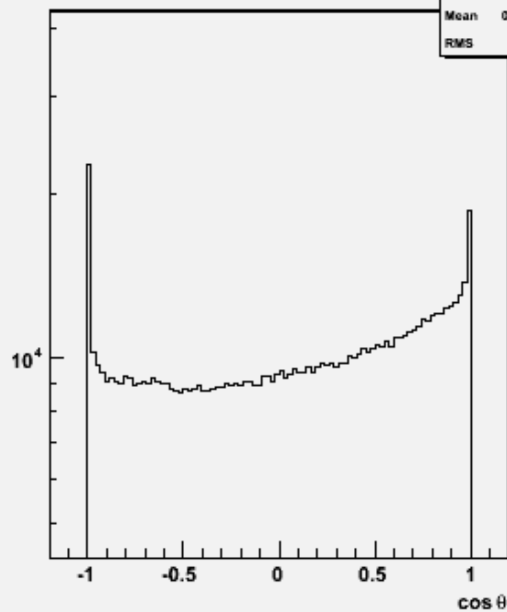
Particle cosθ : w101111 ssn1e1sc_o
