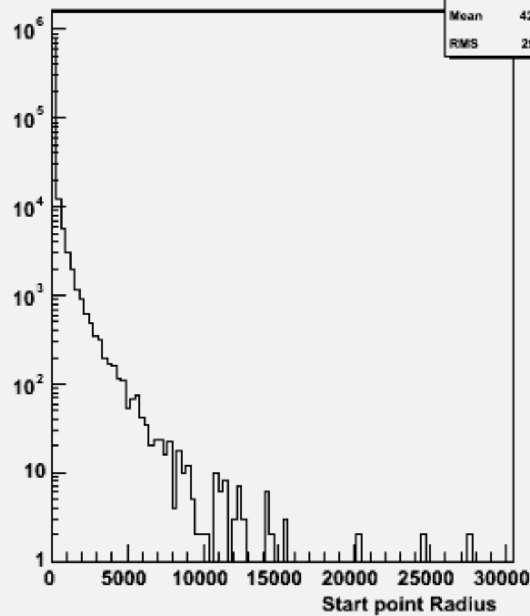
Start point R : w101111 ssn1e1sc_o
