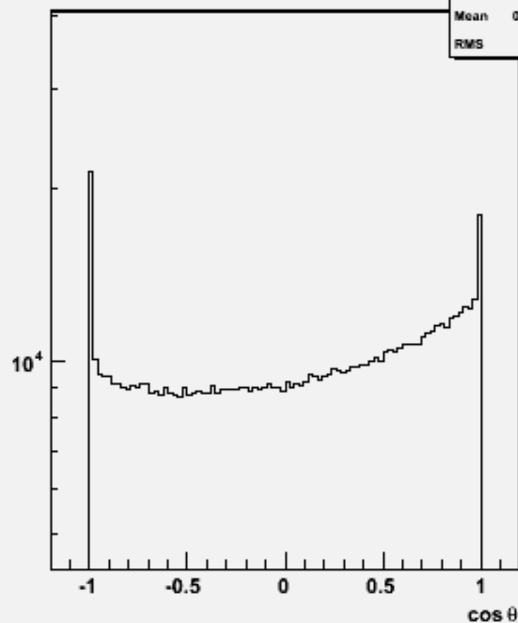
Particle cos \theta : w101108 ssn1e1du_o
