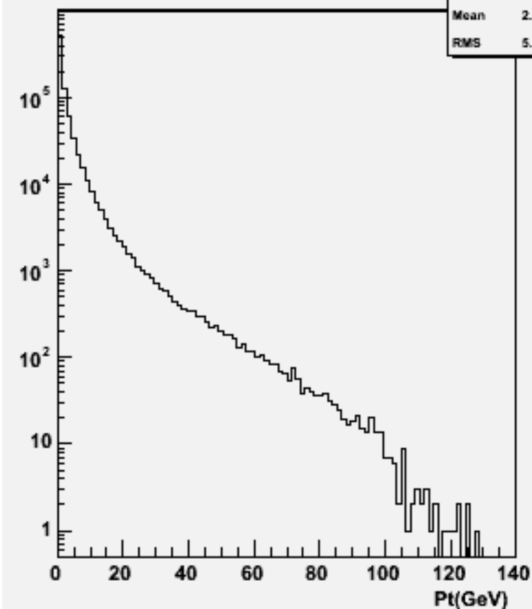
Particle Pt : w101108 ssn1e1du_o
