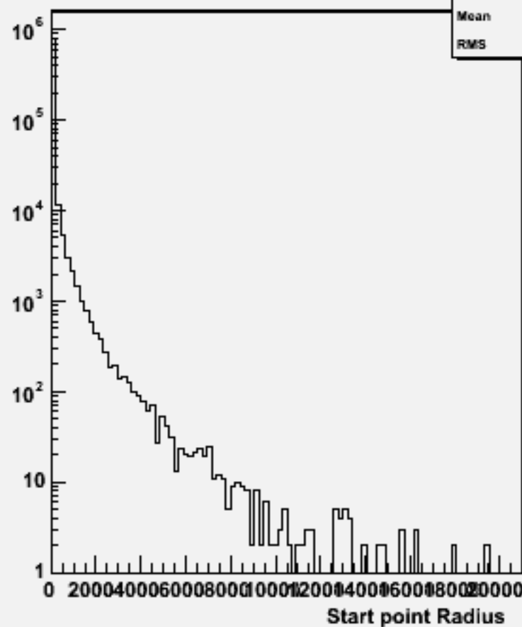
Start point R : w101108 ssn1e1du_o
