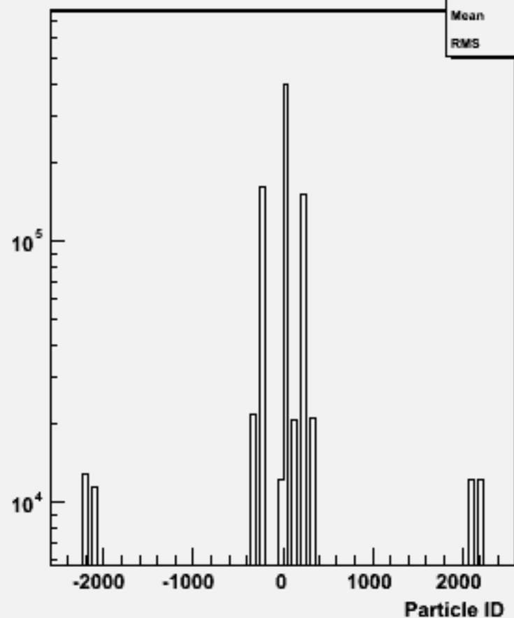
Particle ID : w101108 ssn1e1du_o
