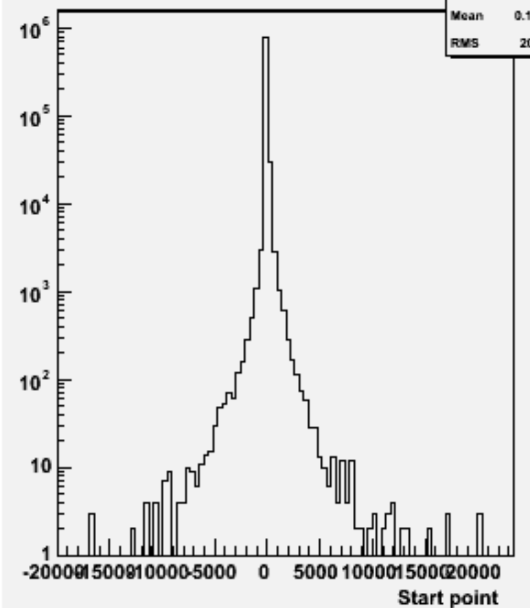
Start point Z : w101108 ssn1e1du_o
