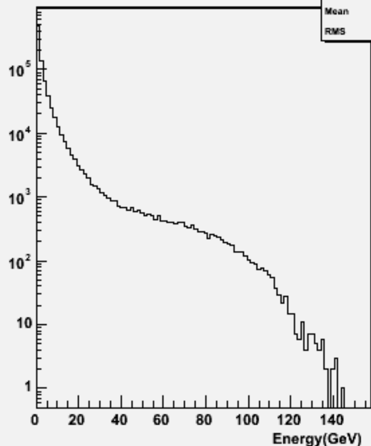
Particle Energy : w101108 ssn1e1du_o
