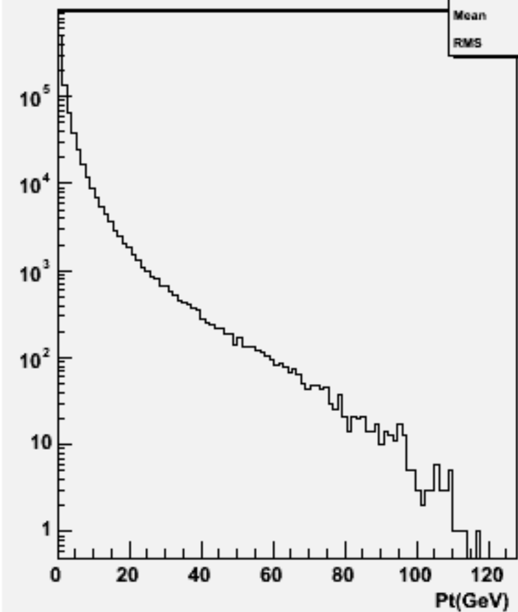
Particle Pt : w101107 ssn1e1du_o
