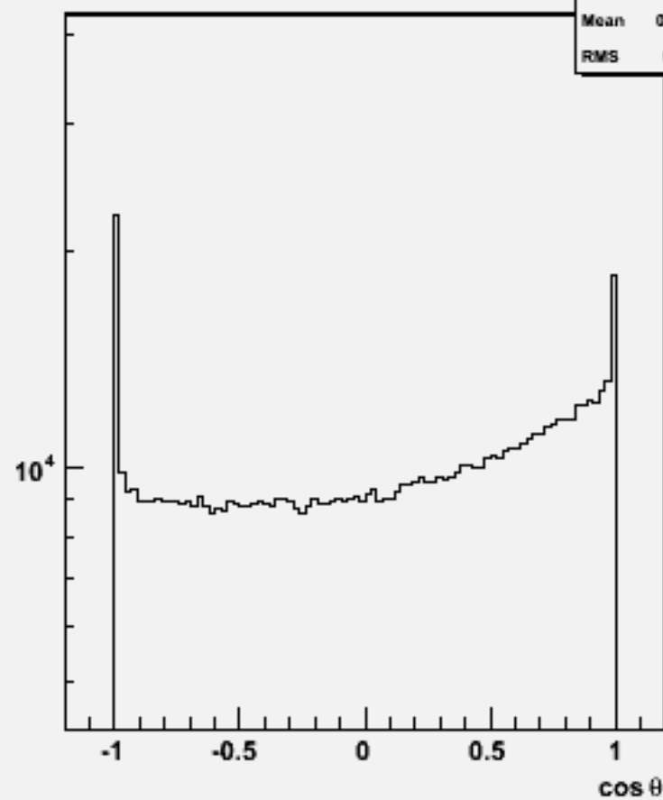
Particle cos \theta : w101107 ssn1e1du_o
