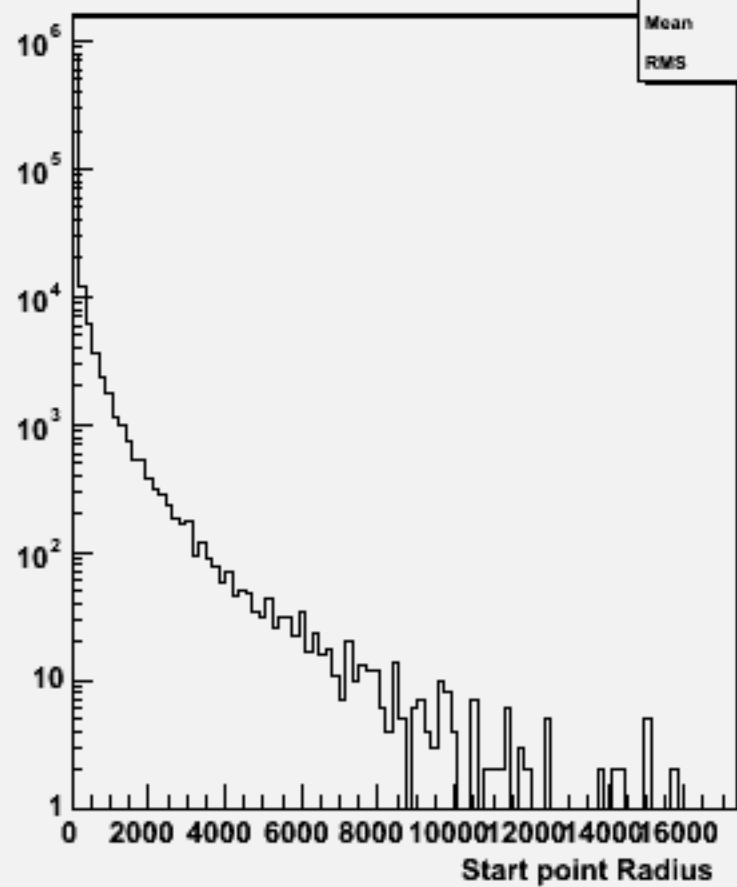
Start point R : w101107 ssn1e1du_o
