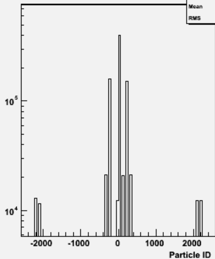
Particle ID : w101107 ssn1e1du_o
