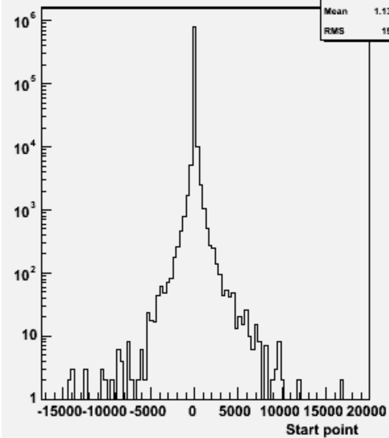
Start point Z : w101107 ssn1e1du_o
