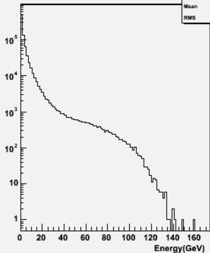
Particle Energy : w101107 ssn1e1du_o
