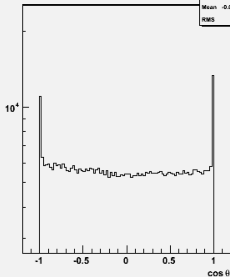
Particle cosθ : w101105 ssn1e1e3n3_o
