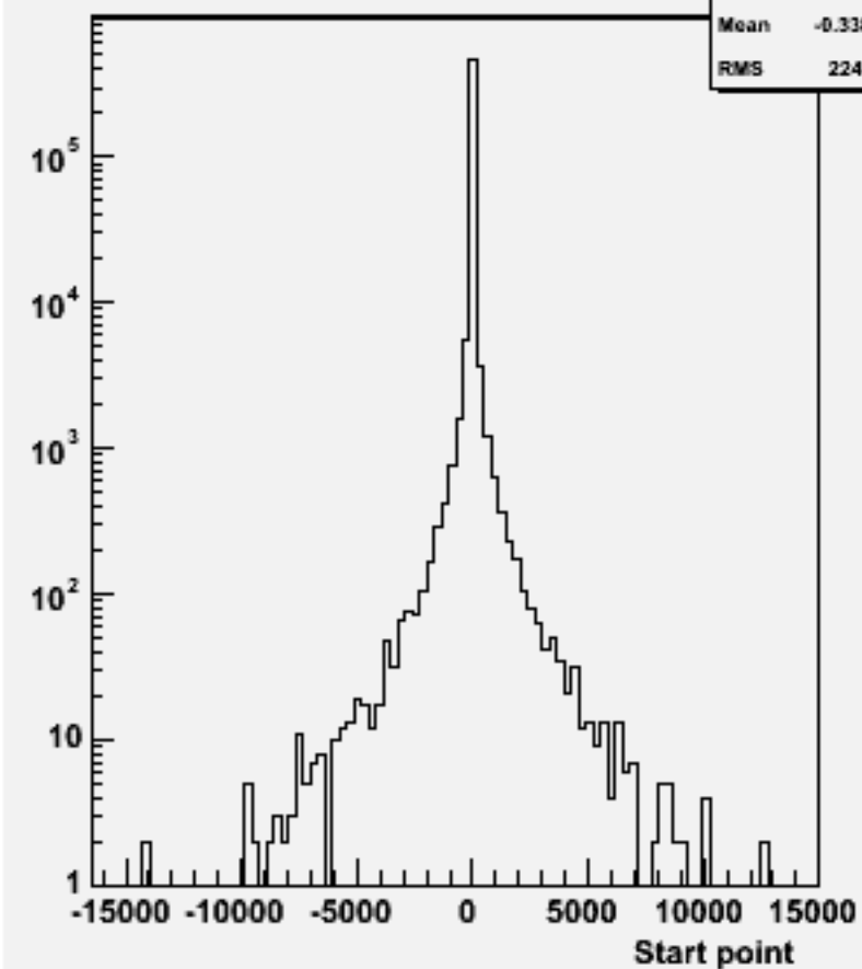
Start point Z : w101105 ssn1e1e3n3_o
