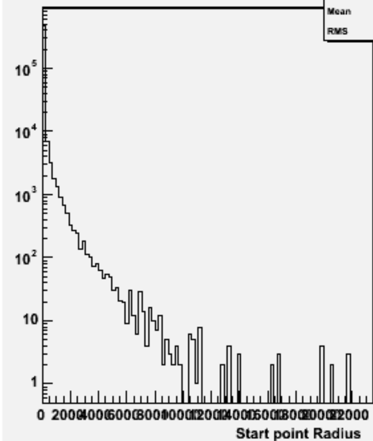
Start point R : w101105 ssn1e1e3n3_o
