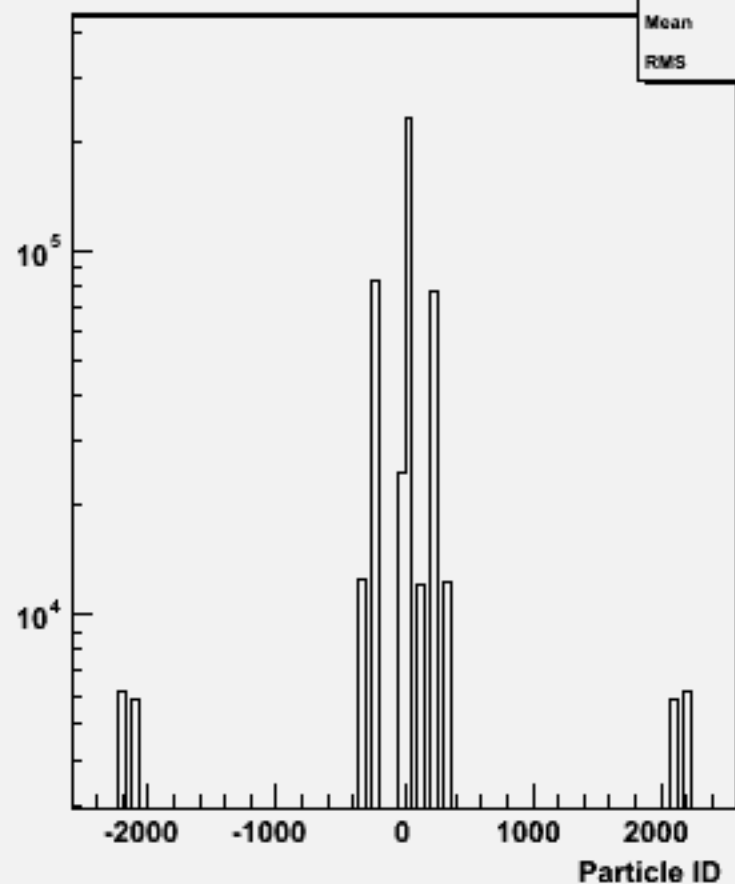
Particle ID : w101105 ssn1e1e3n3_o
