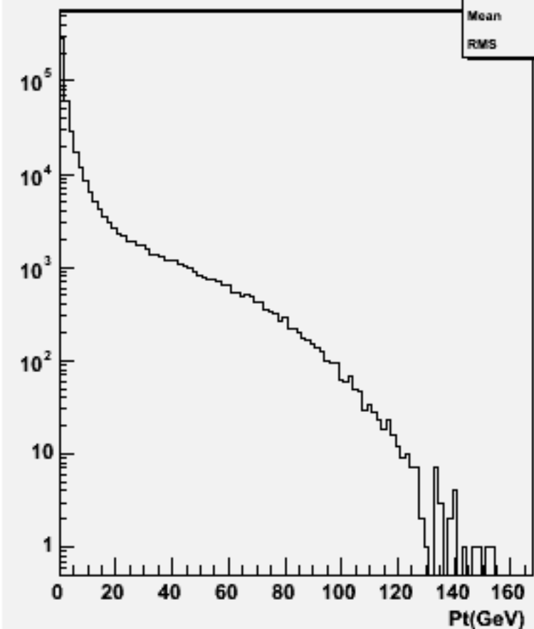
Particle Pt : w101105 ssn1e1e3n3_o
