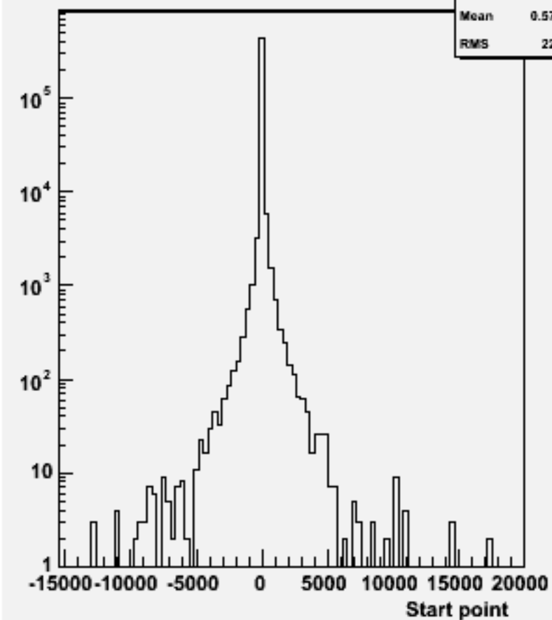
Start point Z : w101101 ssn1e1e2n2_o
