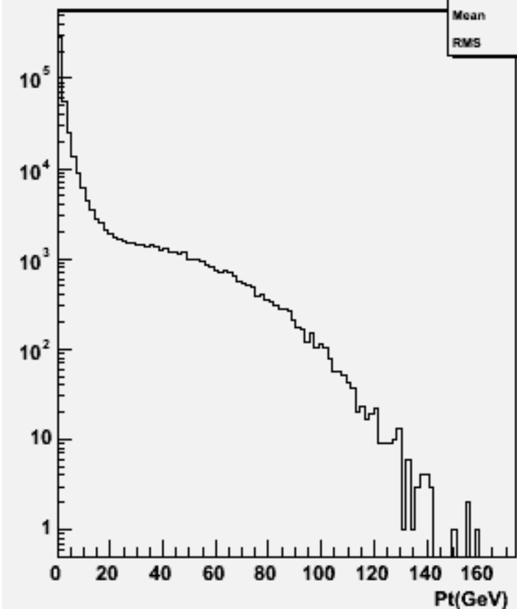
Start point Z : w101101 ssn1e1e2n2_o
