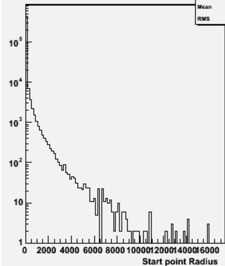
Start point R : w101101 ssn1e1e2n2_o
