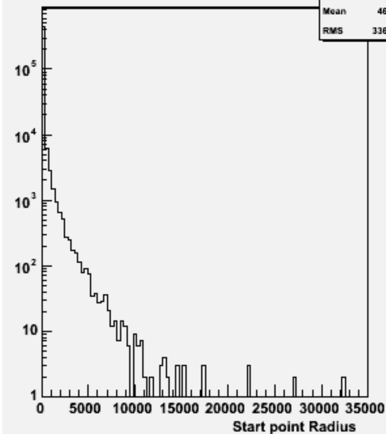
Start point R : w101099 ssn1e1e2n2_o
