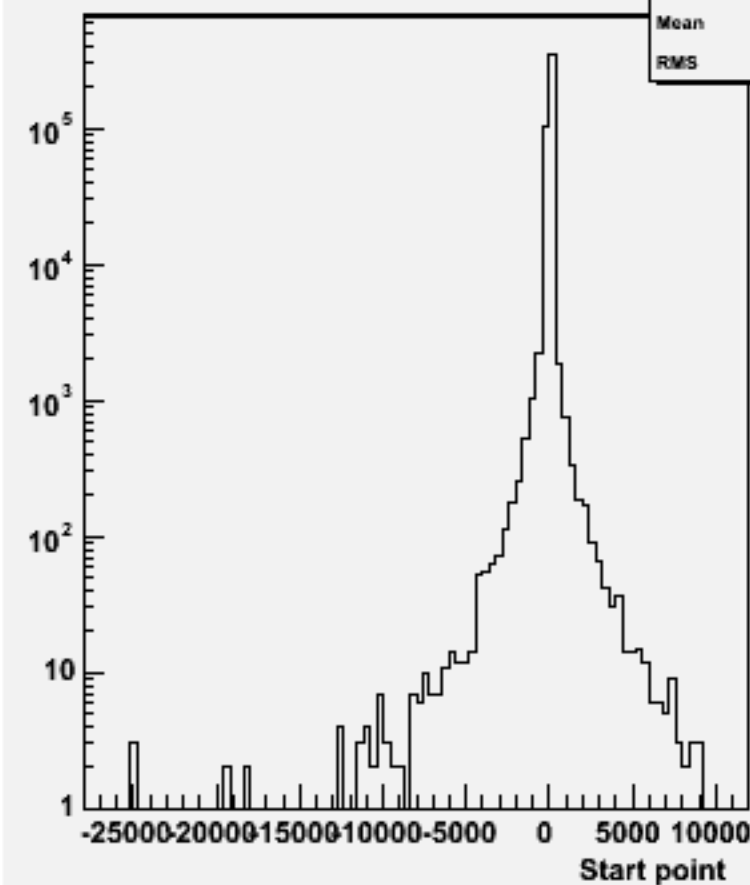
Start point Z : w101099 ssn1e1e2n2_o
