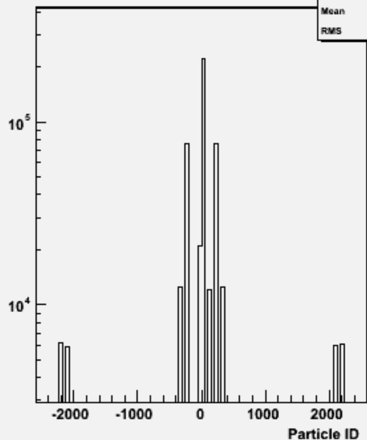
Particle ID : w101099 ssn1e1e2n2_o
