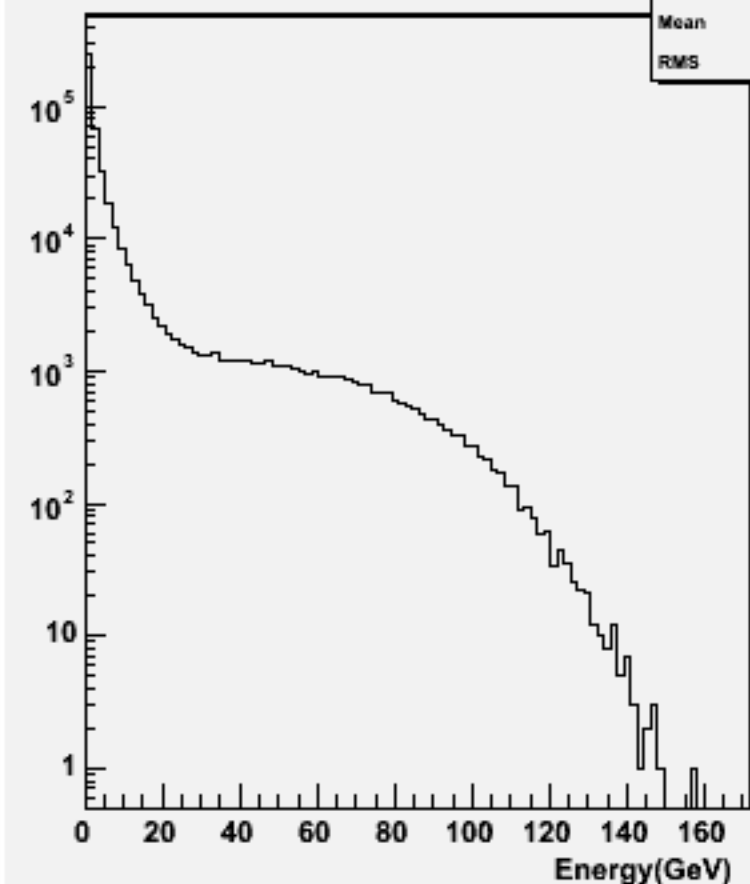
Particle Energy : w101099 ssn1e1e2n2_o
