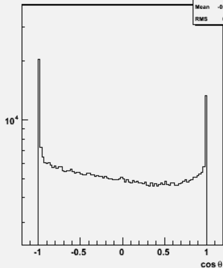
Particle cosθ : w101099 ssn1e1e2n2_o
