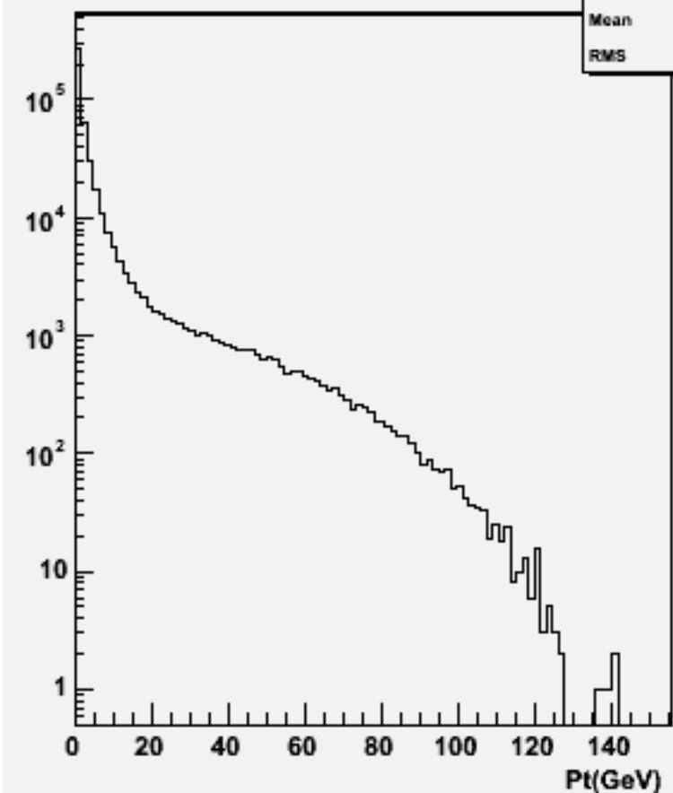
Particle Pt : w101099 ssn1e1e2n2_o
