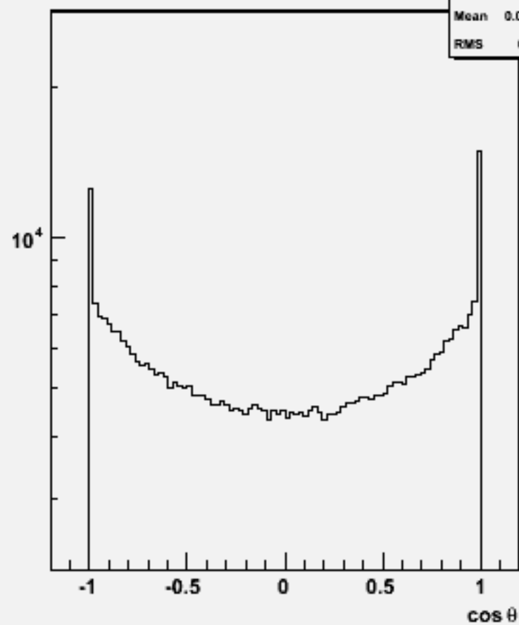
Particle cos \theta : w101097 ssn1e1e1n1_o
