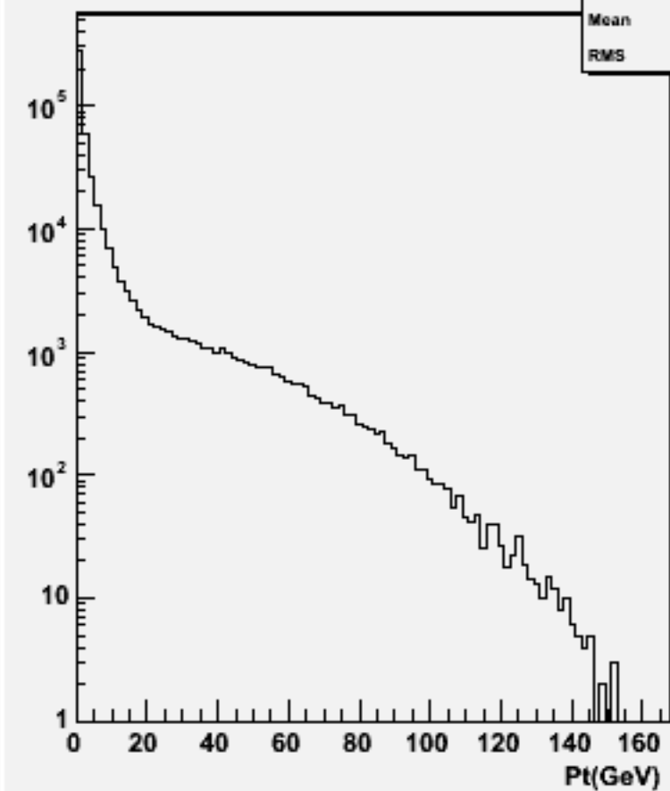
Particle Pt : w101097 ssn1e1e1n1_o
