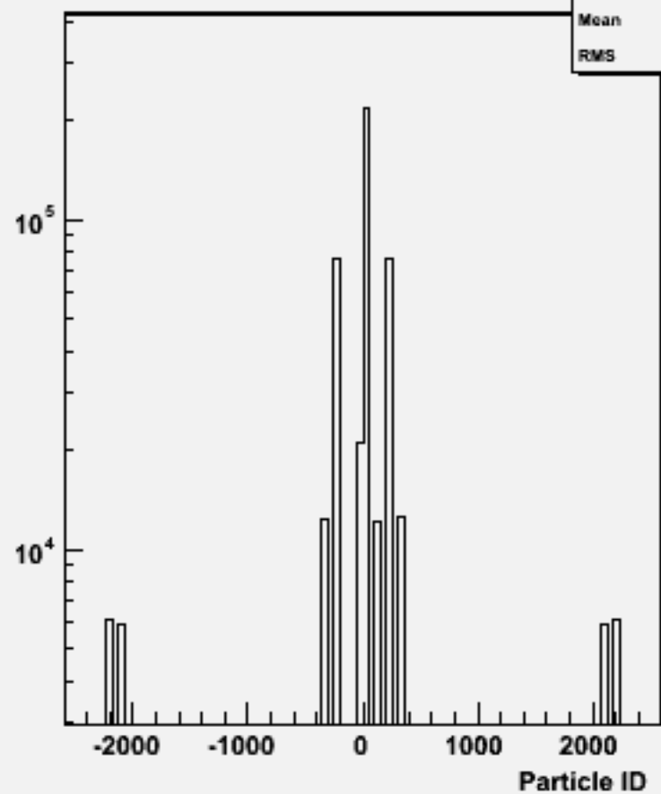
Particle ID : w101097 ssn1e1e1n1_o
