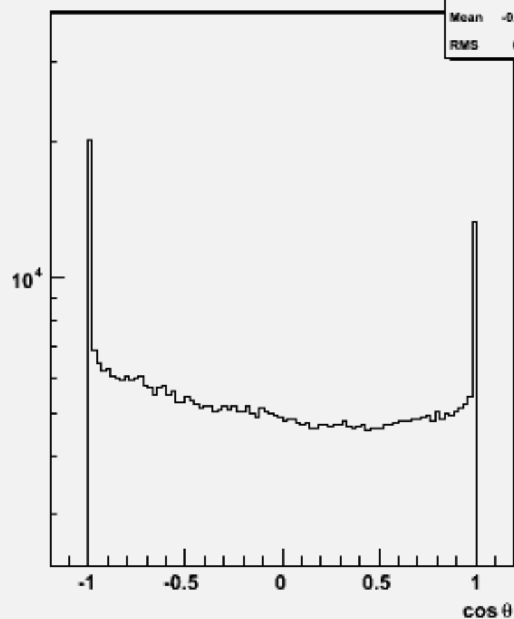
Particle cosθ : w101095 ssn1e1e1n1_o
