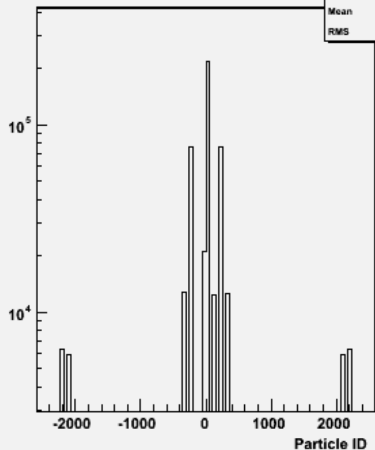
Particle ID : w101095 ssn1e1e1n1_o
