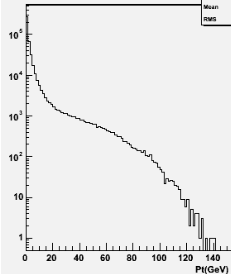
Particle Pt : w101095 ssn1e1e1n1_o
