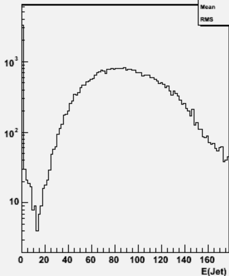
Jet energies(All jets)w101092 ddcssc_o
