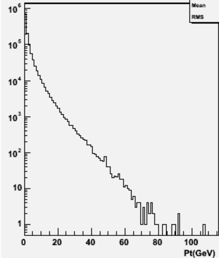
Start point Z : w101089 ddcsdu_o
