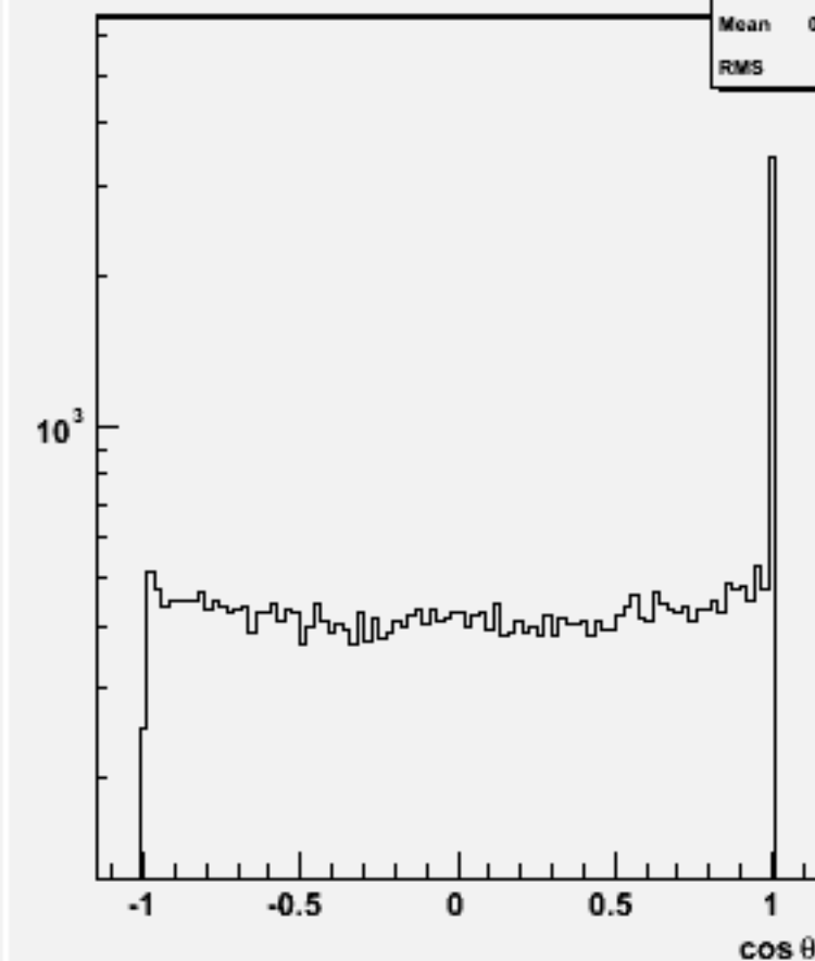
Jet cos \theta (All jets)w101089 ddcdu_o
