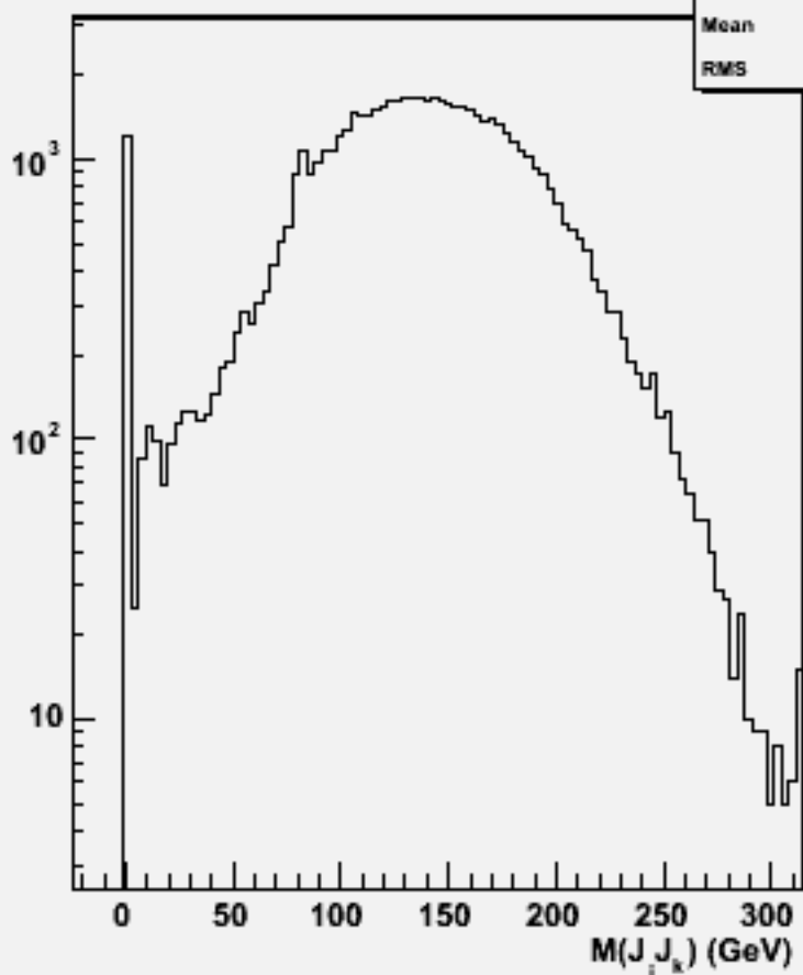
2jets mass(All comb)w101089 ddcdu_o
