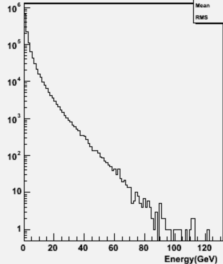
Start point R : w101089 ddcsdu_o
