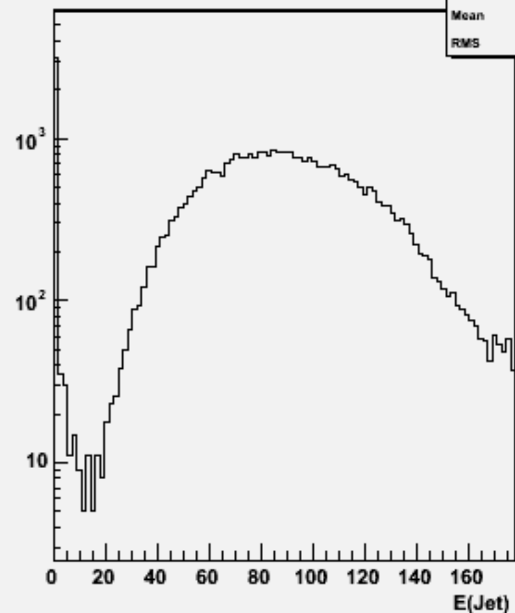
Jet energies(All jets)w101089 ddcdu_o
