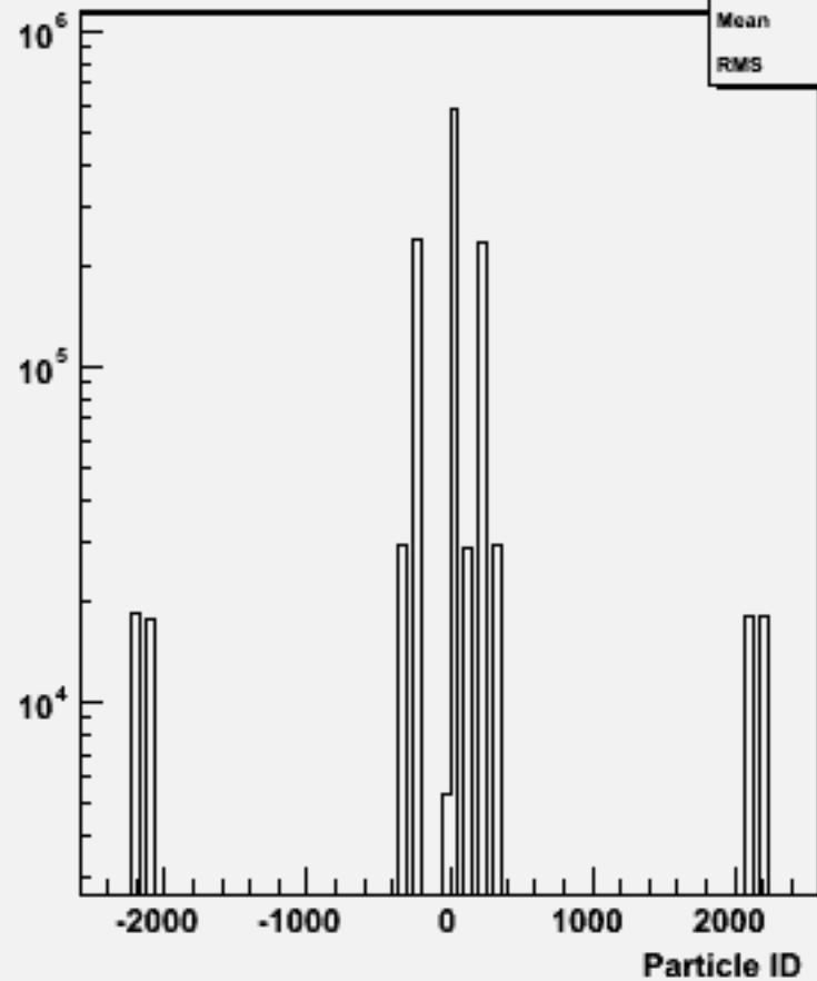
Particle cosθ : w101089 ddcsdu_o
