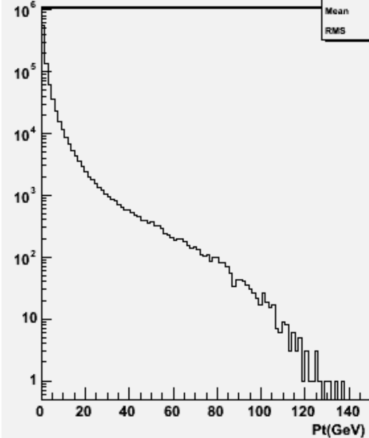
Particle Pt : w101085 ddcse3n3_o
