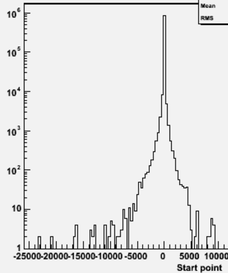
Start point Z : w101084 ddcse3n3_o
