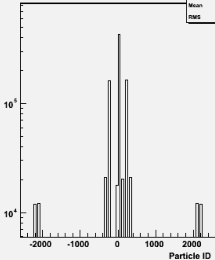
Particle ID : w101084 ddcse3n3_o
