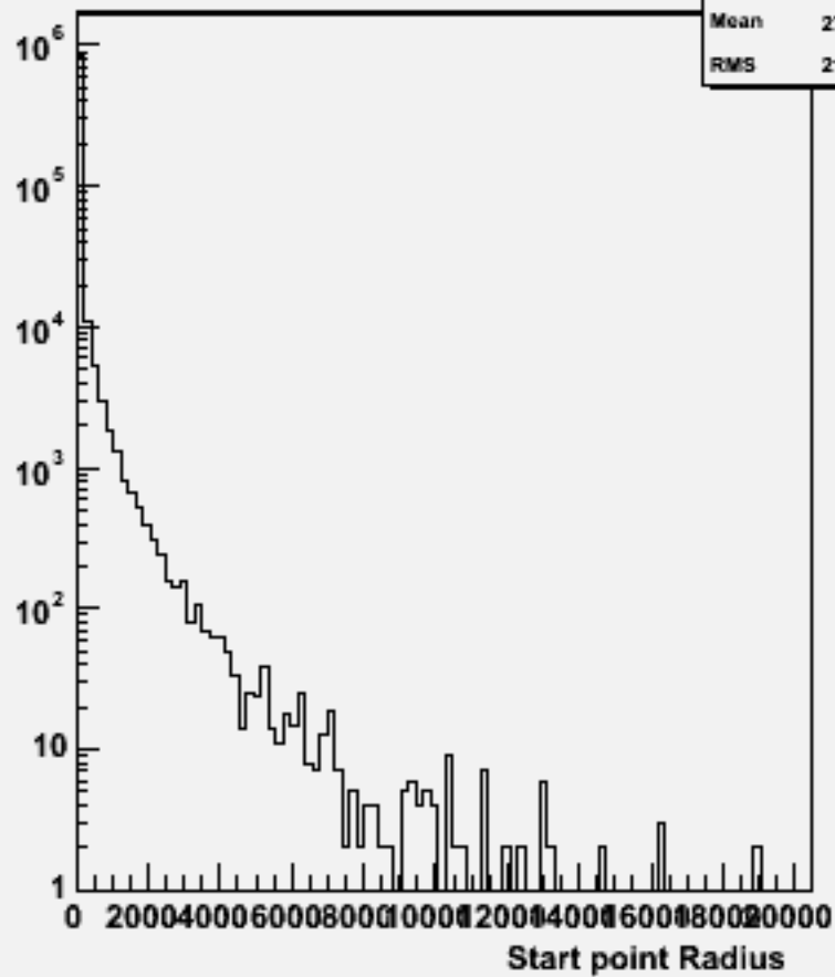
Start point R : w101084 ddcse3n3_o
