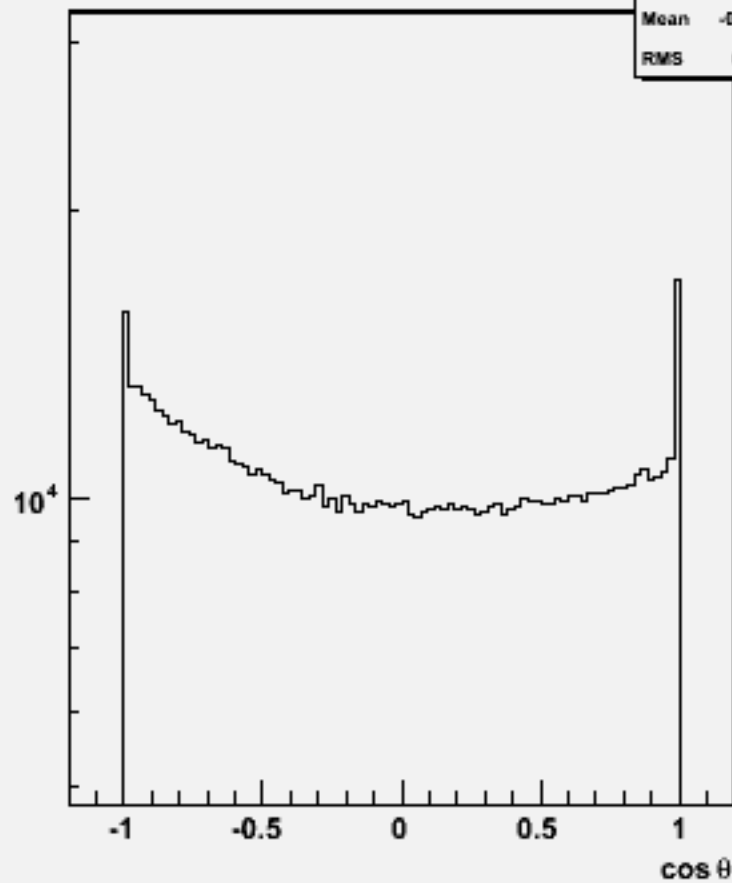
Particle cos \theta : w101084 ddcse3n3_o
