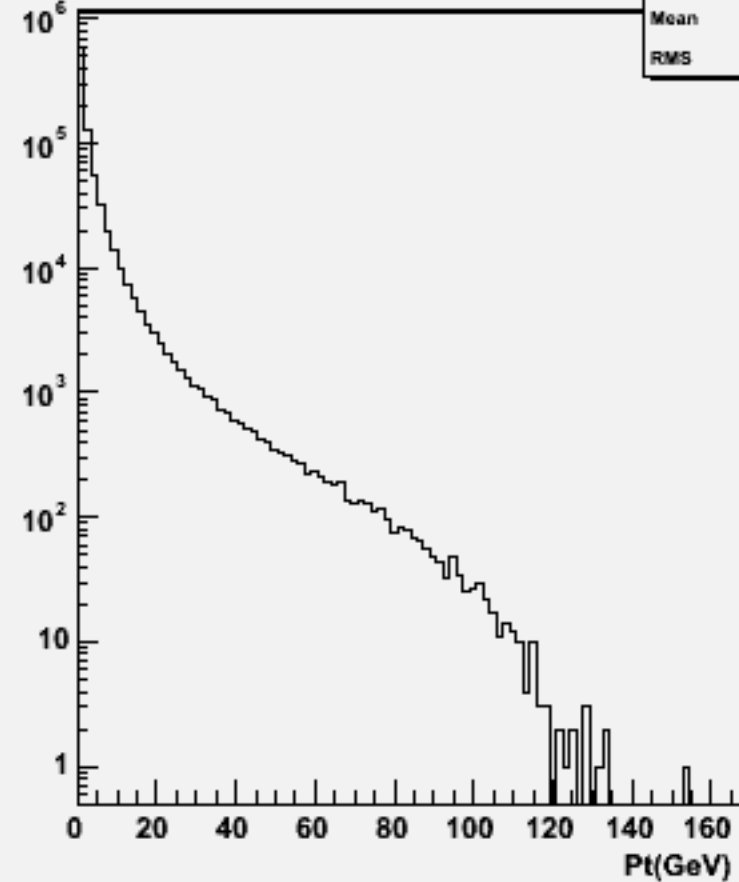
Particle Pt : w101084 ddcse3n3_o
