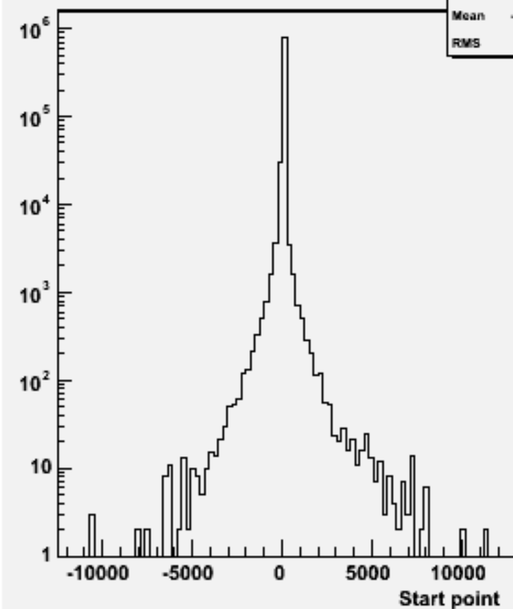
Start point Z : w101081 ddcse2n2_o
