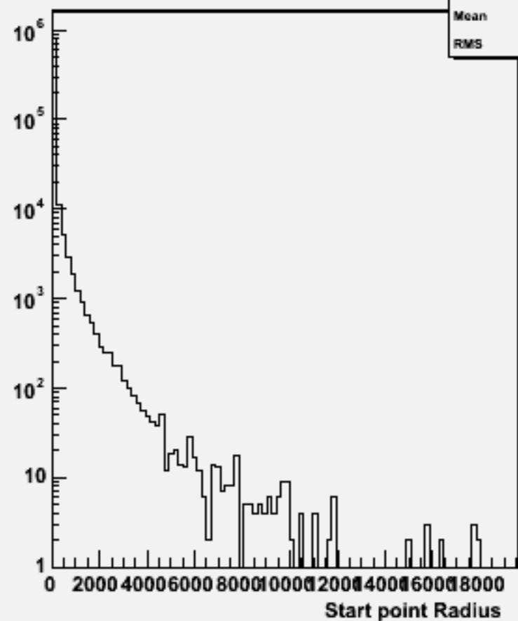
Start point R : w101081 ddcse2n2_o
