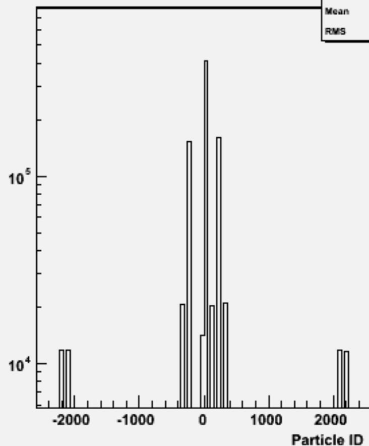
Particle ID : w101081 ddcse2n2_o
