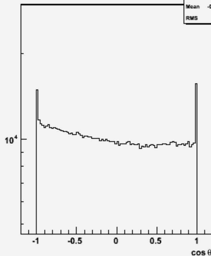
Particle cos \theta : w101081 ddcse2n2_o
