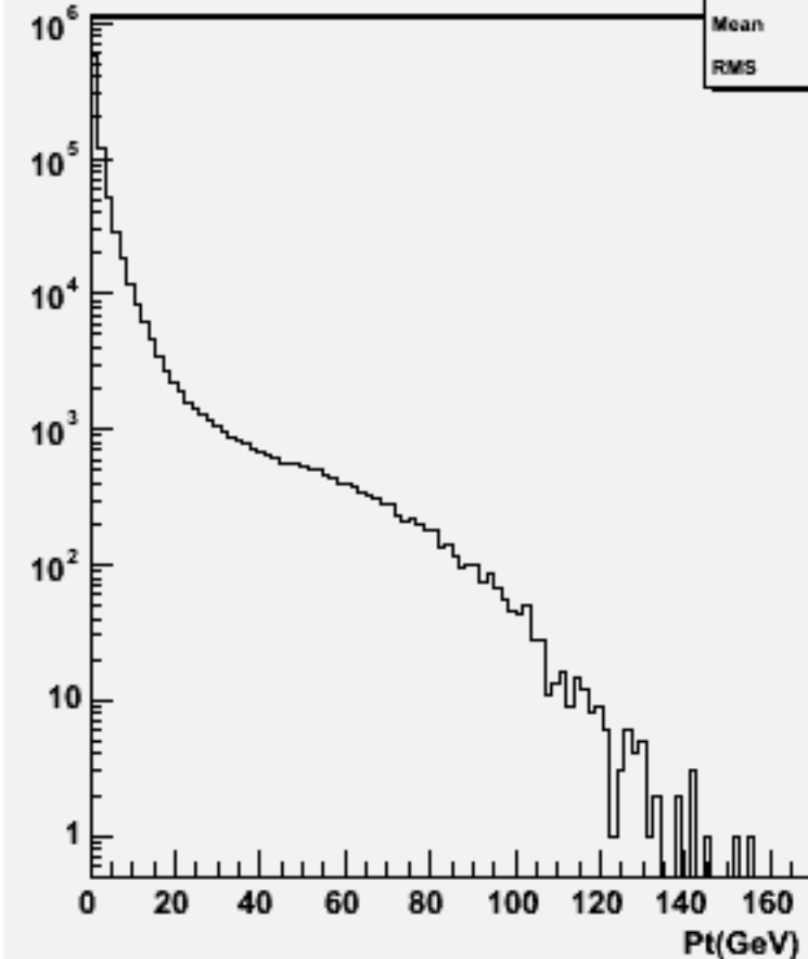
Particle Pt : w101081 ddcse2n2_o
