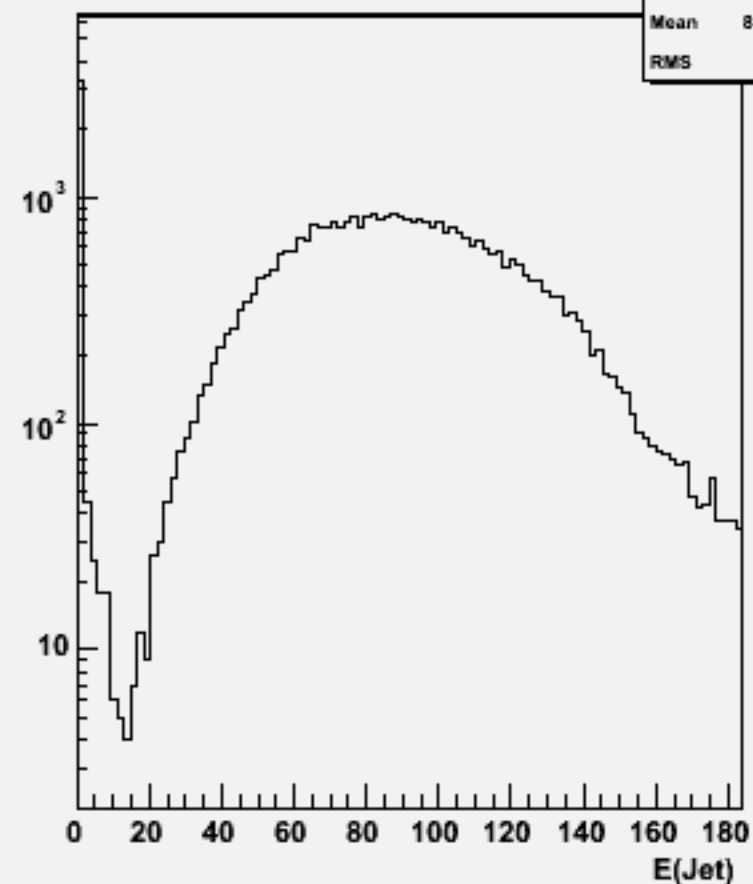
Jet energies(All jets)w101072 ddudsc_o
