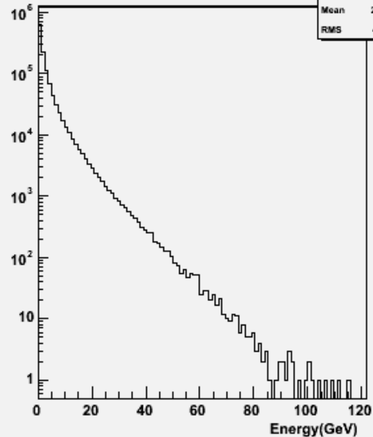
Start point R : w101072 ddudsc_o
