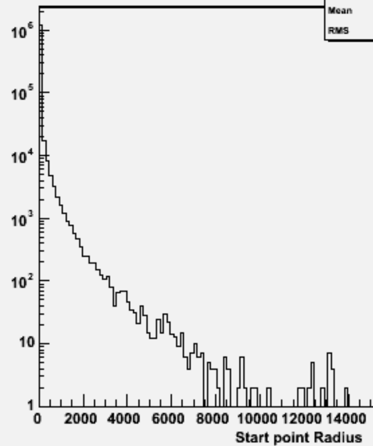
Start point R : w101072 ddudsc_o
