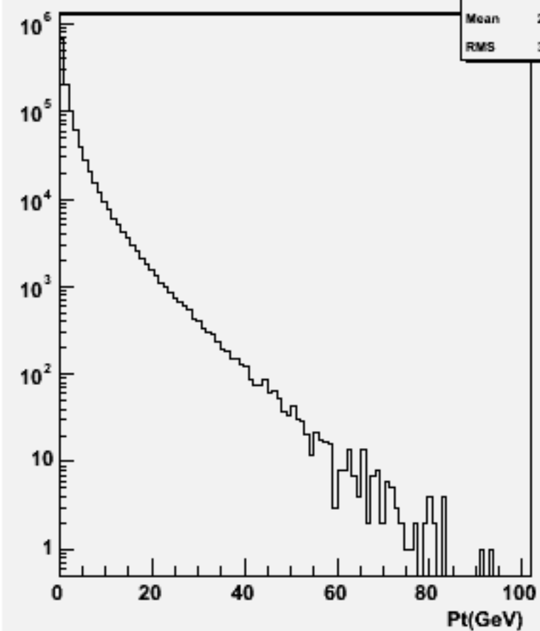
Particle Pt : w101069 dduddu_o
