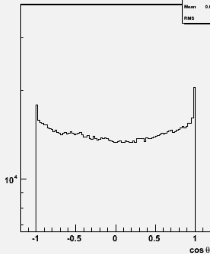
Particle cos \theta : w101069 dduddu_o
