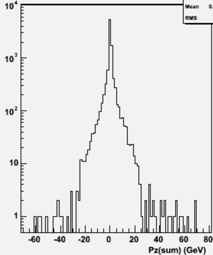
Pz Sum: w101069 dduddu_o
