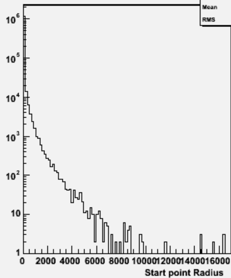
Start point R : w101069 dduddu_o
