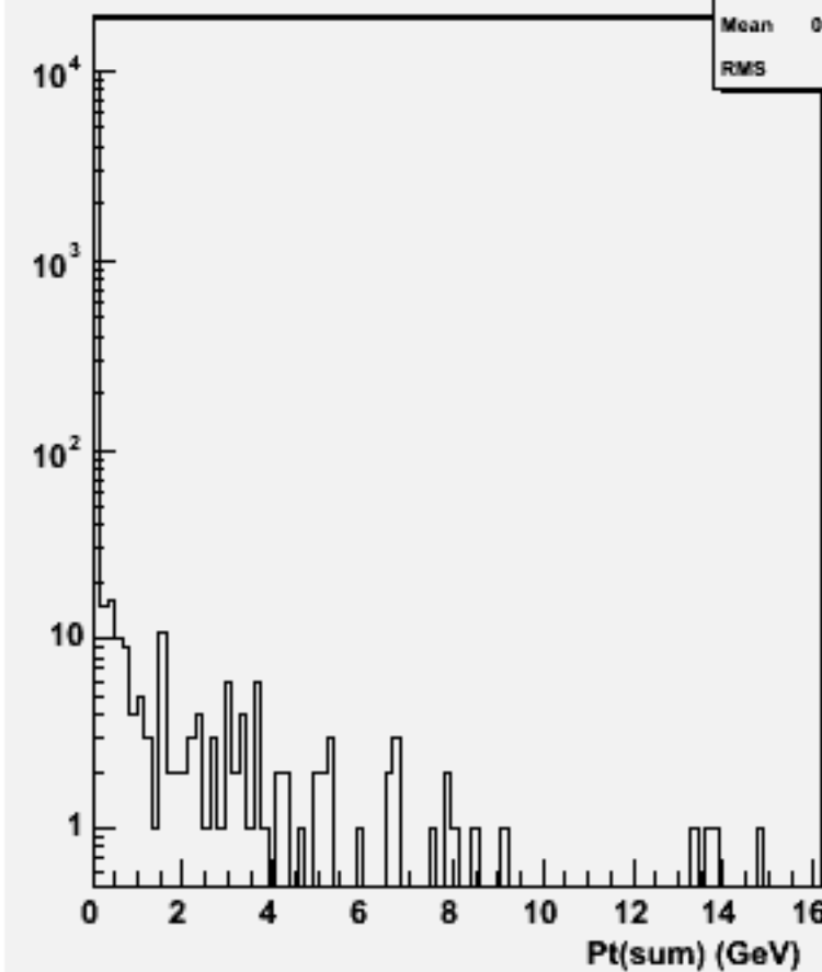
Pt Sum: w101069 dduddu_o
