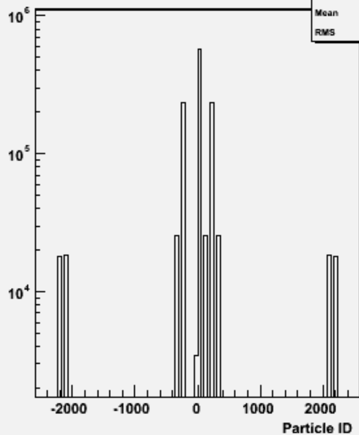
Particle ID : w101069 dduddu_o
