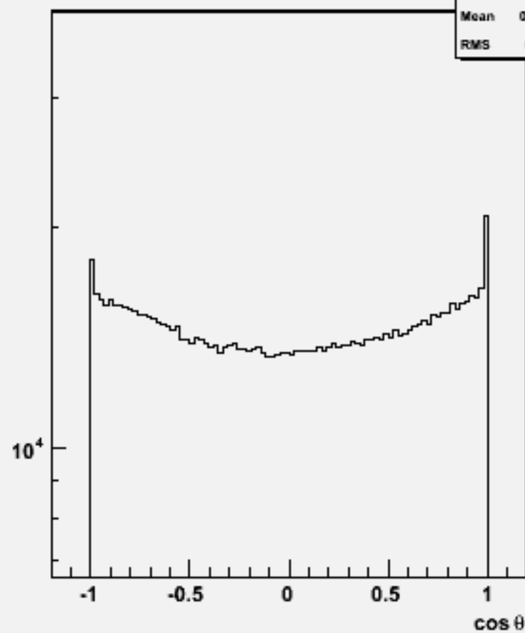
Particle cosθ : w101068 dduddu_o
