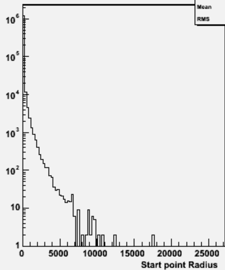
Start point R : w101068 dduddu_o
