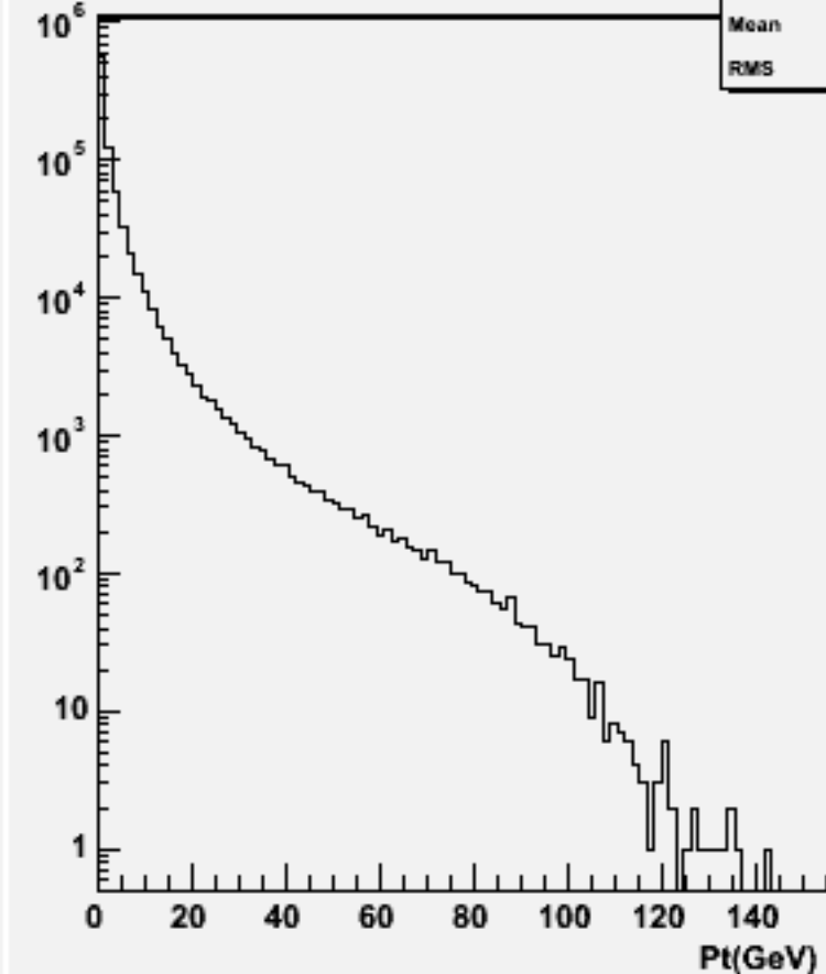
Particle Pt : w101064 ddude3n3_o
