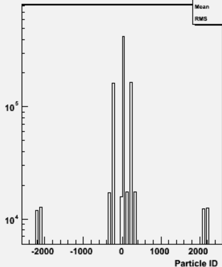
Particle ID : w101064 ddude3n3_o
