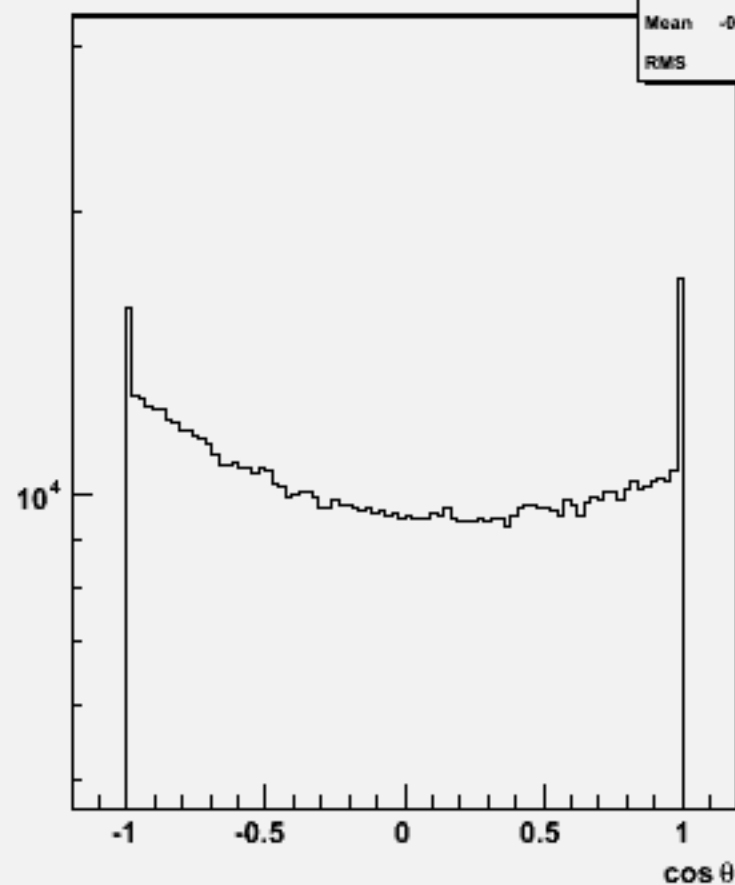
Particle cos \theta : w101064 ddude3n3_o
