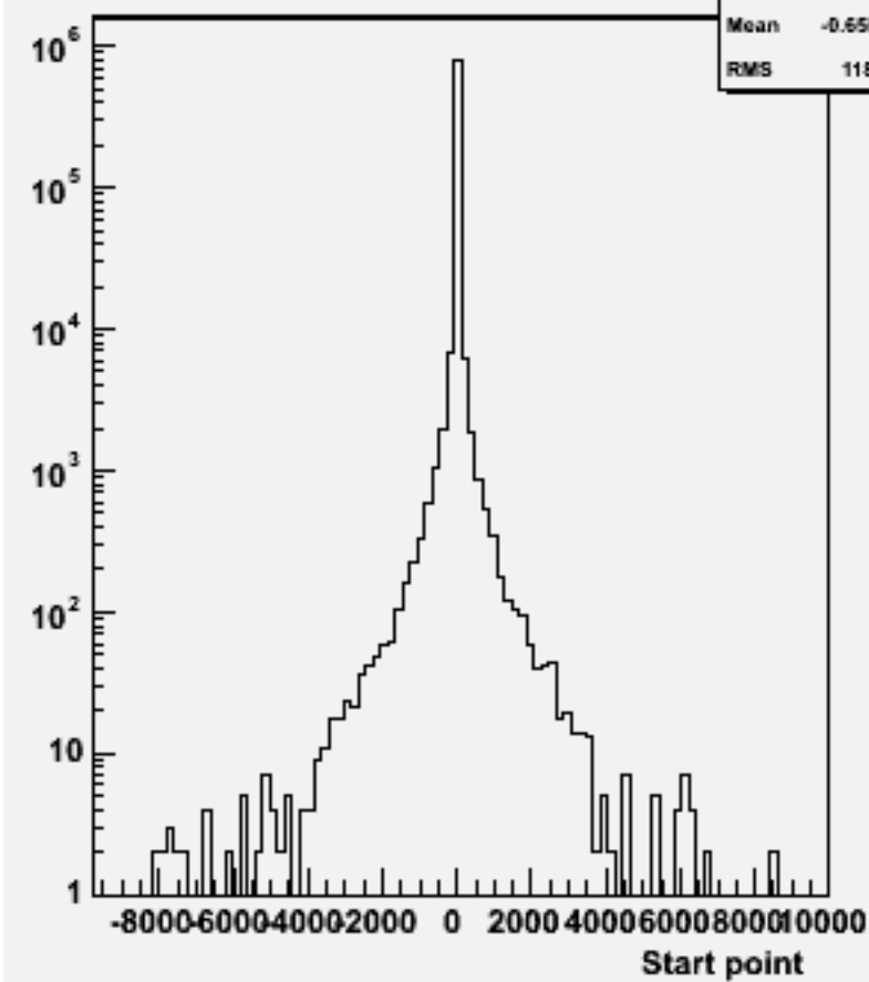
Start point Z : w101061 ddude2n2_o
