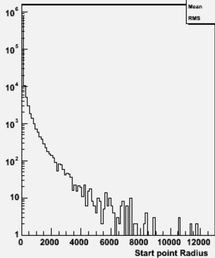
Start point R : w101061 ddude2n2_o
