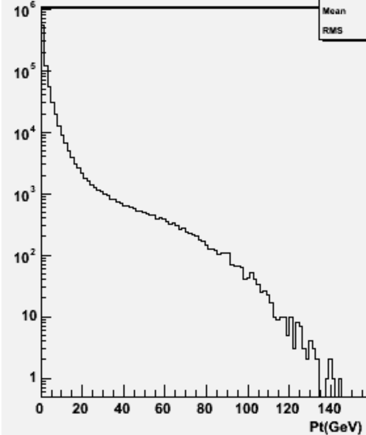
Particle Pt : w101061 ddude2n2_o
