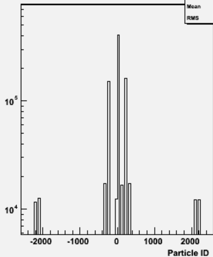
Particle ID : w101061 ddude2n2_o
