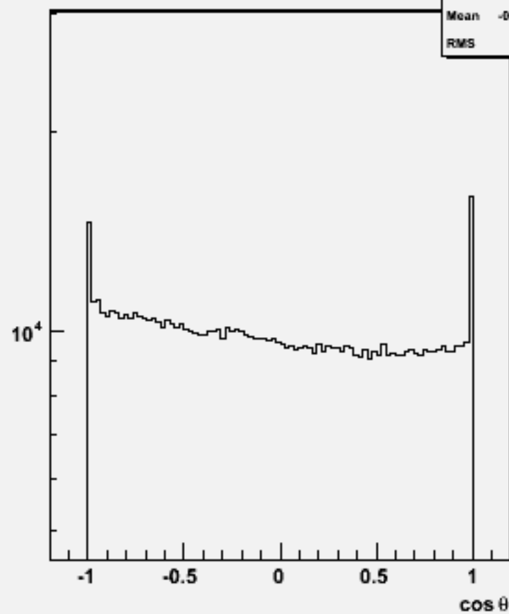
Particle cos \theta : w101061 ddude2n2_o
