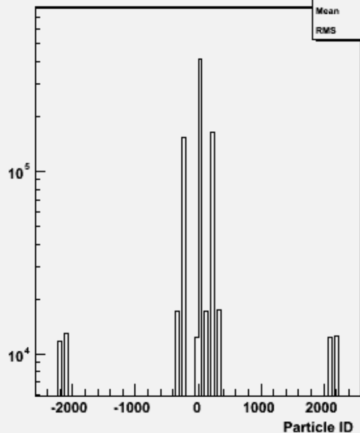
Particle ID : w101060 ddude2n2_o
