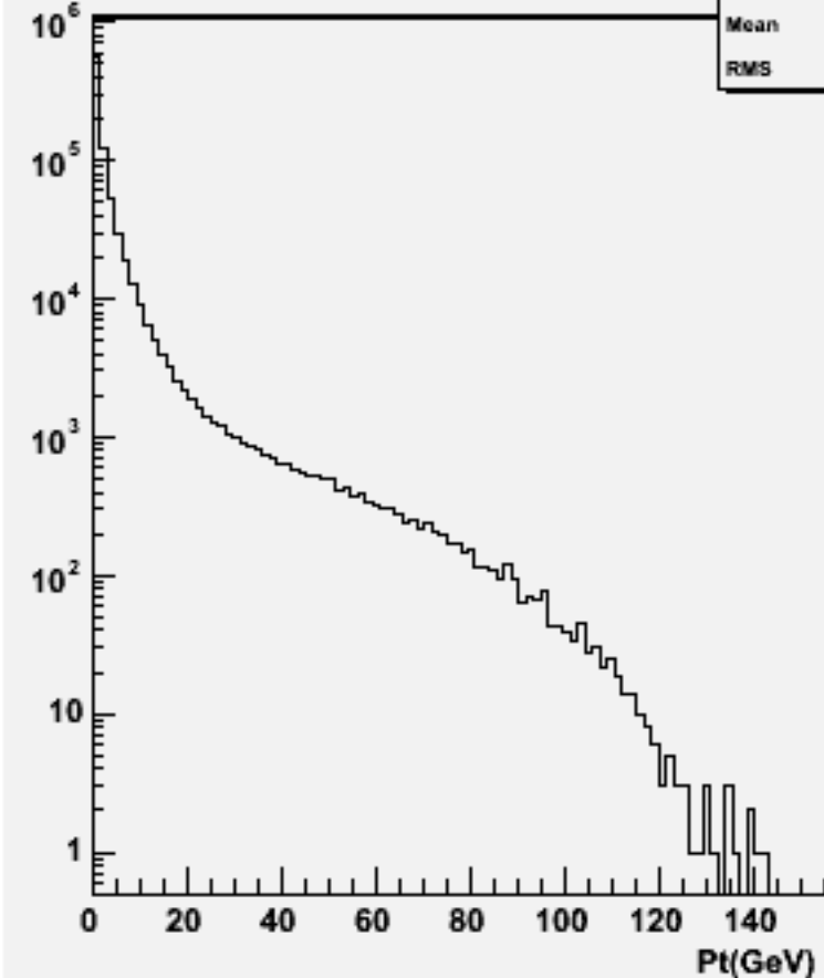
Particle Pt : w101060 ddude2n2_o
