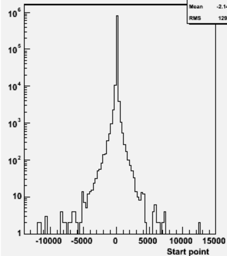
Start point Z : w101060 ddude2n2_o
