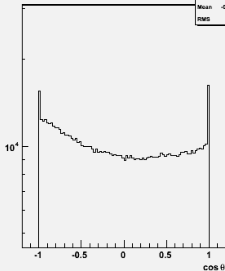
Particle cos \theta : w101060 ddude2n2_o
