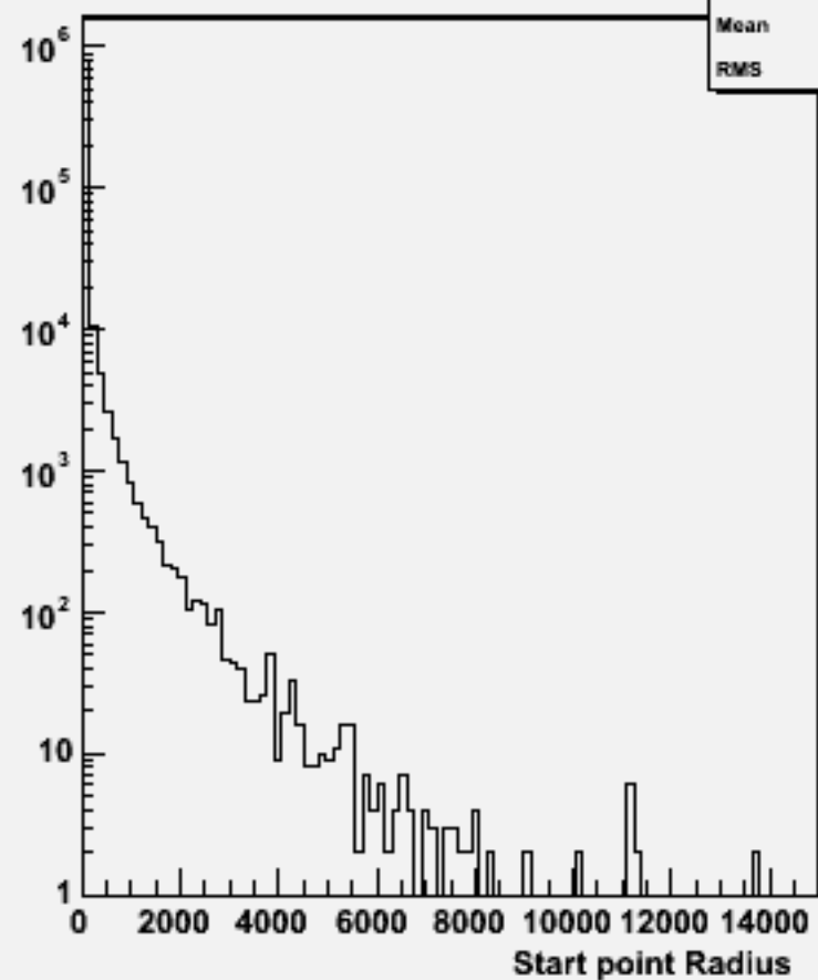
Start point R : w101060 ddude2n2_o
