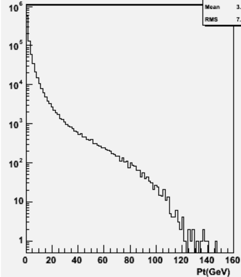
Particle Pt : w101053 ddn3e3sc_o
