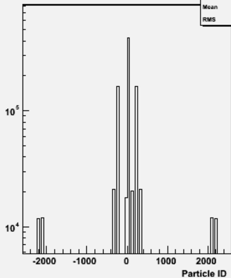
Particle ID : w101053 ddn3e3sc_o
