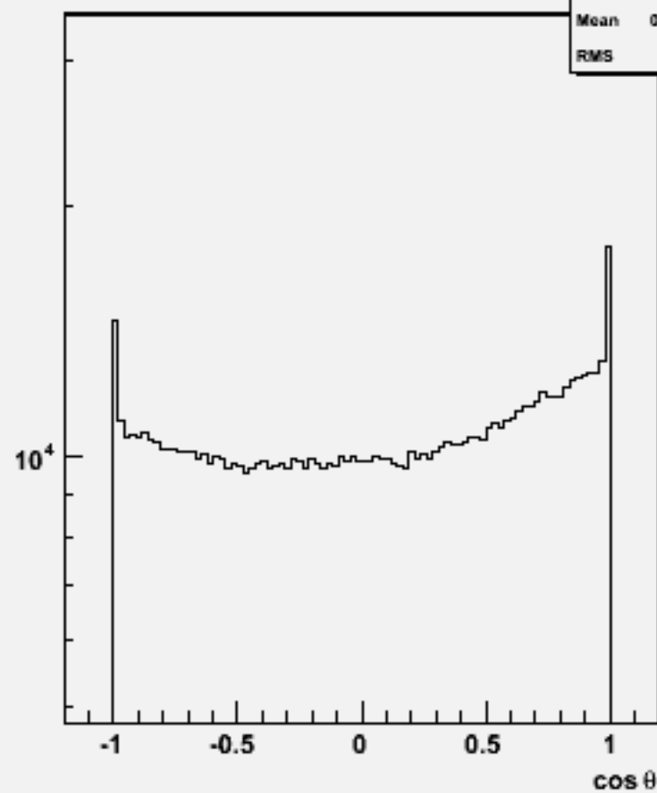
Particle cos \theta : w101052 ddn3e3sc_o
