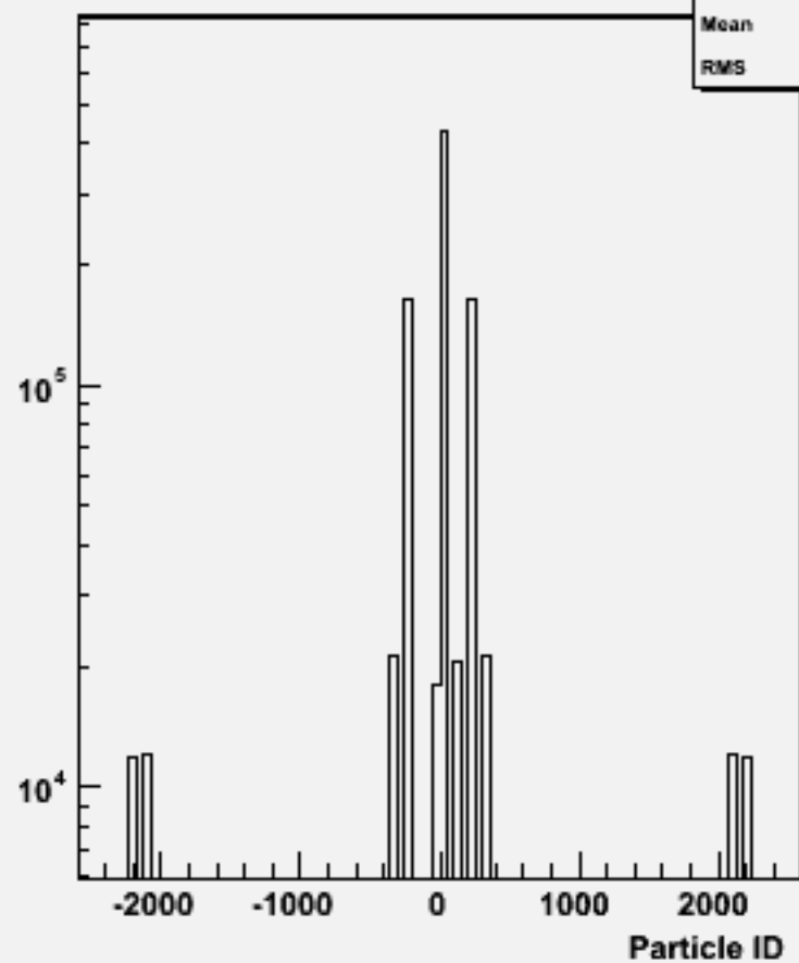
Particle ID : w101052 ddn3e3sc_o
