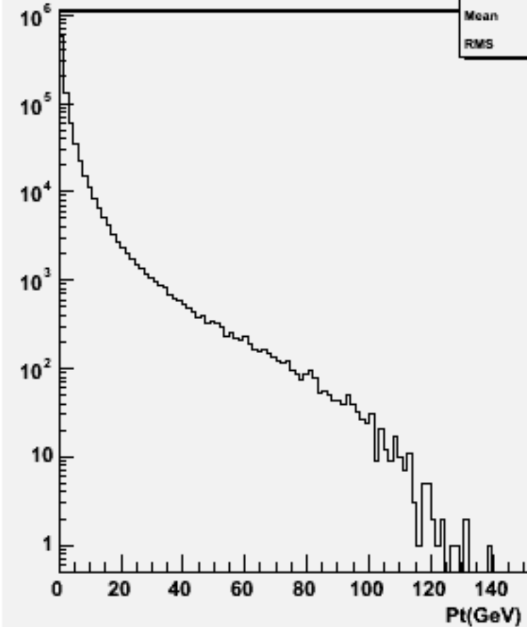
Particle Pt : w101052 ddn3e3sc_o
