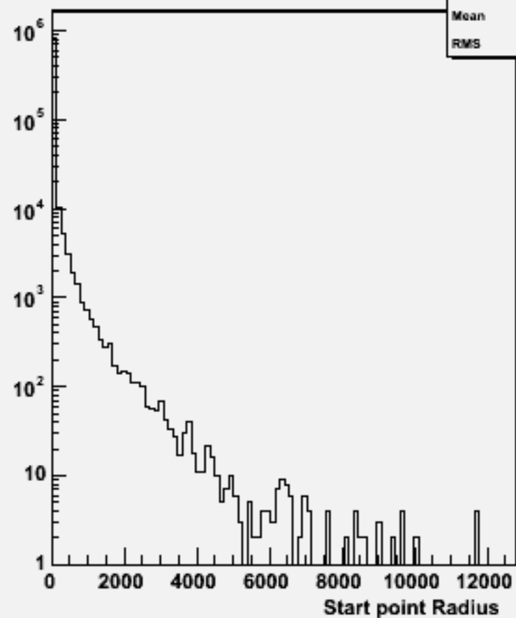
Start point R : w101048 ddn3e3du_o
