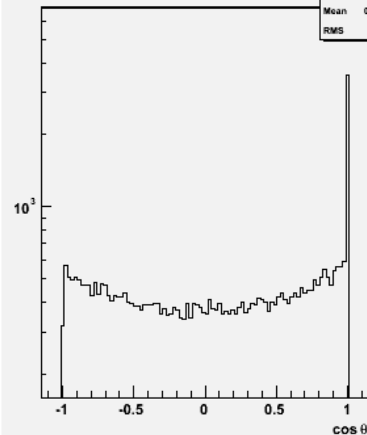
Jet cos \theta (All jets)w101048 ddn3e3du_o
