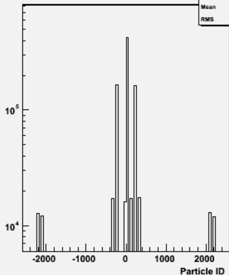
Particle ID : w101048 ddn3e3du_o
