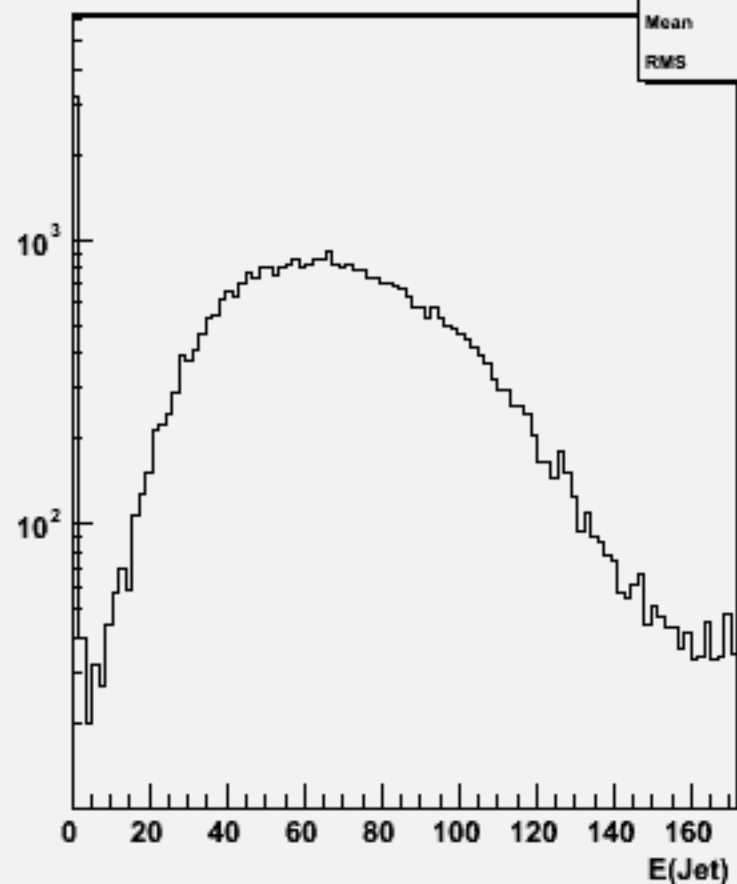
Jet energies(All jets)w101048 ddn3e3du_o
