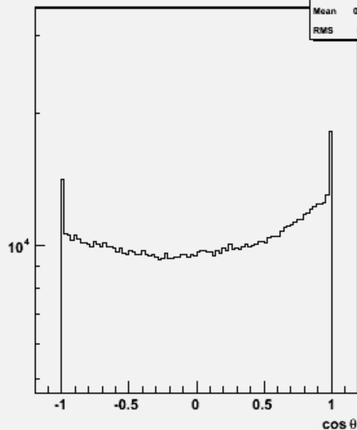
Particle cos \theta : w101048 ddn3e3du_o
