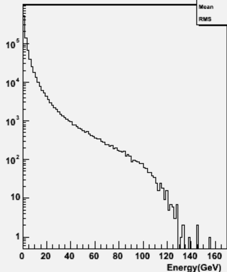
Particle Energy : w101048 ddn3e3du_o
