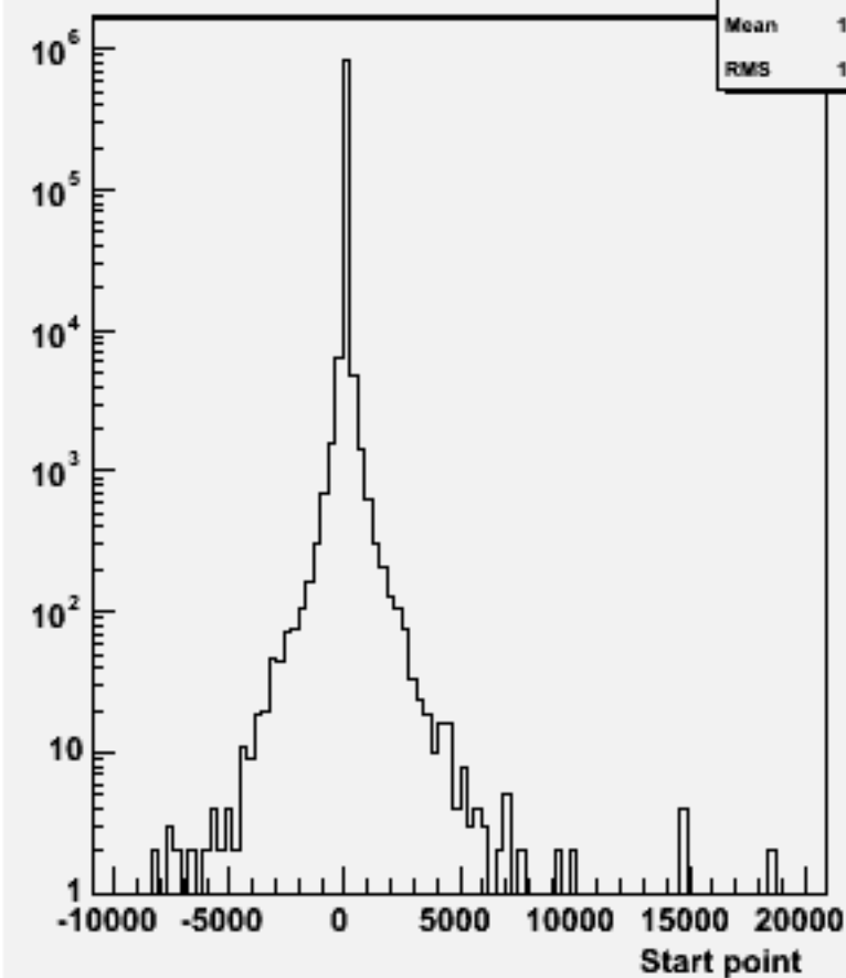
Start point Z : w101048 ddn3e3du_o
