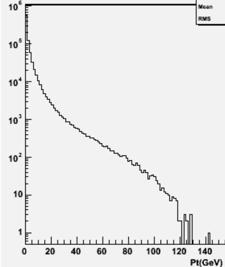
Particle Pt : w101048 ddn3e3du_o
