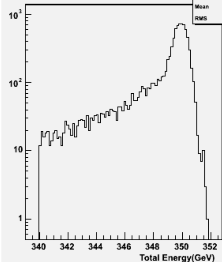
Pz Sum: w101041 ddn3e3e2n2_o
