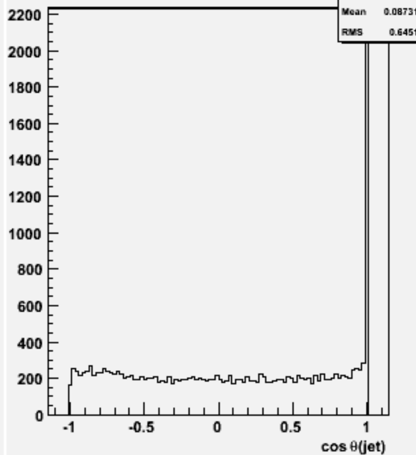
cos \theta for 2-jets :w101041 ddn3e3e2n2_o
