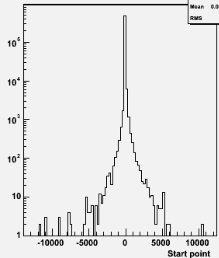
Start point Z : w101041 ddn3e3e2n2_o
