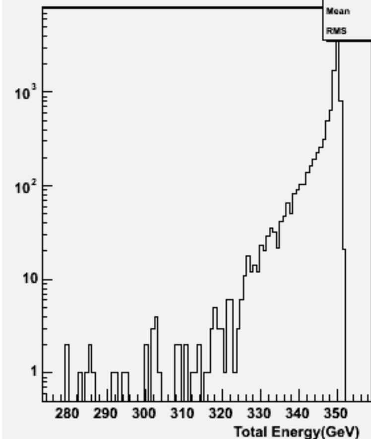
Pt Sum: w101041 ddn3e3e2n2_o
