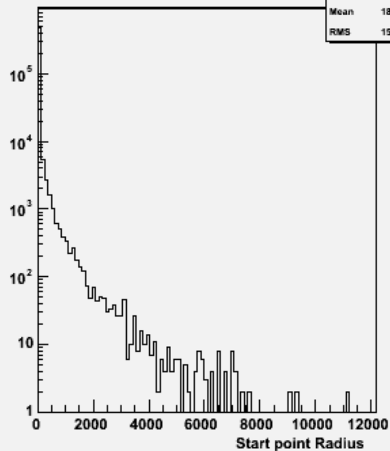
Start point R : w101041 ddn3e3e2n2_o
