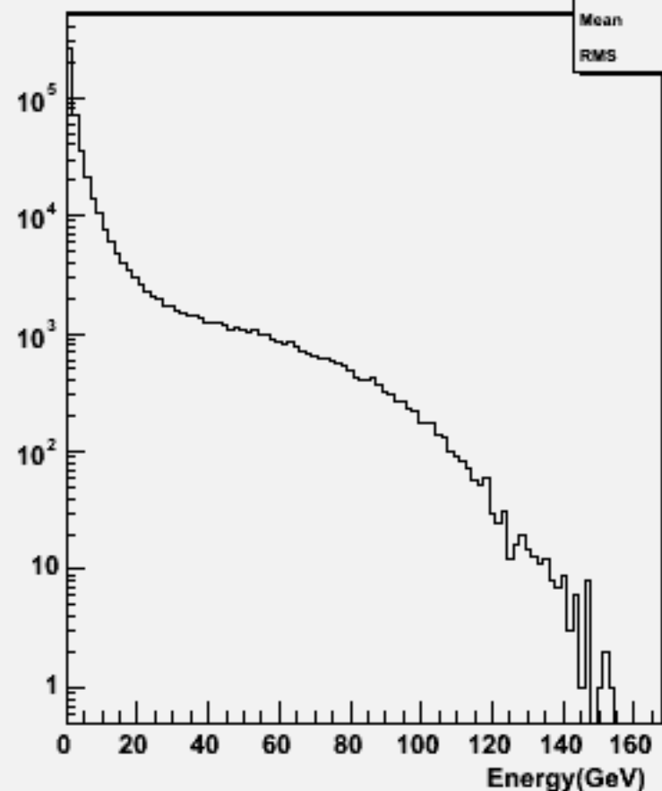
Particle Energy : w101041 ddn3e3e2n2_o
