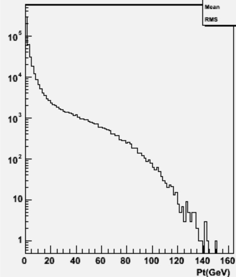
Particle Pt : w101041 ddn3e3e2n2_o
