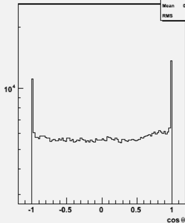
Particle cos \theta : w101041 ddn3e3e2n2_o
