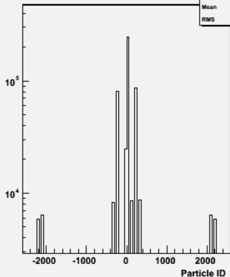
Particle ID : w101041 ddn3e3e2n2_o
