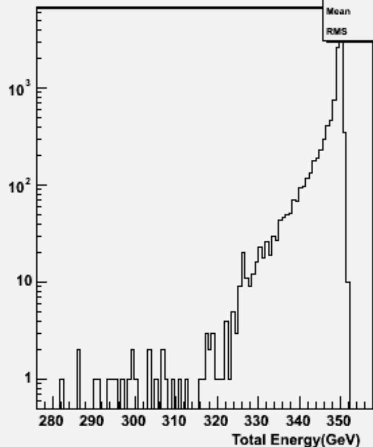
Pt Sum: w101040 ddn3e3e2n2_o
