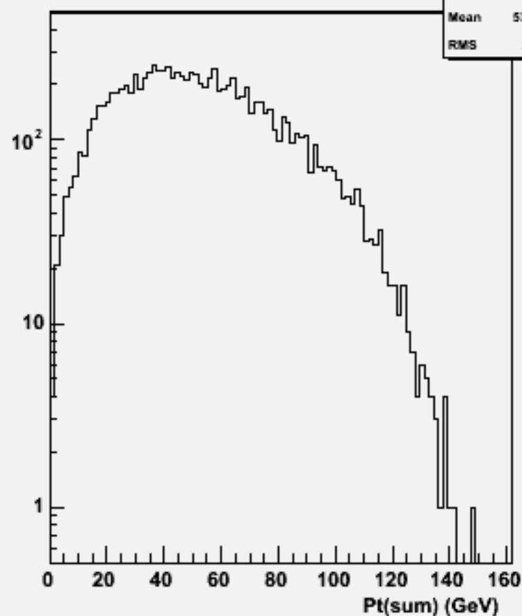
Pt Sum: w101040 ddn3e3e2n2_o
