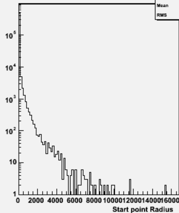
Start point R : w101040 ddn3e3e2n2_o
