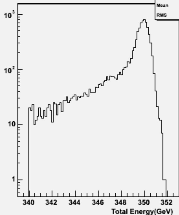
Pz Sum: w101040 ddn3e3e2n2_o
