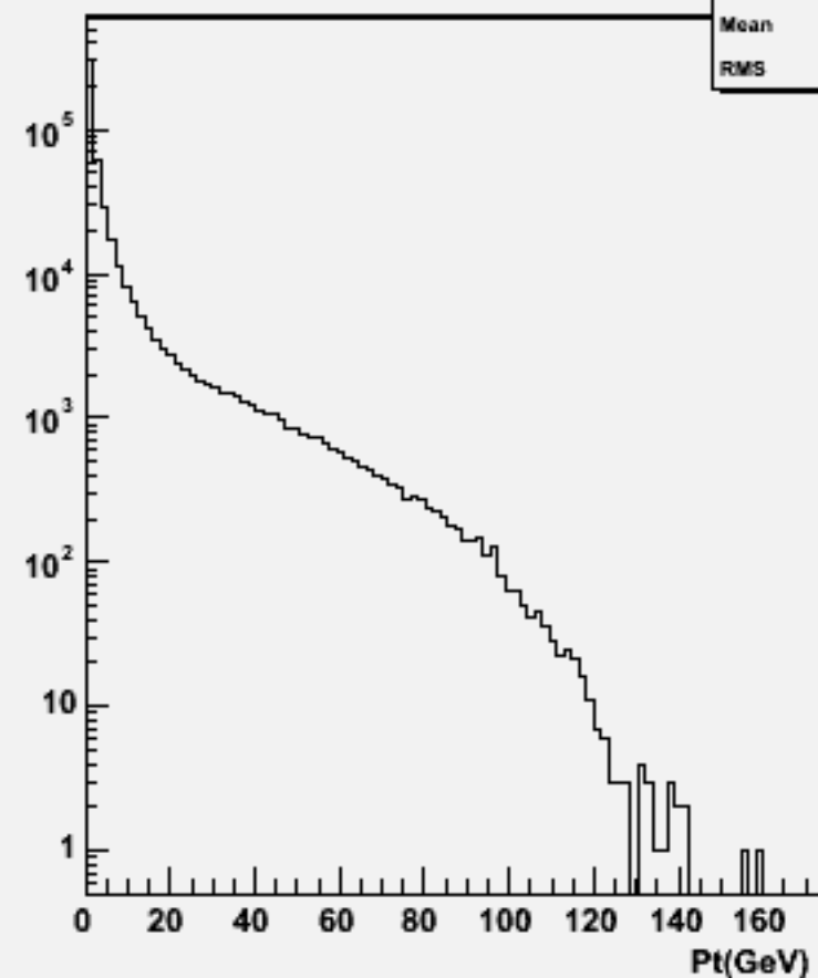
Start point Z : w101040 ddn3e3e2n2_o
