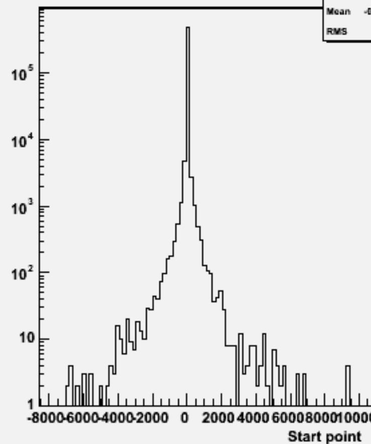
Start point Z : w101040 ddn3e3e2n2_o
