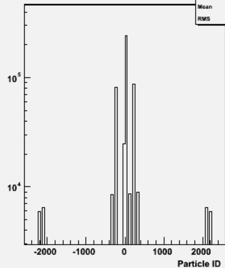
Particle ID : w101037 ddn3e3e1n1_o
