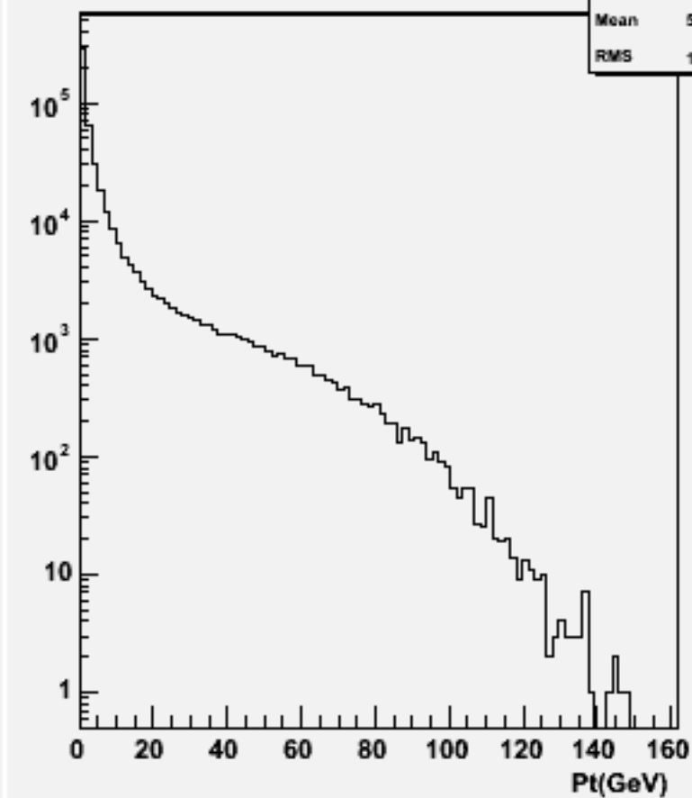
Particle Pt : w101037 ddn3e3e1n1_o
