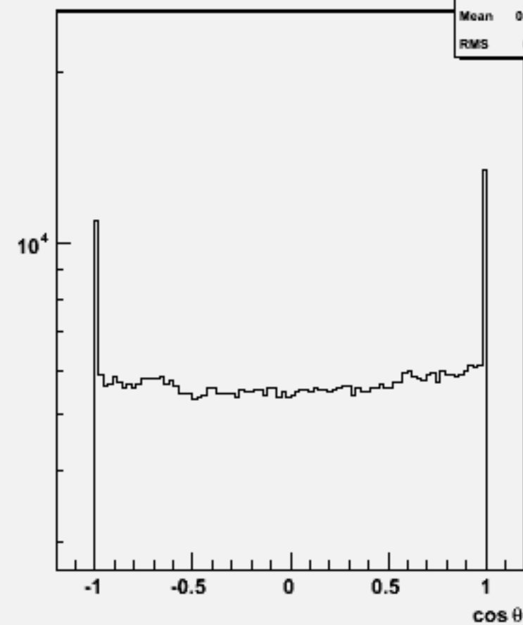
Particle cos \theta : w101037 ddn3e3e1n1_o
