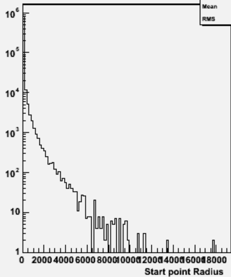
Start point R : w101033 ddn2e2sc_o
