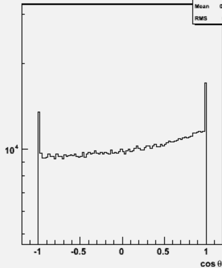
Particle cos \theta : w101033 ddn2e2sc_o
