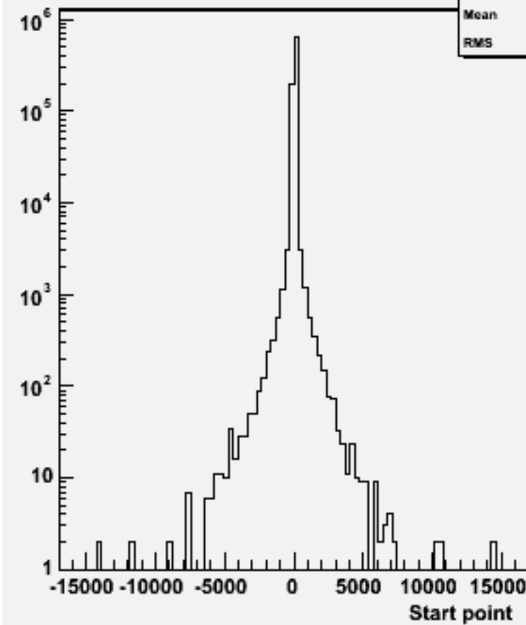
Start point Z : w101033 ddn2e2sc_o
