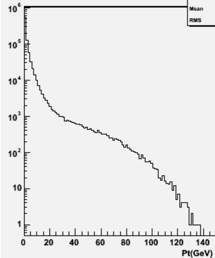
Particle Pt : w101033 ddn2e2sc_o
