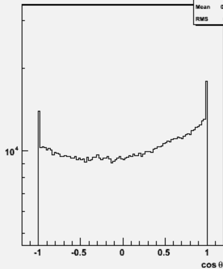
Particle cos \theta : w101032 ddn2e2sc_o
