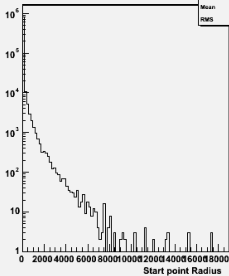
Start point R : w101032 ddn2e2sc_o
