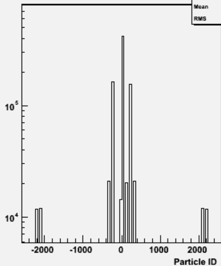
Particle ID : w101032 ddn2e2sc_o
