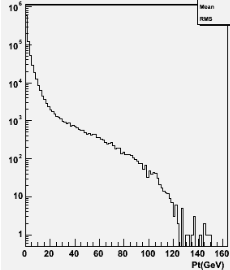
Particle Pt : w101032 ddn2e2sc_o
