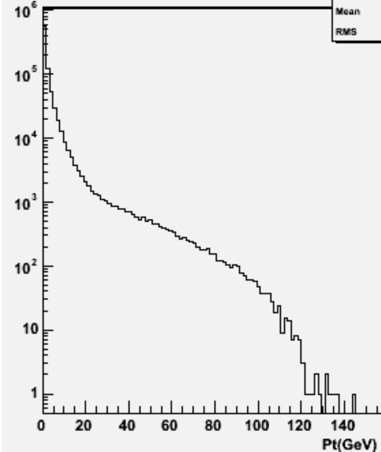
Particle Pt : w101028 ddn2e2du_o
