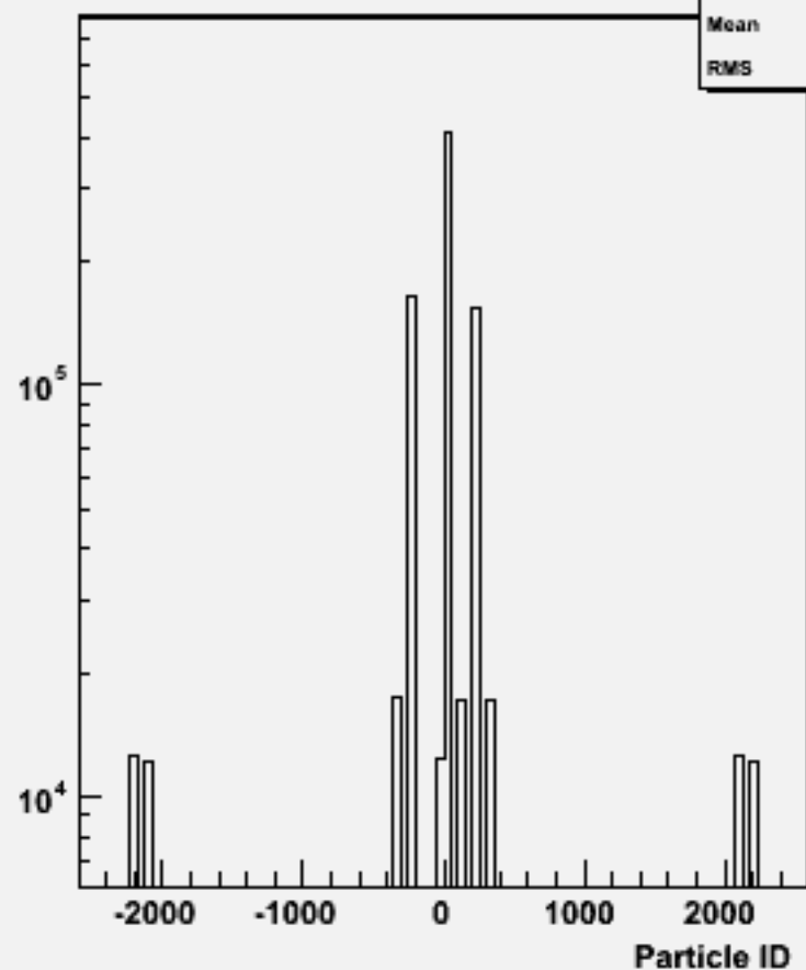
Particle ID : w101028 ddn2e2du_o
