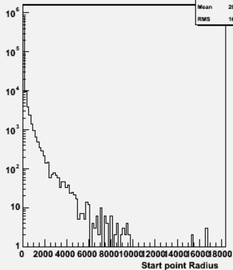
Start point R : w101028 ddn2e2du_o
