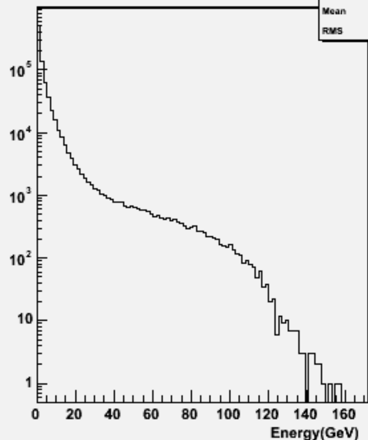
Particle Energy : w101028 ddn2e2du_o
