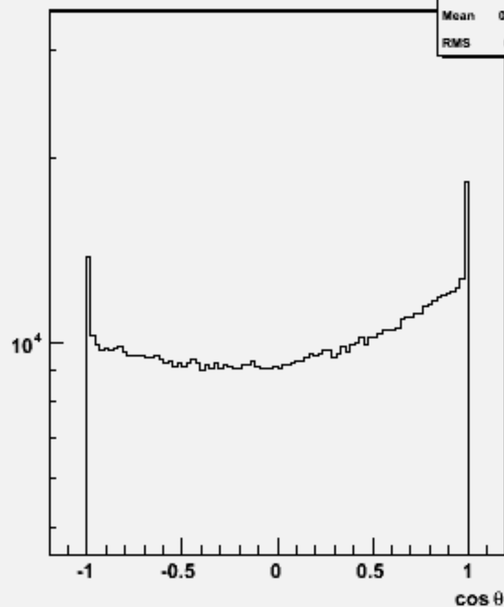
Particle cos \theta : w101028 ddn2e2du_o
