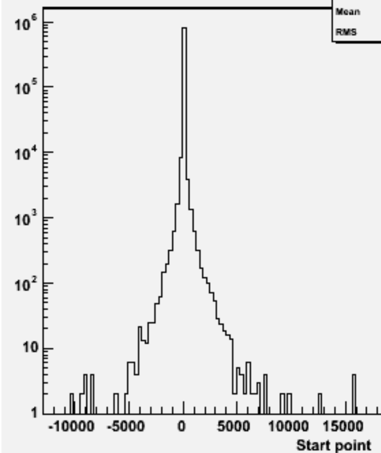
Start point Z : w101028 ddn2e2du_o
