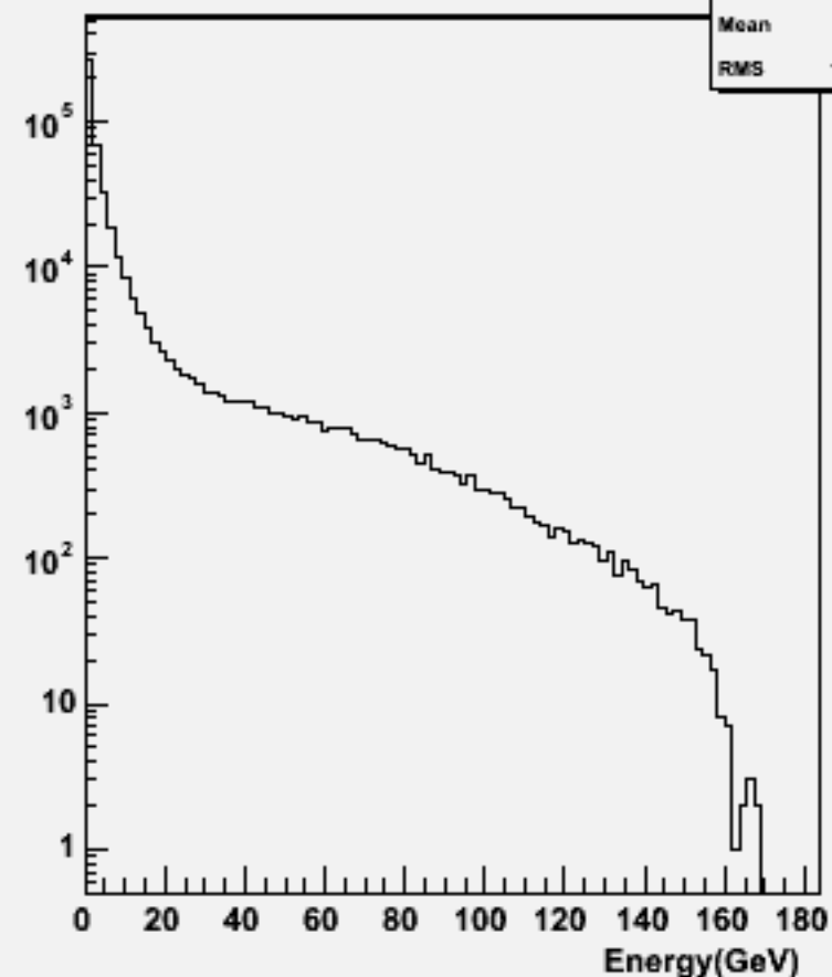
Start point R : w101021 ddn2e2e2n2_o
