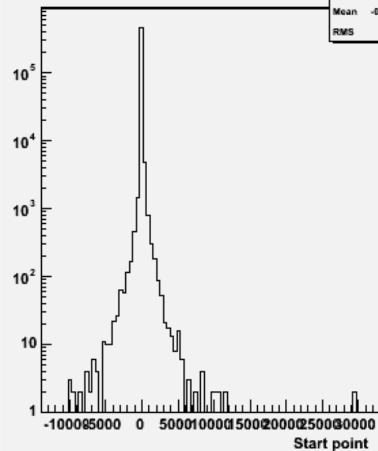
Start point Z : w101021 ddn2e2e2n2_o
