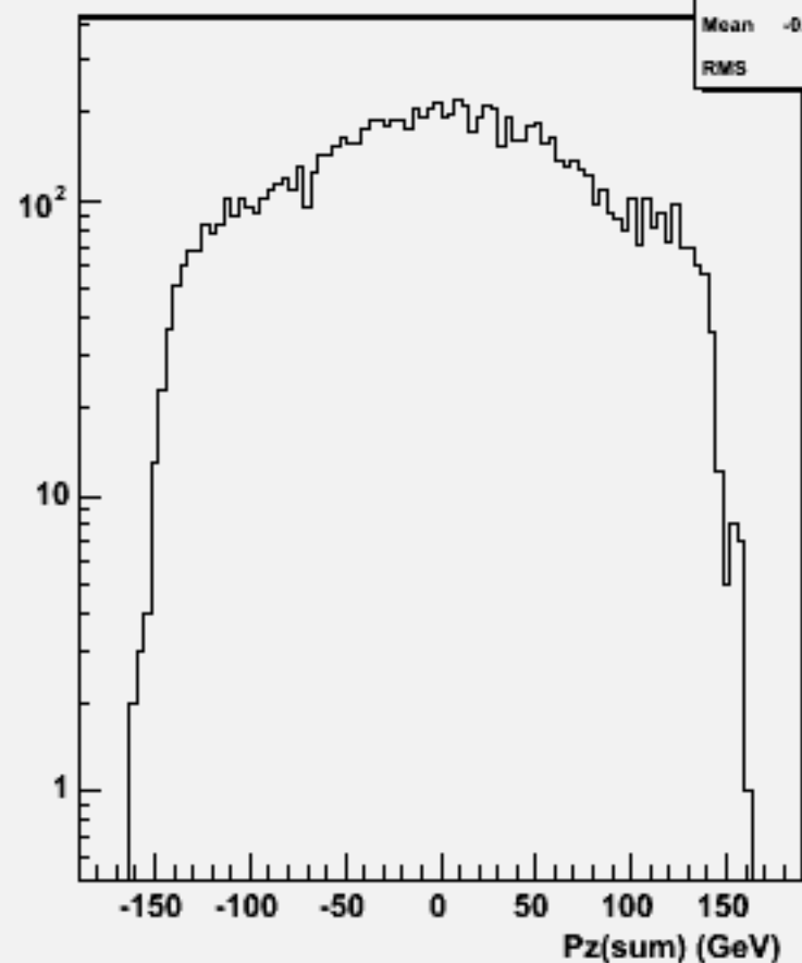
Pz Sum: w101021 ddn2e2e2n2_o
