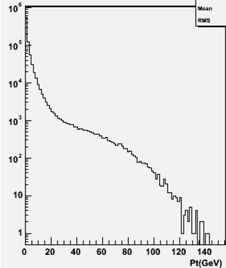
Particle Pt : w101013 ddn1e1sc_o
