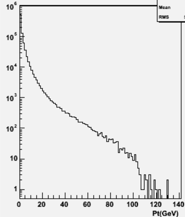
Particle Pt : w101012 ddn1e1sc_o
