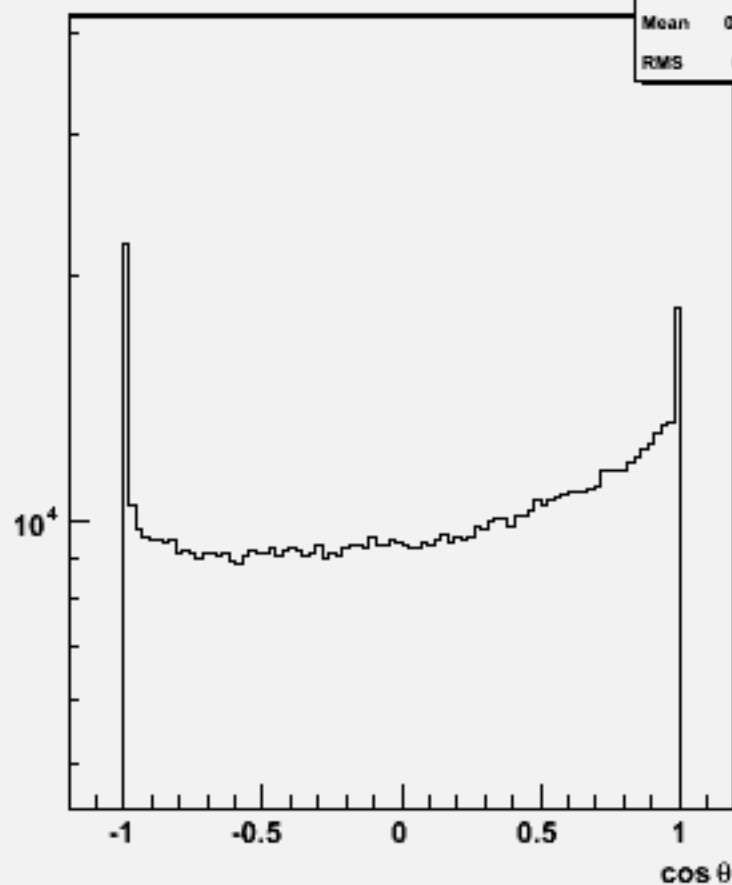
Particle cos \theta : w101012 ddn1e1sc_o
