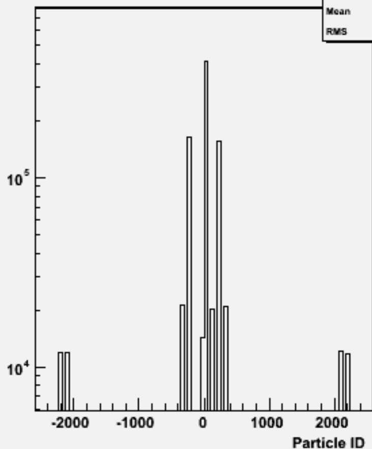
Particle ID : w101012 ddn1e1sc_o
