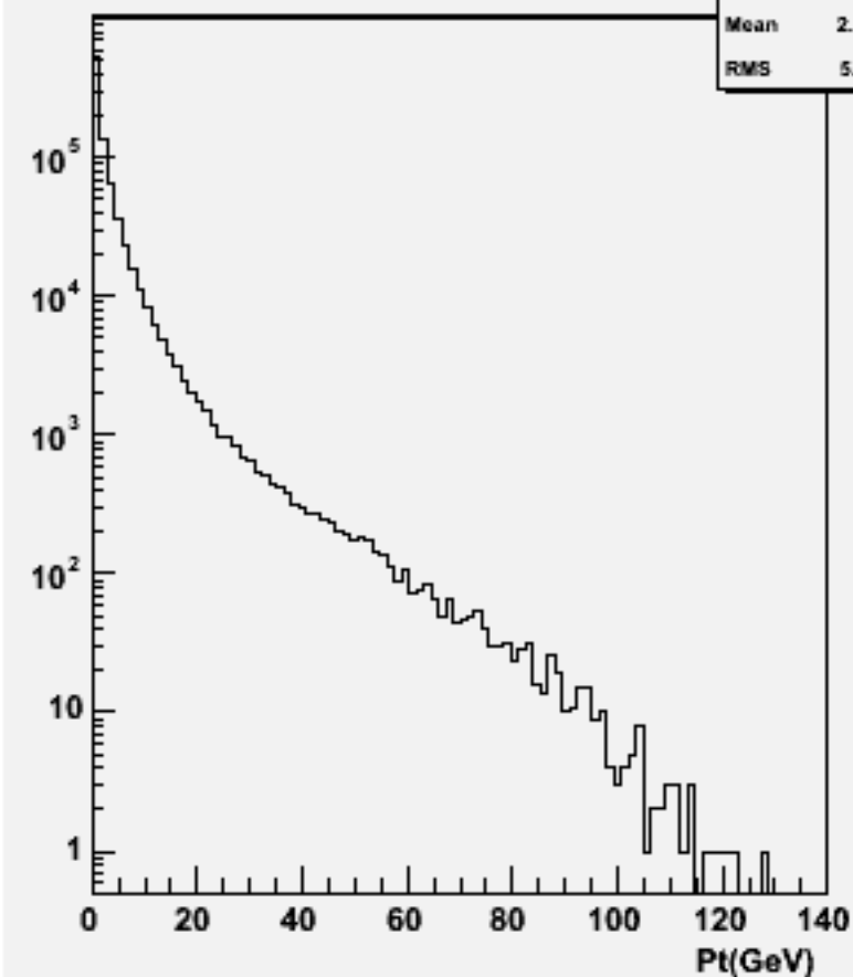
Particle Pt : w101011 ddn1e1sc_o
