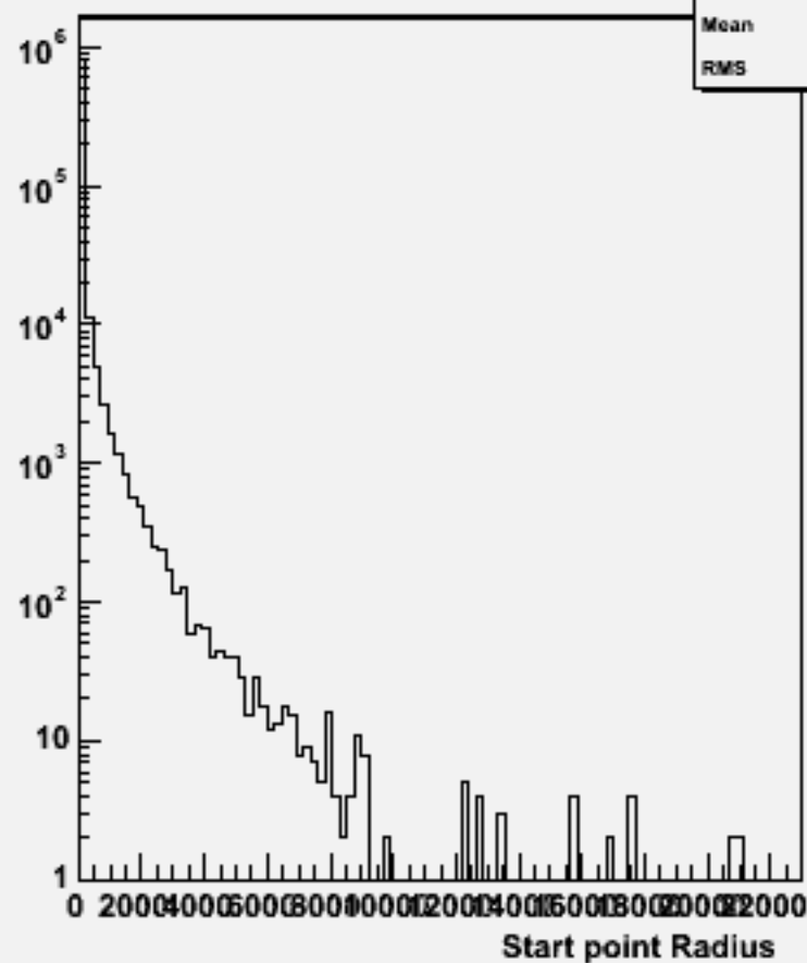
Start point R : w101011 ddn1e1sc_o
