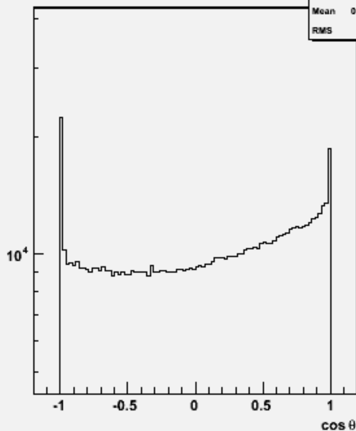
Particle cos \theta : w101011 ddn1e1sc_o
