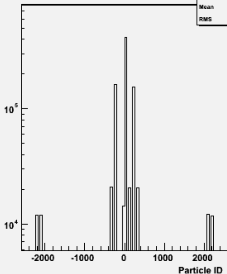
Particle ID : w101011 ddn1e1sc_o
