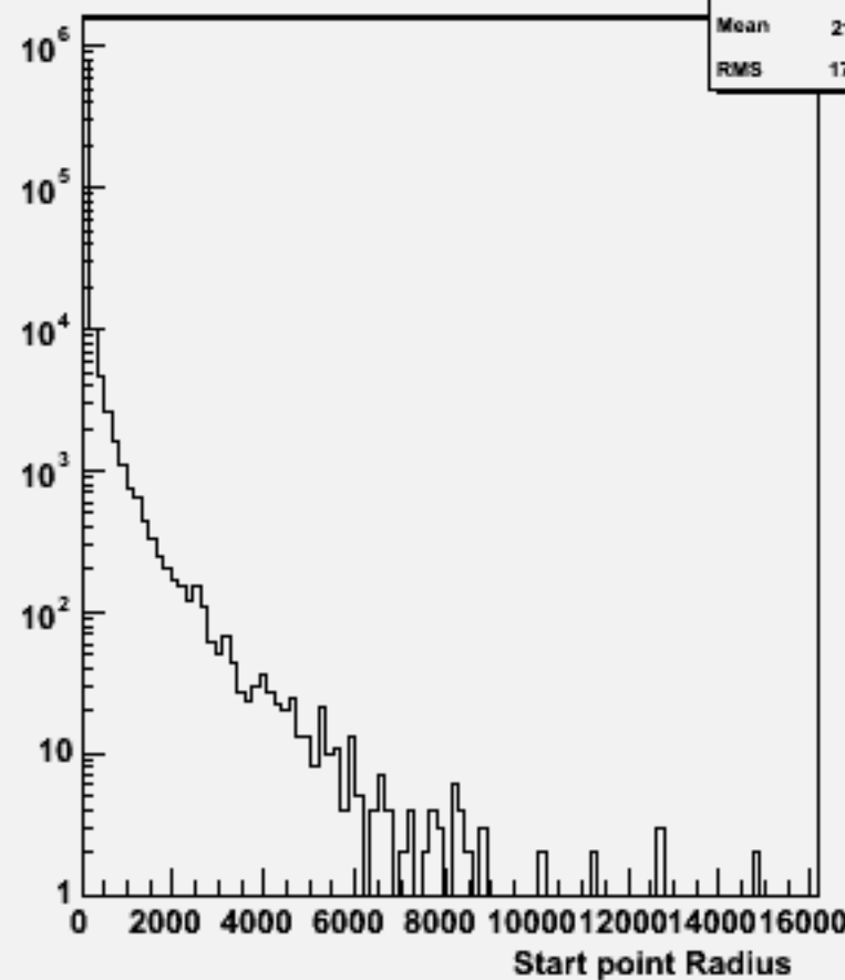
Start point R : w101007 ddn1e1du_o
