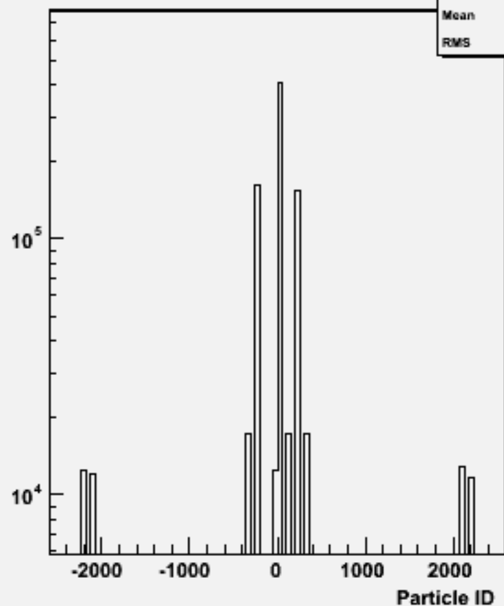
Particle ID : w101007 ddn1e1du_o
