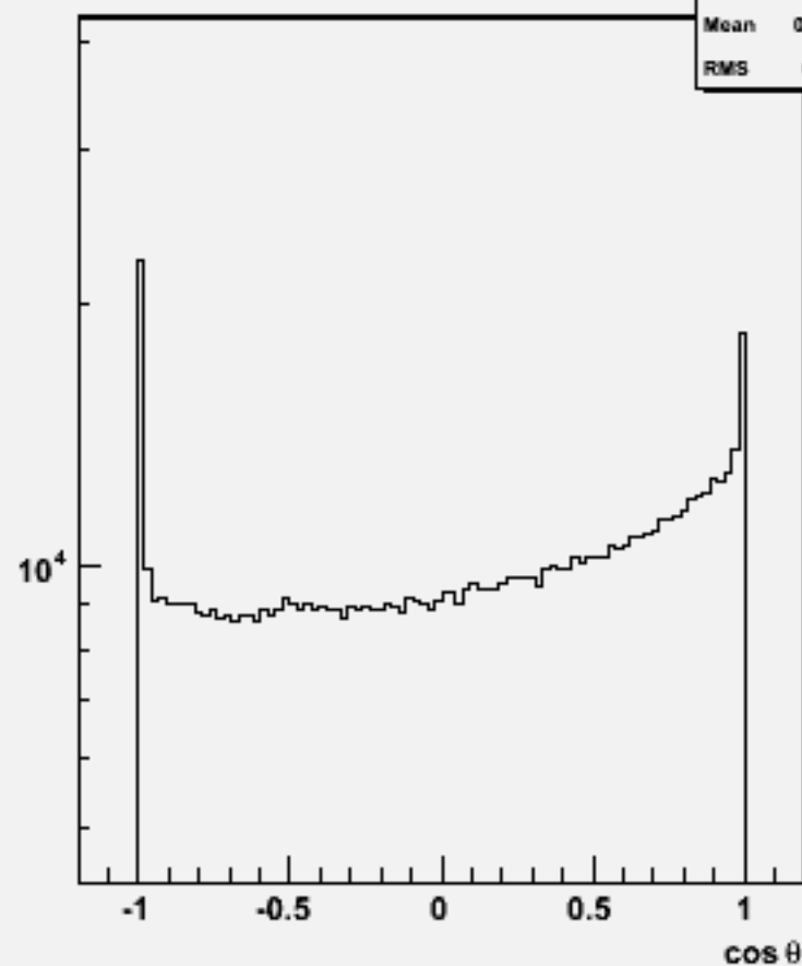
Particle cos \theta : w101007 ddn1e1du_o
