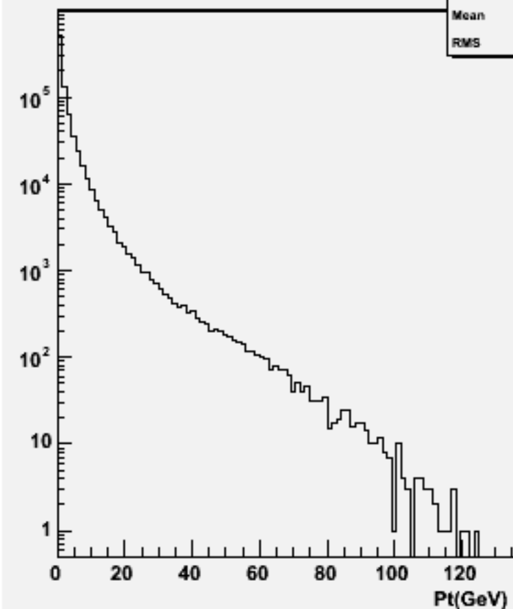
Particle Pt : w101007 ddn1e1du_o
