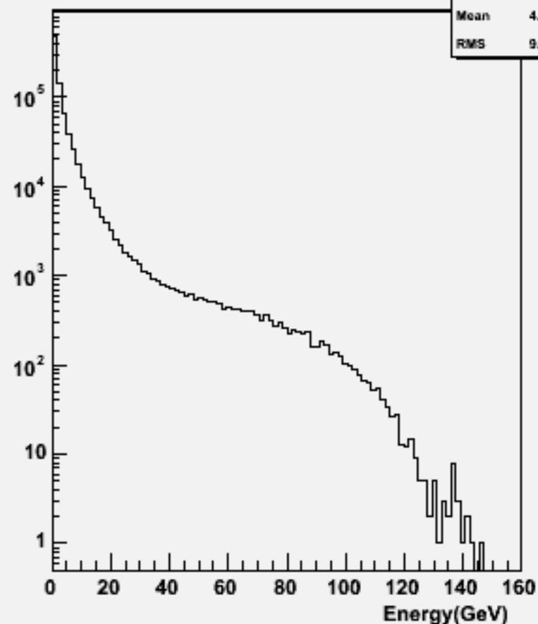
Particle Energy : w101007 ddn1e1du_o
