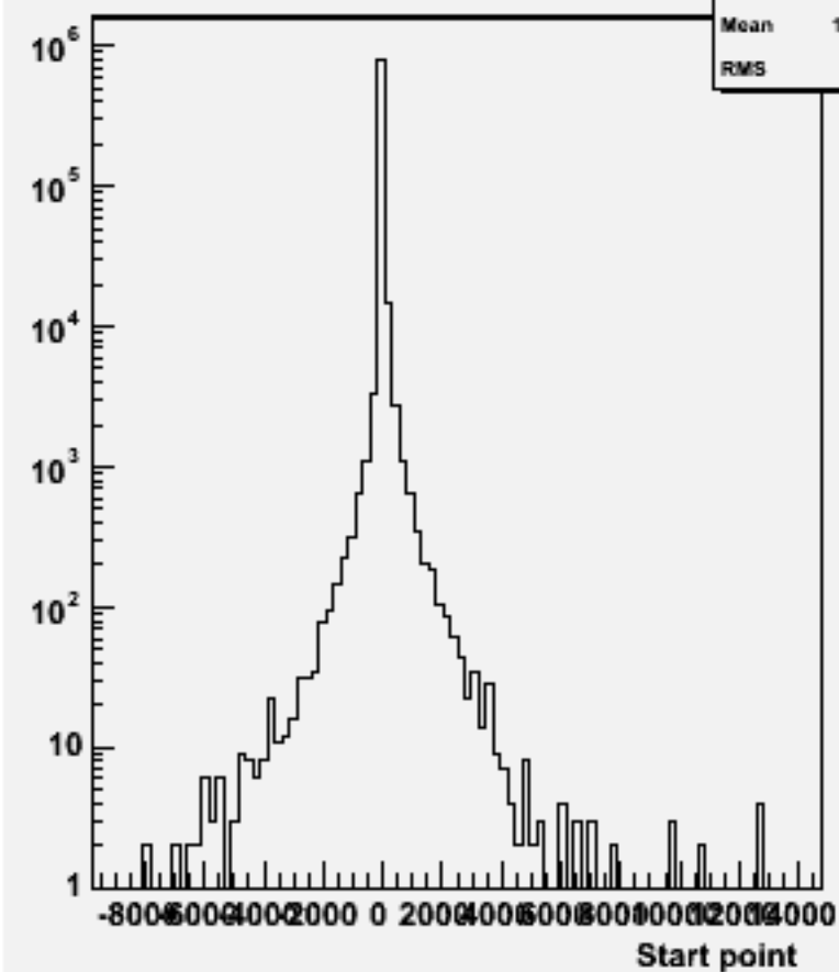
Start point Z : w101007 ddn1e1du_o
