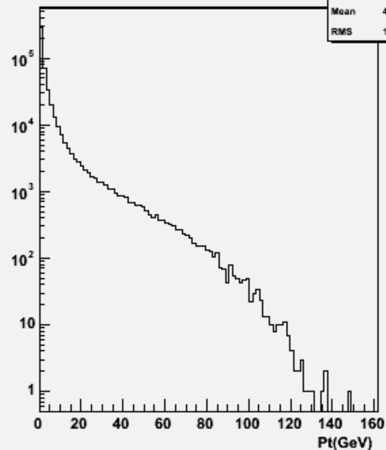
Particle Pt : w101004 ddn1e1e3n3_o
