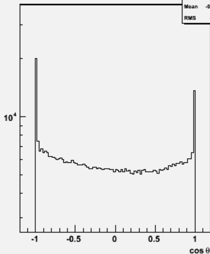
Particle cos \theta : w101004 ddn1e1e3n3_o
