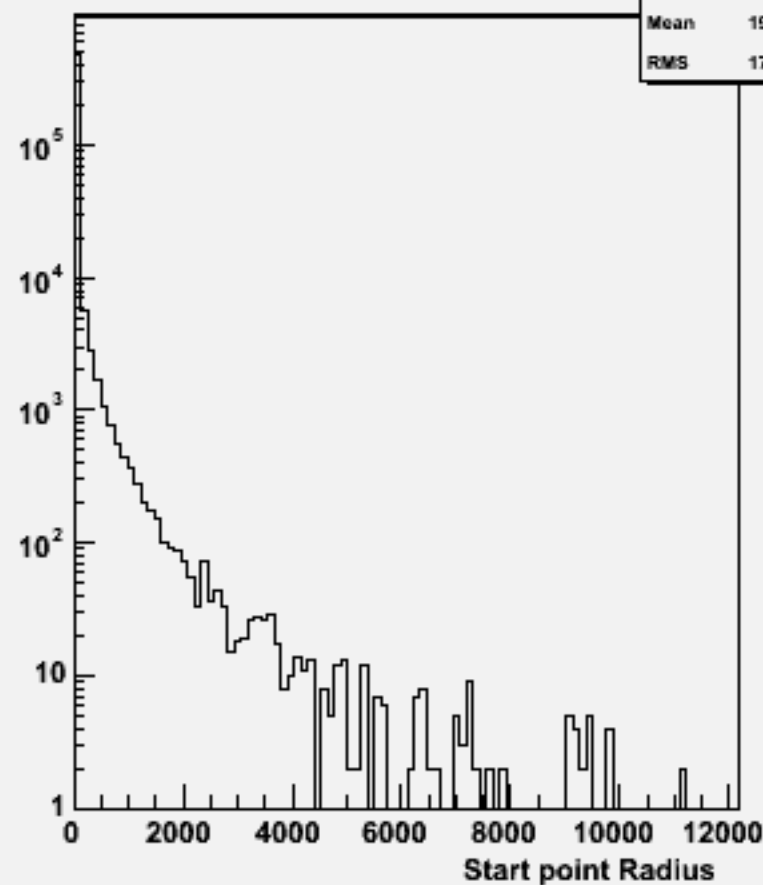
Start point R : w101004 ddn1e1e3n3_o
