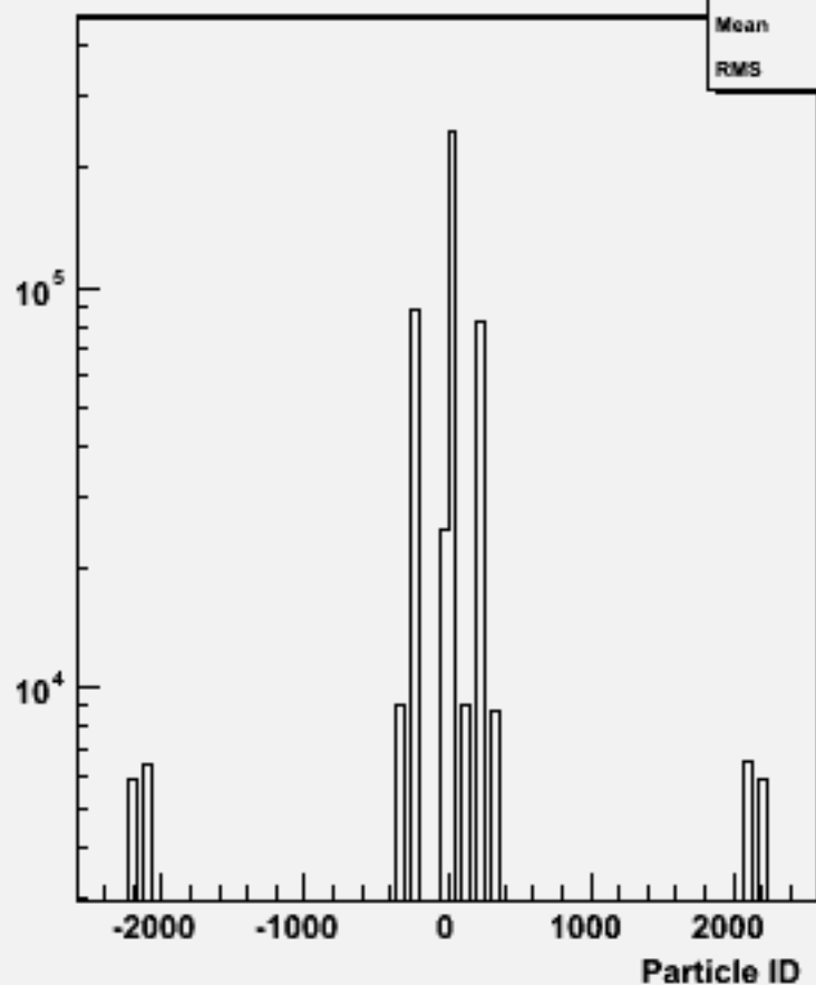
Particle ID : w101004 ddn1e1e3n3_o
