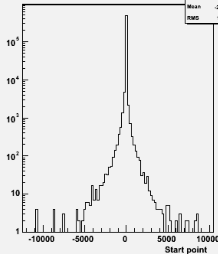
Start point Z : w101004 ddn1e1e3n3_o
