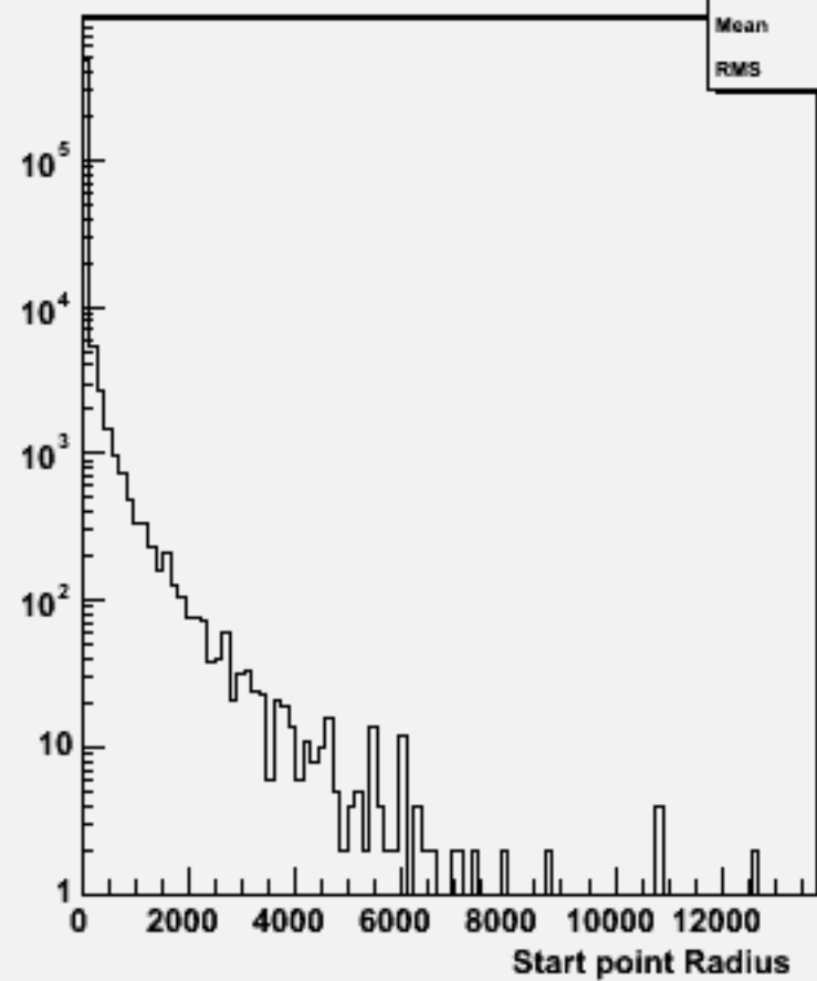
Start point R : w101003 ddn1e1e3n3_o
