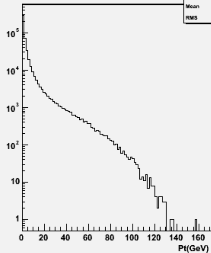
Start point Z : w101003 ddn1e1e3n3_o
