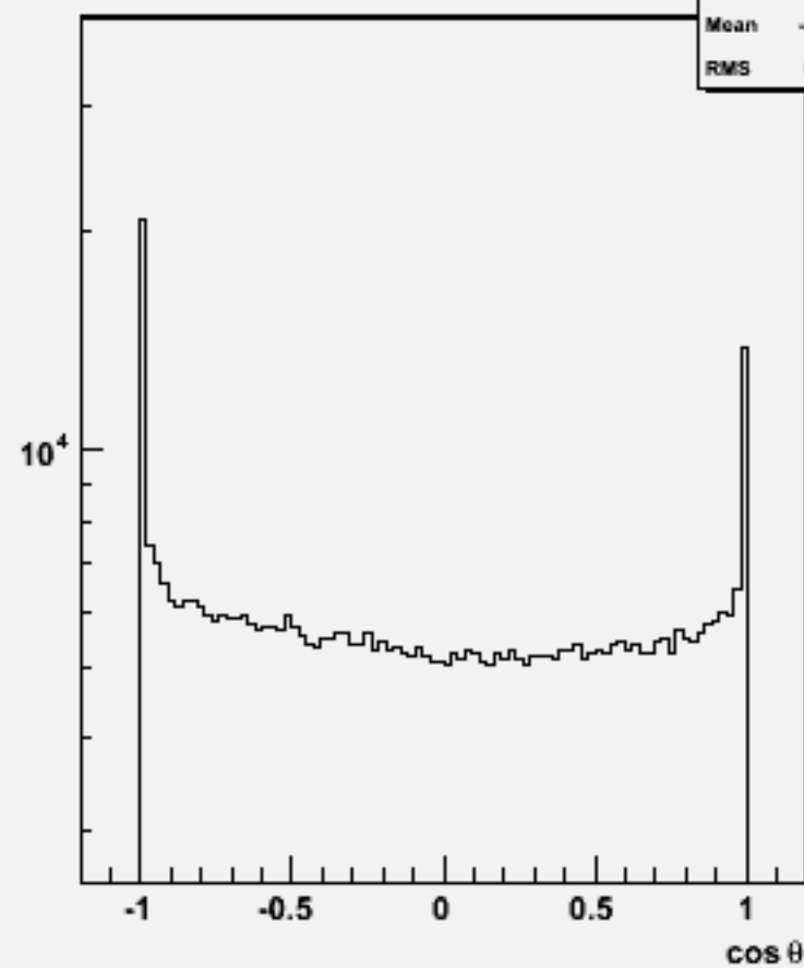
Particle cos θ : w101003 ddn1e1e3n3_o
