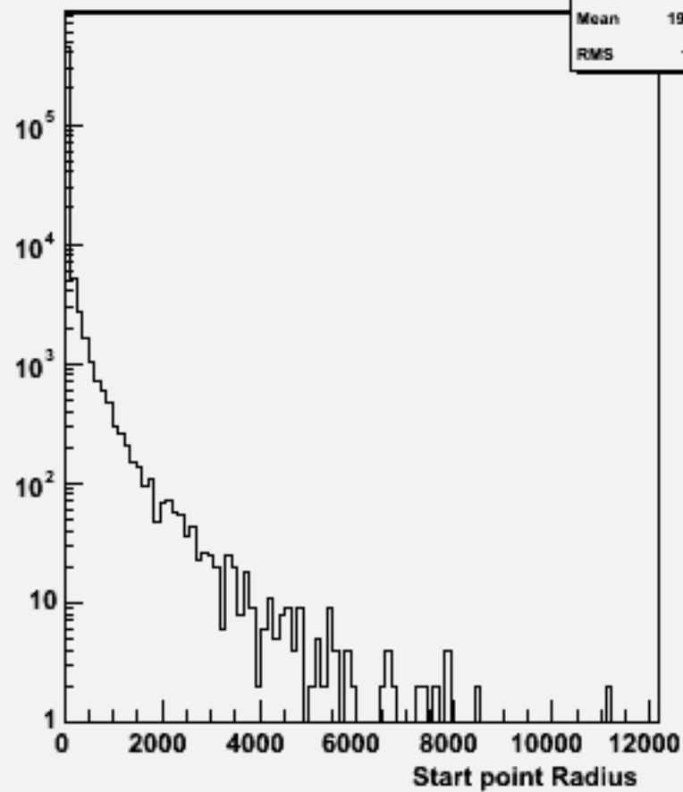
Start point R : w101001 ddn1e1e2n2_o
