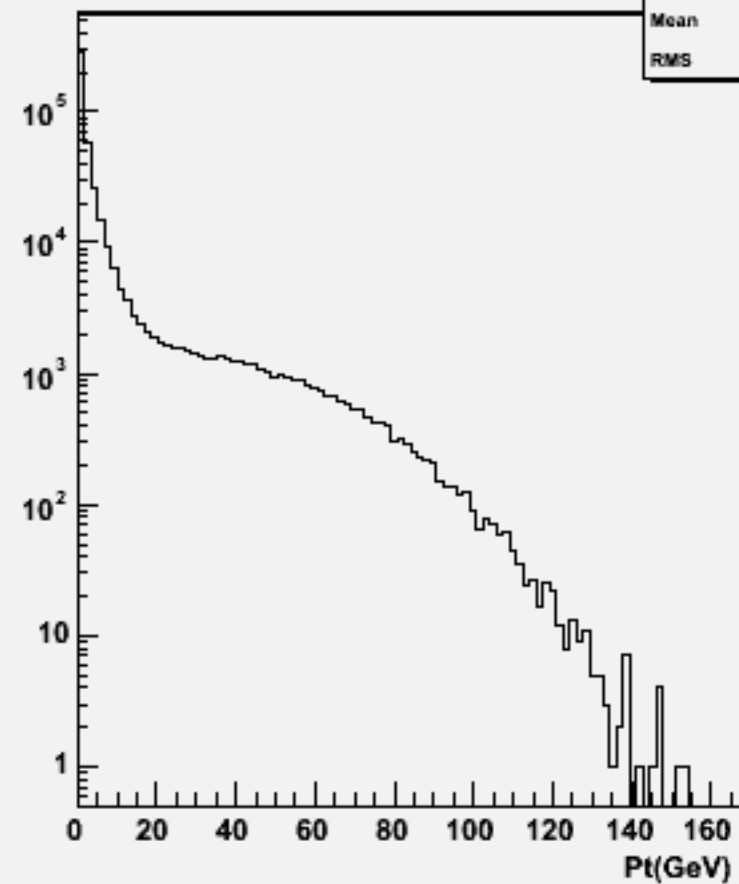
Start point Z : w101001 ddn1e1e2n2_o
