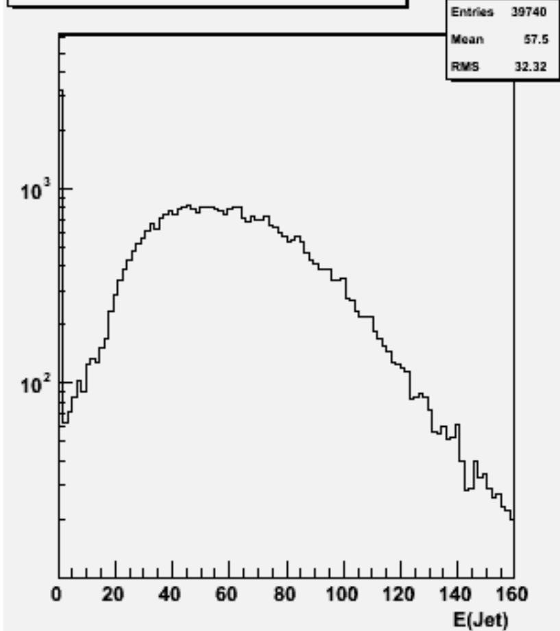
Jet energies(All jets)w101001 ddn1e1e2n2_o
