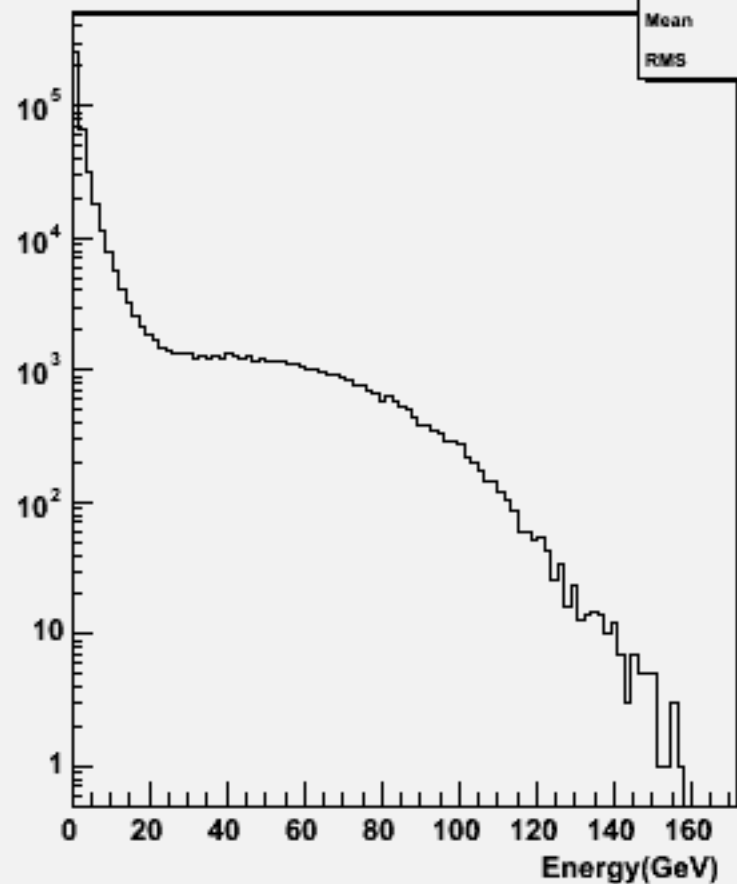
Start point R : w101001 ddn1e1e2n2_o
