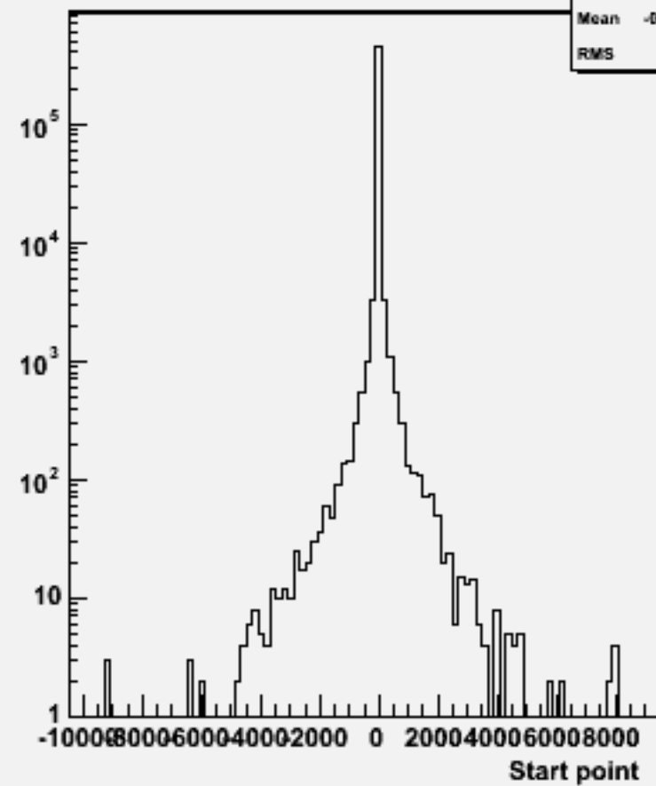
Start point Z : w101001 ddn1e1e2n2_o
