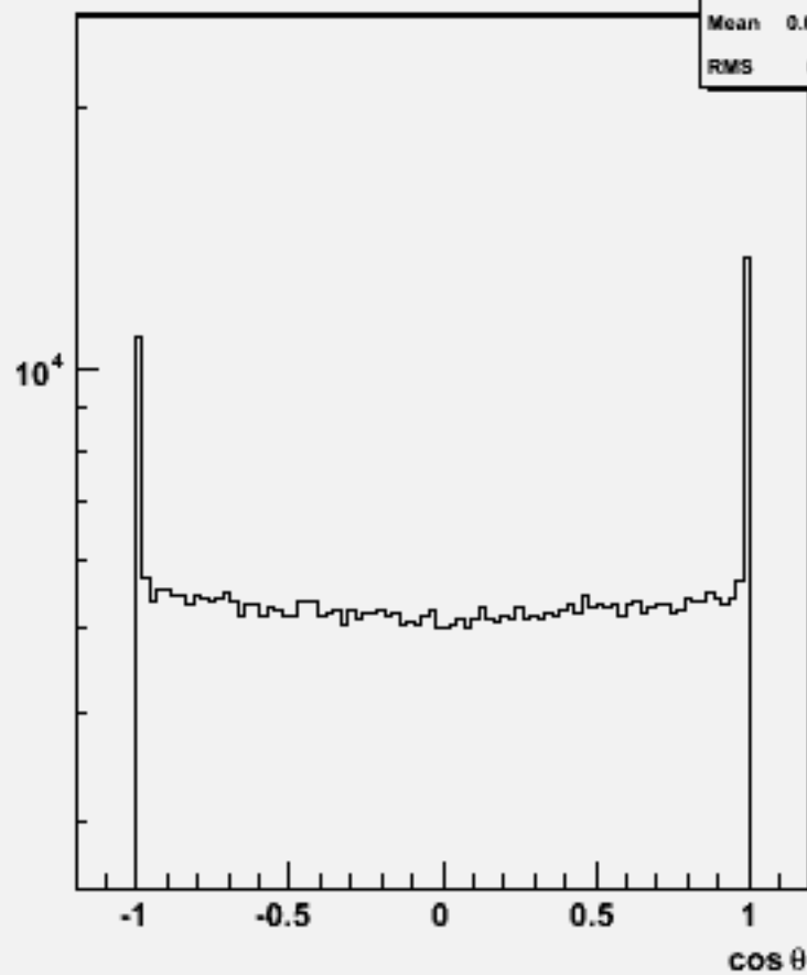
Particle \cos\theta : w101001 ddn1e1e2n2_o
