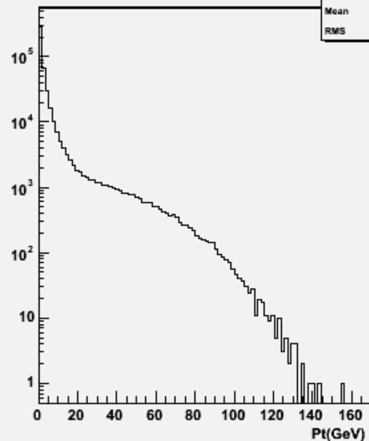
Start point Z : w100999 ddn1e1e2n2_o
