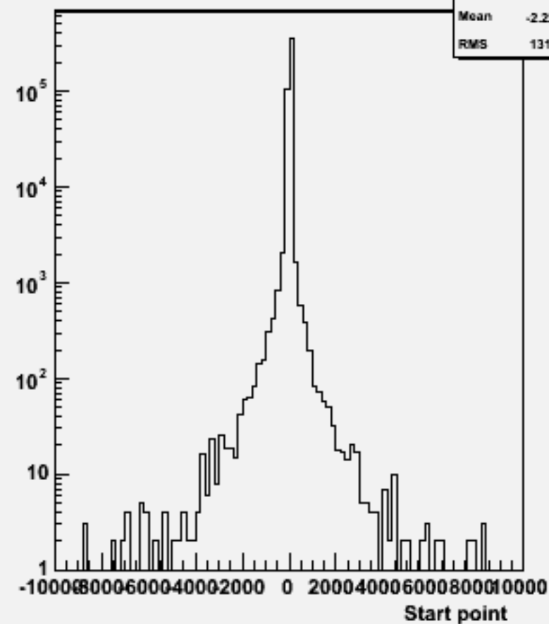
Start point Z : w100999 ddn1e1e2n2_o
