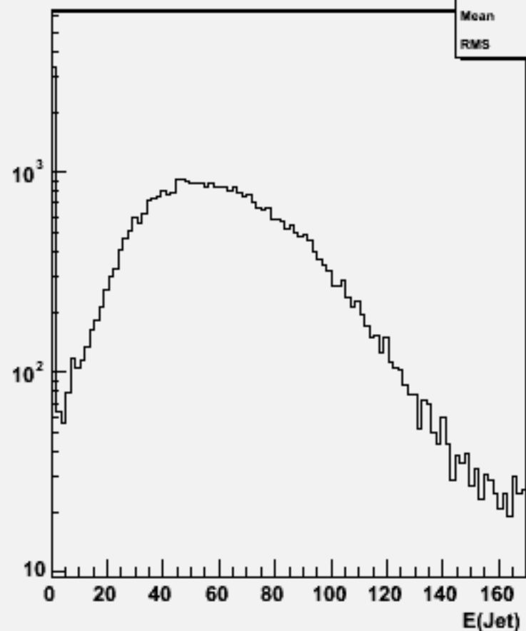
Jet energies(All jets)w100999 ddn1e1e2n2_o
