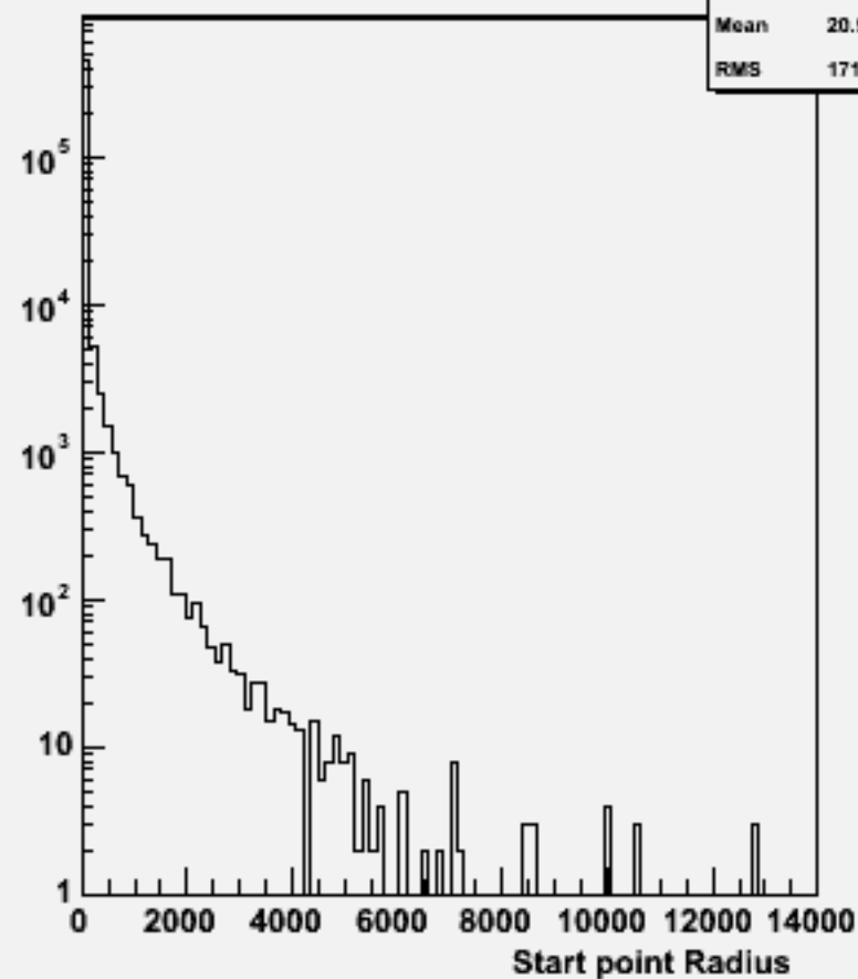
Start point R : w100999 ddn1e1e2n2_o
