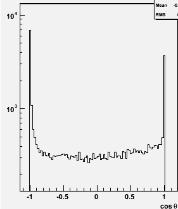
Jet cos \theta (All jets)w100999 ddn1e1e2n2_o
