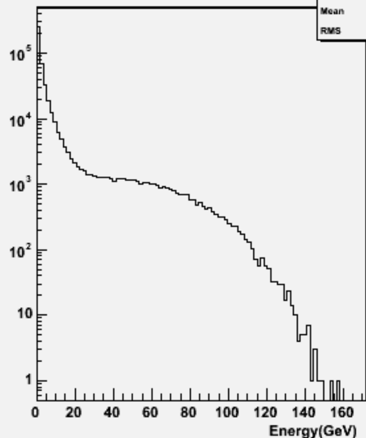
Start point R : w100999 ddn1e1e2n2_o
