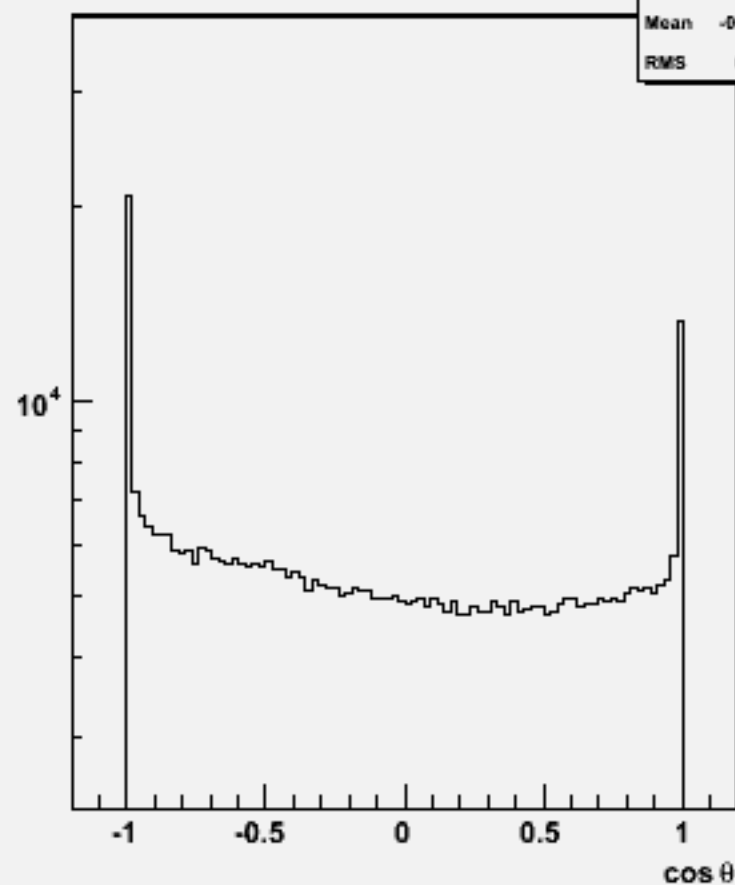
Particle cos \theta : w100999 ddn1e1e2n2_o
